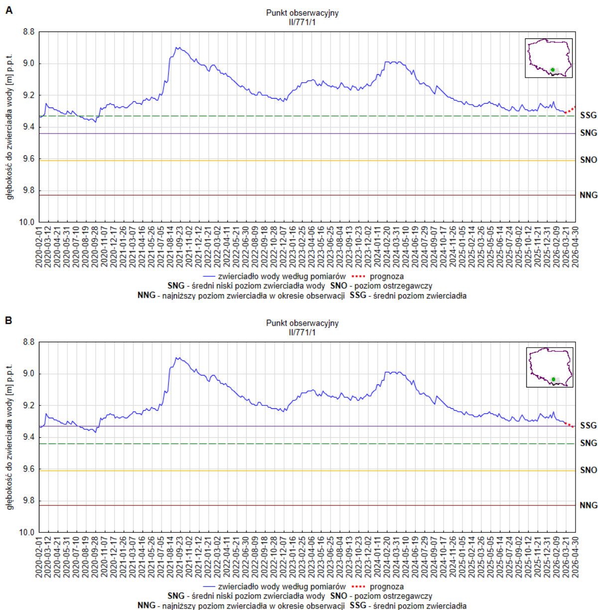
Rys. 10. Prognoza dotycząca stanu wód o zwierciadle swobodnym (gruntowych) na okres 01.04.2026 – 30.04.2026 r. – stacja hydrogeologiczna nr II/771/1 w miejscowości Kraków (woj. małopolskie). A – prognoza przy założeniu scenariusza A; B – prognoza przy założeniu scenariusza B
