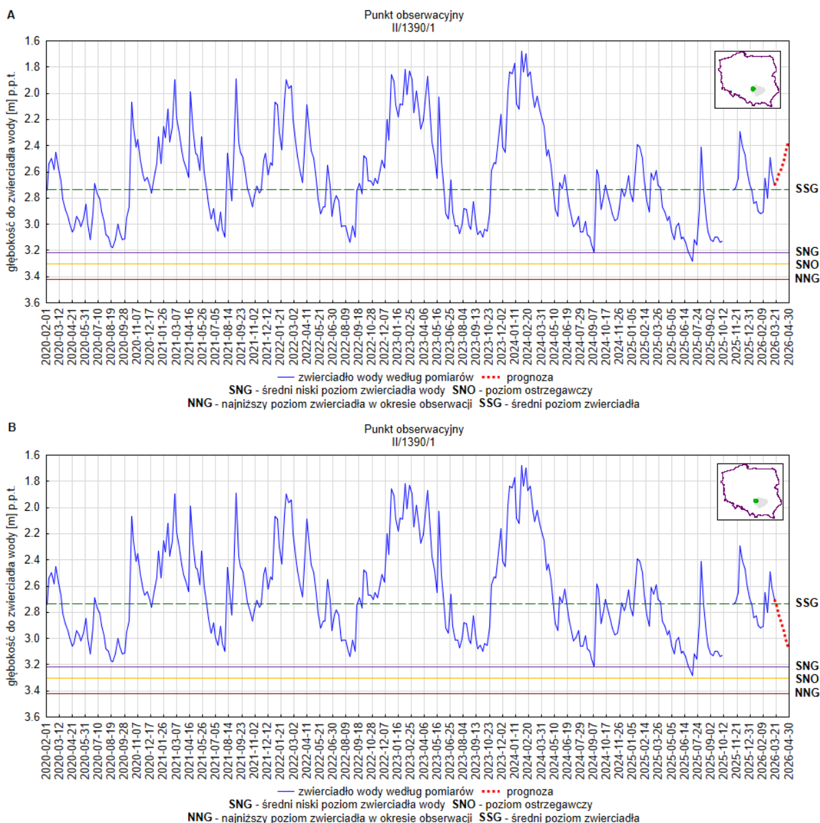
Rys. 21. Prognoza dotycząca stanu wód o zwierciadle swobodnym (gruntowych) na okres 01.04.2026 – 30.04.2026 r. – stacja hydrogeologiczna nr II/1390/1 w miejscowości Januszewice (woj. świętokrzyskie). A – prognoza przy założeniu scenariusza A; B – prognoza przy założeniu scenariusza B
