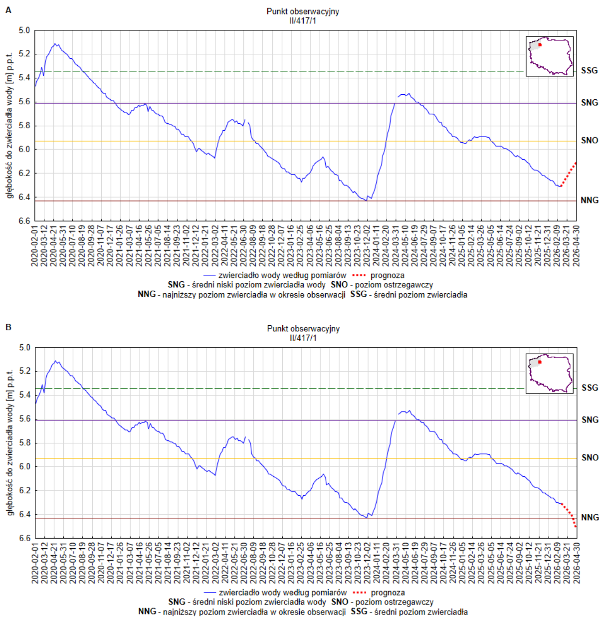
Rys. 25. Prognoza dotycząca stanu wód o zwierciadle swobodnym (gruntowych) na okres 01.04.2026 – 30.04.2026 r. – stacja hydrogeologiczna nr II/417/1 w miejscowości Turowo (woj. zachodniopomorskie). A – prognoza przy założeniu scenariusza A; B – prognoza przy założeniu scenariusza B
