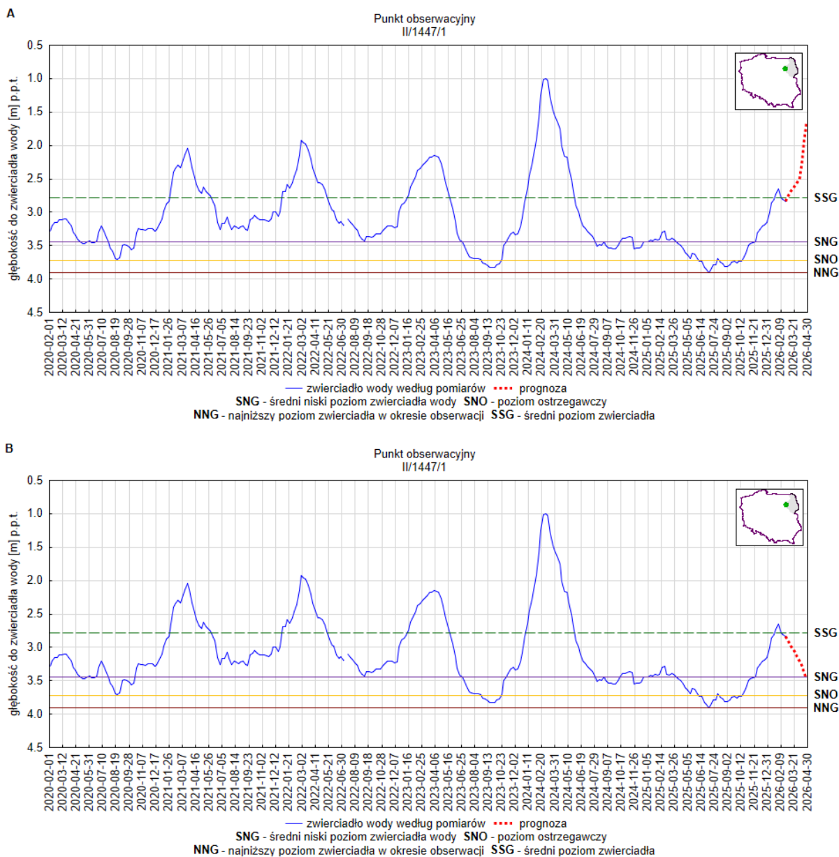
Rys. 16. Prognoza dotycząca stanu wód o zwierciadle swobodnym (gruntowych) na okres 01.04.2026 – 30.04.2026 r.- stacja hydrogeologiczna nr II/1447/1 w miejscowości Morgowniki (woj. podlaskie). A – prognoza przy założeniu scenariusza A; B – prognoza przy założeniu scenariusza B
