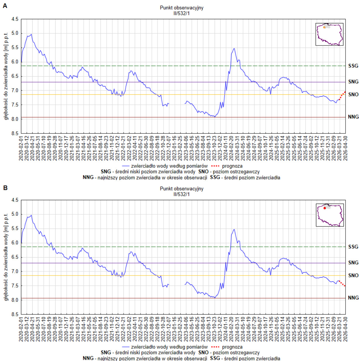
Rys. 17. Prognoza dotycząca stanu wód o zwierciadle swobodnym (gruntowych) na okres 01.04.2026 -30.04.2026 r. – stacja hydrogeologiczna nr II/532/1 w miejscowości Rzeczenica (woj. pomorskie). A – prognoza przy założeniu scenariusza A; B – prognoza przy założeniu scenariusza B
