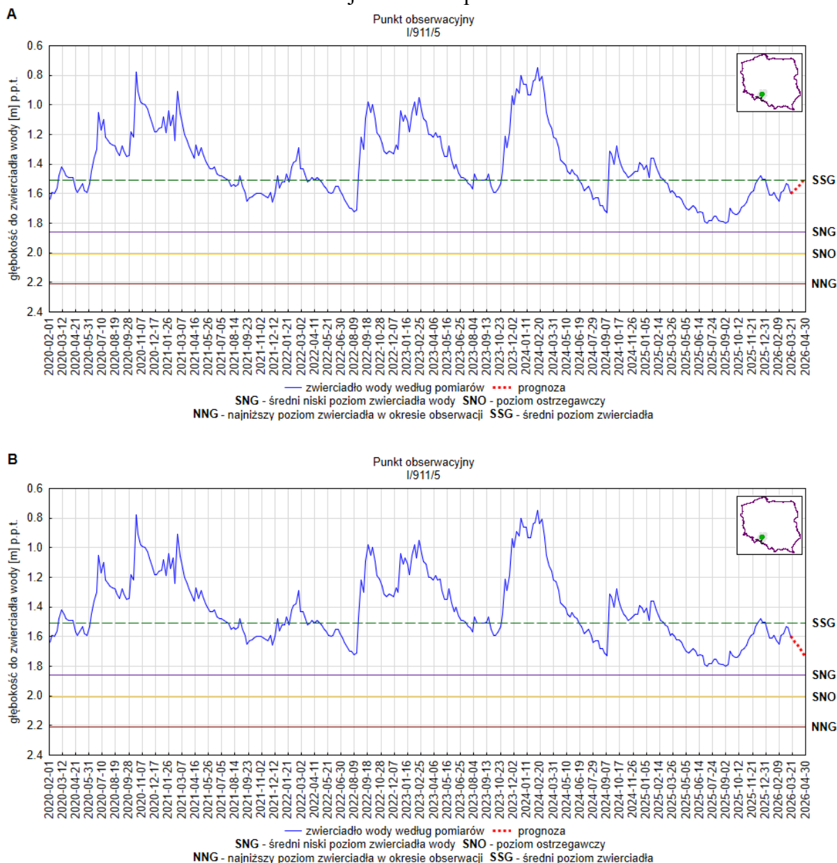
Rys. 13. Prognoza dotycząca stanu wód o zwierciadle swobodnym (gruntowych) na okres 01.04.2026 – 30.04.2026 r. – stacja hydrogeologiczna nr I/911/5 w miejscowości Wrzoski (woj. opolskie). A – prognoza przy założeniu scenariusza A; B – prognoza przy założeniu scenariusza B
