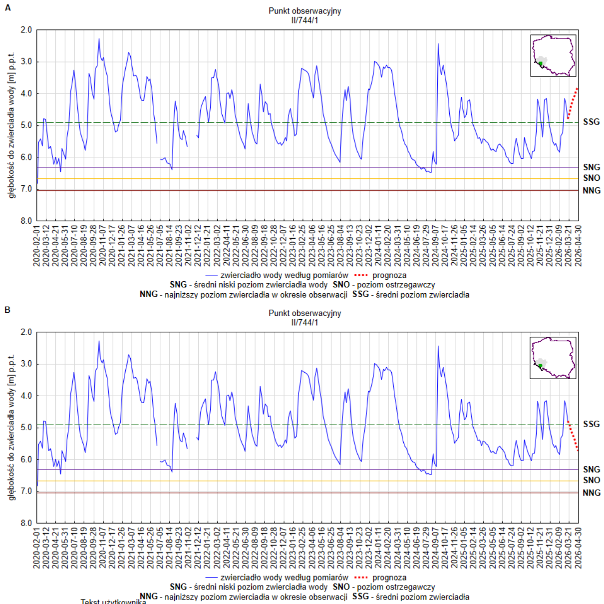
Rys. 2. Prognoza dotycząca stanu wód o zwierciadle swobodnym (gruntowych) na okres 01.04.2026 – 30.04.2026 r. – stacja hydrogeologiczna nr II/744/1 w miejscowości Szczawno Zdrój (woj. dolnośląskie). A – prognoza przy założeniu scenariusza A; B – prognoza przy założeniu scenariusza B
