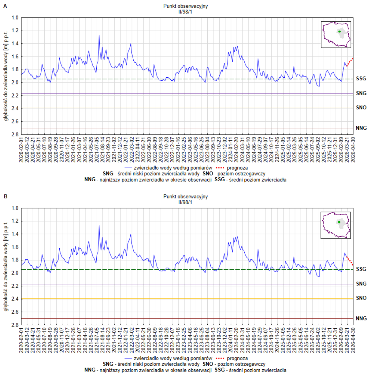
Rys. 12. Prognoza dotycząca stanu wód o zwierciadle swobodnym (gruntowych) na okres 01.04.2026 – 30.04.2026 r. – stacja hydrogeologiczna nr II/98/1 w miejscowości Płońsk (woj. mazowieckie). A – prognoza przy założeniu scenariusza A; B – prognoza przy założeniu scenariusza B
