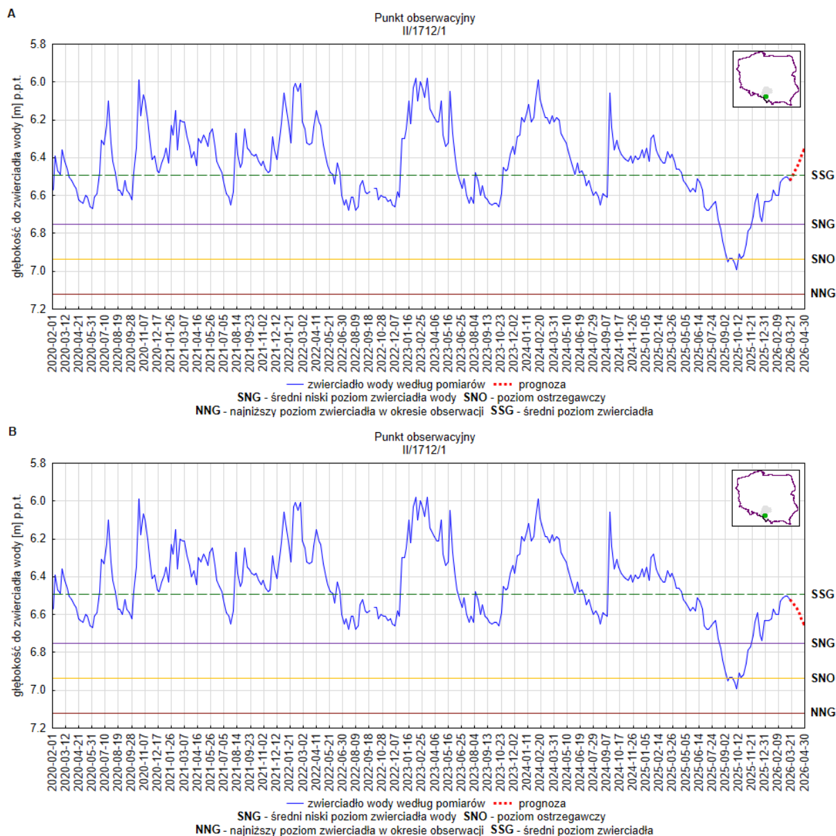
Rys. 19 Prognoza dotycząca stanu wód o zwierciadle swobodnym (gruntowych) na okres 01.04.2026 – 30.04.2026 r. – stacja hydrogeologiczna nr II/1712/1 w miejscowości Piasek (woj. śląskie). A – prognoza przy założeniu scenariusza A; B – prognoza przy założeniu scenariusza B
