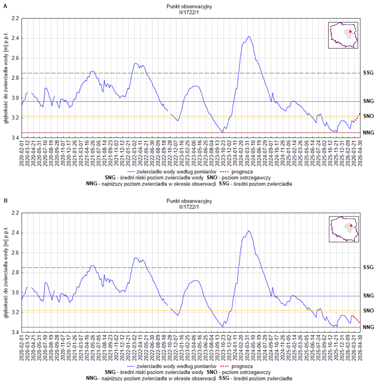
Rys. 11. Prognoza dotycząca stanu wód o zwierciadle swobodnym (gruntowych) na okres 01.04.2026 – 30.04.2026 r. – stacja hydrogeologiczna nr II/1722/1 w miejscowości Nagoszewo (woj. mazowieckie). A – prognoza przy założeniu scenariusza A; B – prognoza przy założeniu scenariusza B
