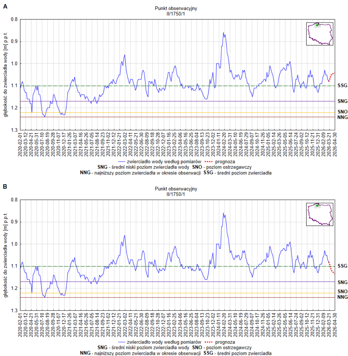
Rys. 18. Prognoza dotycząca stanu wód o zwierciadle swobodnym (gruntowych) na okres 01.04.2026 -30.04.2026 r. – stacja hydrogeologiczna nr II/1750/1 w miejscowości Borucino (woj. pomorskie). A – prognoza przy założeniu scenariusza A; B – prognoza przy założeniu scenariusza B
