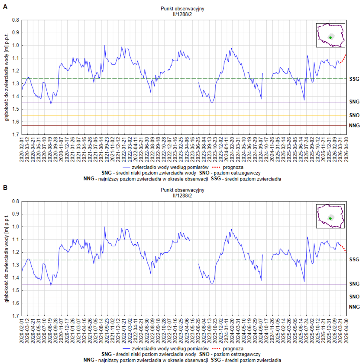
Rys. 9. Prognoza dotycząca stanu wód o zwierciadle swobodnym (gruntowych) na okres 01.04.2026 – 30.04.2026 r. – stacja hydrogeologiczna nr II/1288/2 w miejscowości Marcelów (woj. łódzkie). A – prognoza przy założeniu scenariusza A; B – prognoza przy założeniu scenariusza B
