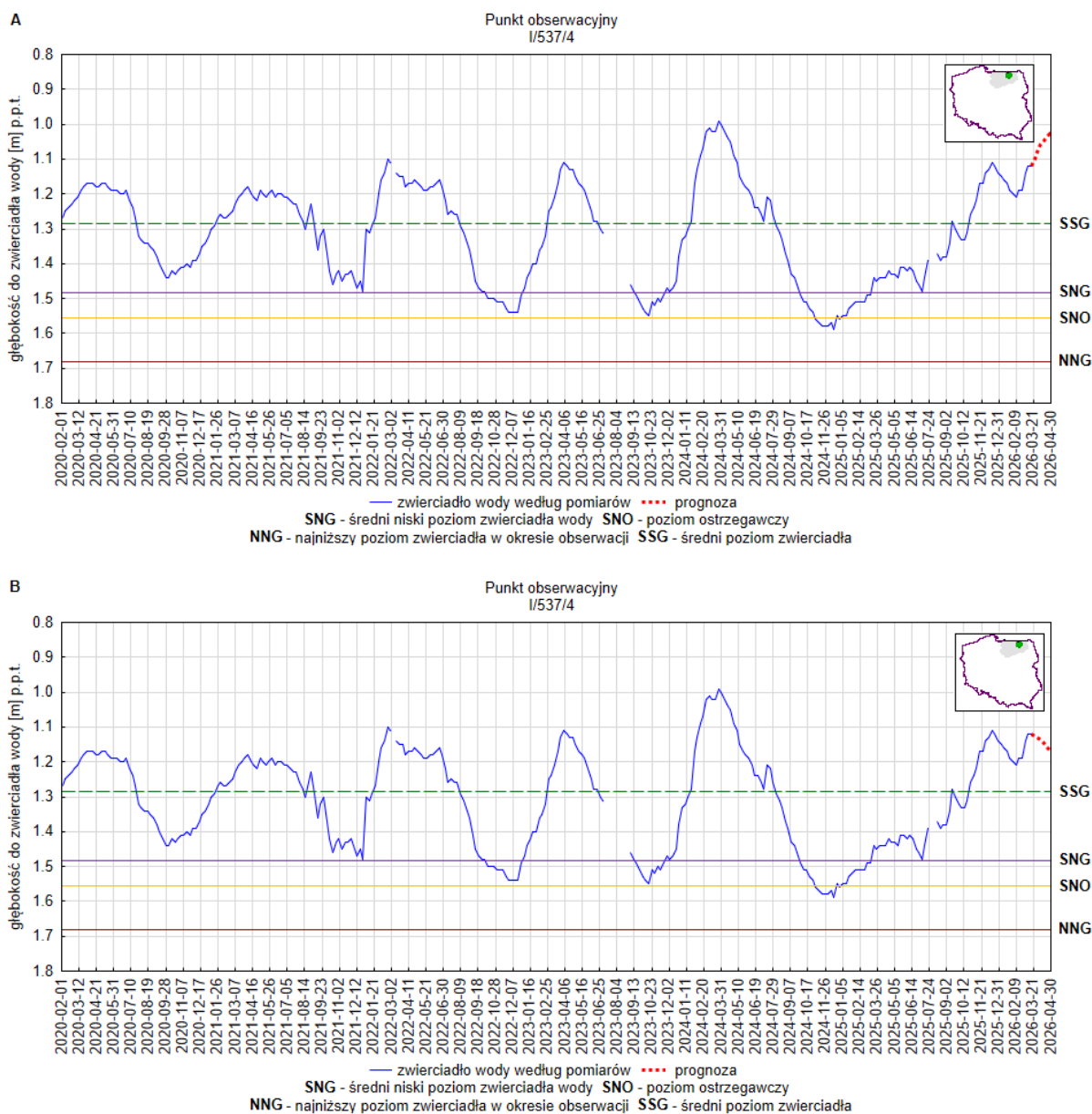
Rys. 23. Prognoza dotycząca stanu wód o zwierciadle swobodnym (gruntowych) na okres 01.04.2026 – 30.04.2026 r. – stacja hydrogeologiczna nr I/537/4 w miejscowości Doba (woj. warmińsko-mazurskie). A – prognoza przy założeniu scenariusza A; B – prognoza przy założeniu scenariusza B
