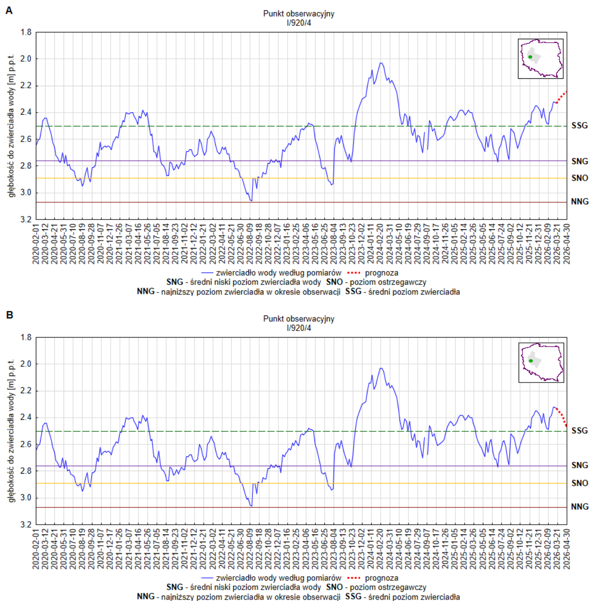
Rys. 24. Prognoza dotycząca stanu wód o zwierciadle swobodnym (gruntowych) na okres 01.04.2026 – 30.04.2026 r. – stacja hydrogeologiczna nr I/920/4 w miejscowości Sepno (woj. wielkopolskie). A – prognoza przy założeniu scenariusza A; B – prognoza przy założeniu scenariusza B
