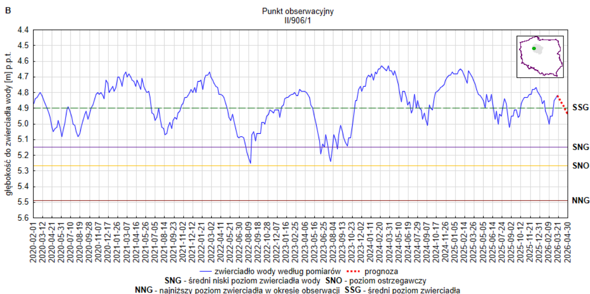
Rys. 4. Prognoza dotycząca stanu wód o zwierciadle swobodnym (gruntowych) na okres 01.04.2026 – 30.04.2026 r. – stacja hydrogeologiczna nr II/906/1 w miejscowości Rozwarzyn (woj. kujawsko-pomorskie). A – prognoza przy założeniu scenariusza A; B – prognoza przy założeniu scenariusza B
