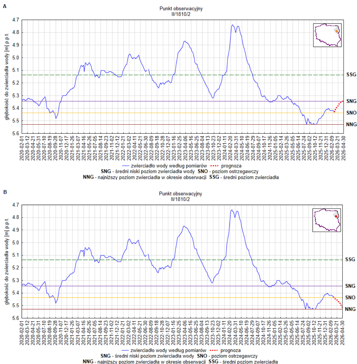
Rys. 15. Prognoza dotycząca stanu wód o zwierciadle swobodnym (gruntowych) na okres 01.04.2026 – 30.04.2026 r.- stacja hydrogeologiczna nr II/1810/2 w miejscowości Liza Stara (woj. podlaskie). A – prognoza przy założeniu scenariusza A; B – prognoza przy założeniu scenariusza B
