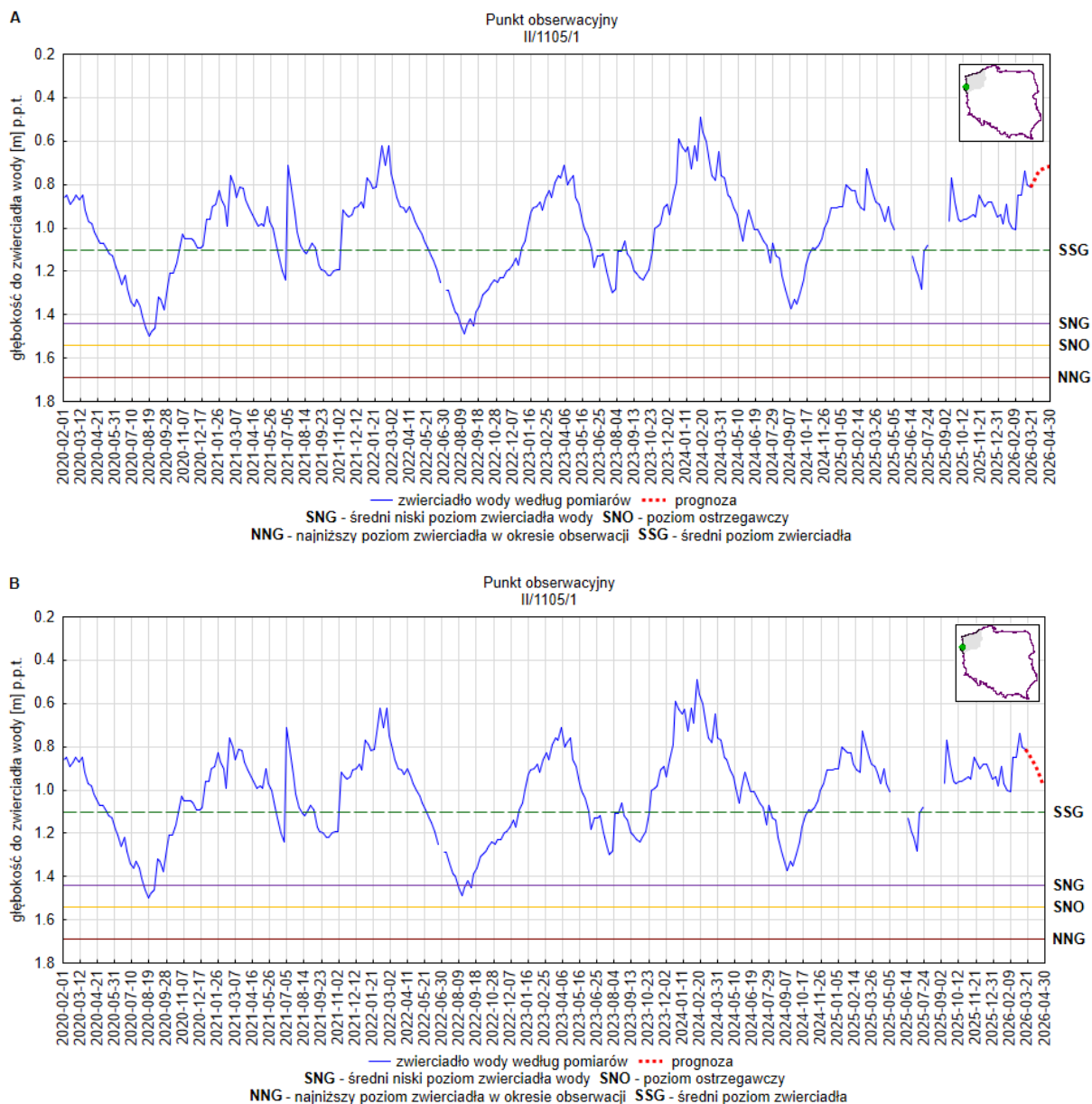
Rys. 26. Prognoza dotycząca stanu wód o zwierciadle swobodnym (gruntowych) na okres 01.04.2026 – 30.04.2026 r. – stacja hydrogeologiczna nr II/1105/1 w miejscowości Ognica (woj. zachodniopomorskie). A – prognoza przy założeniu scenariusza A; B – prognoza przy założeniu scenariusza B
