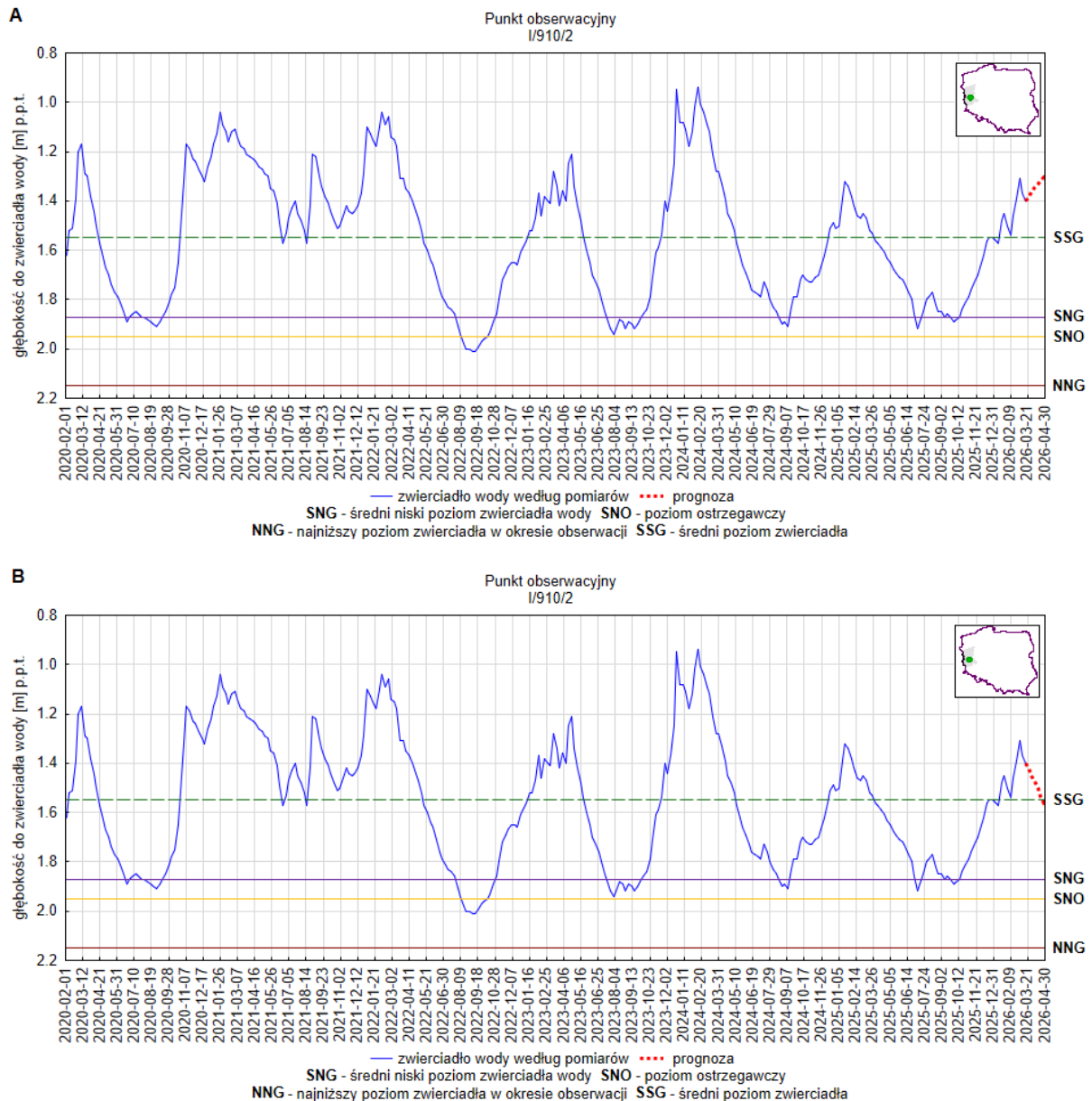
Rys. 7. Prognoza dotycząca stanu wód o zwierciadle swobodnym (gruntowych) na okres 01.04.2026 – 30.04.2026 r. – stacja hydrogeologiczna nr I/910/2 w miejscowości Wysokie (woj. lubuskie) A – prognoza przy założeniu scenariusza A; B – prognoza przy założeniu scenariusza B
