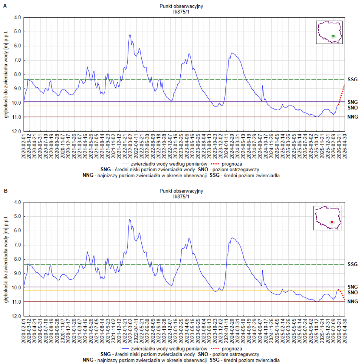
Rys. 20. Prognoza dotycząca stanu wód o zwierciadle swobodnym (gruntowych) na okres 01.04.2026 – 30.04.2026 r. – stacja hydrogeologiczna nr II/875/1 w miejscowości Ściegna (woj. świętokrzyskie). A – prognoza przy założeniu scenariusza A; B – prognoza przy założeniu scenariusza B
