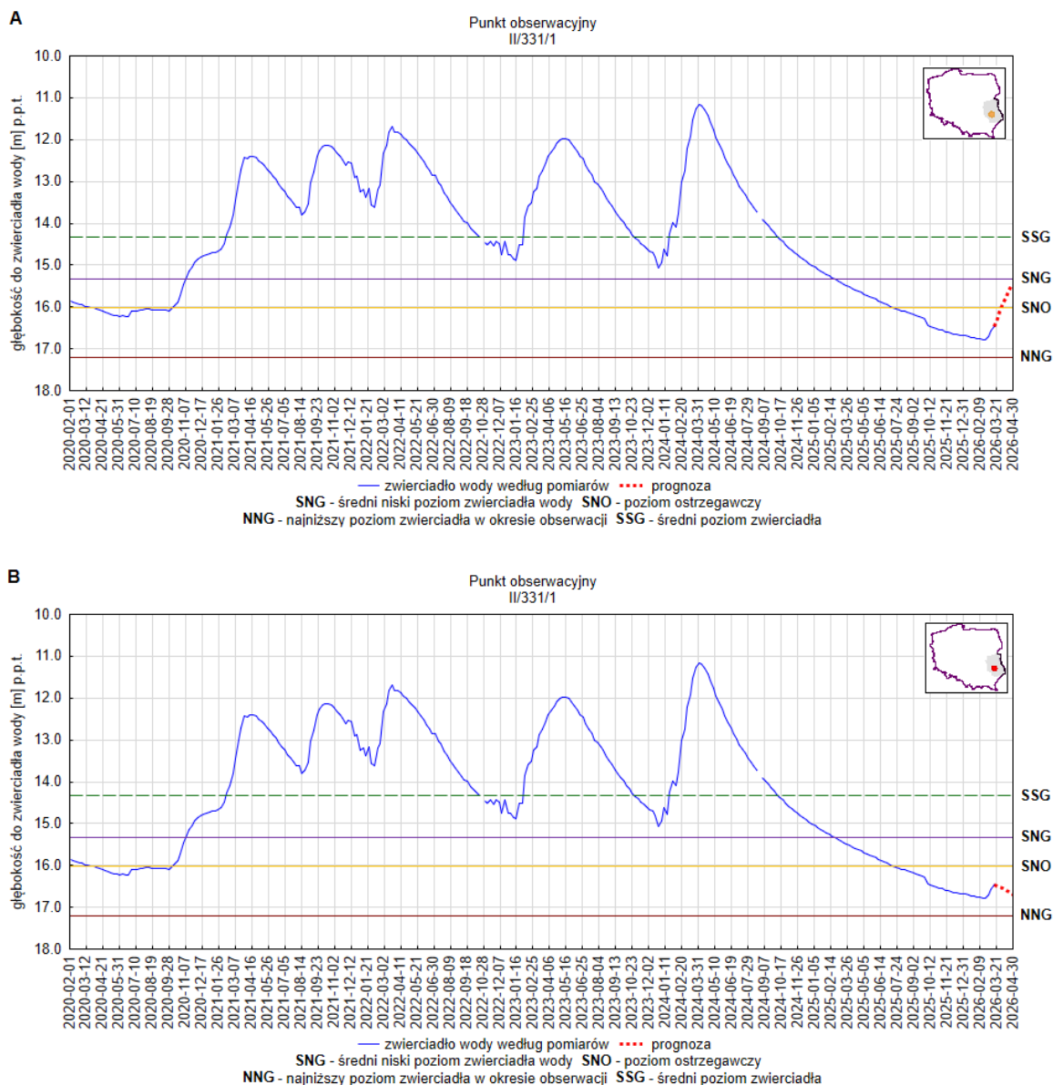
Rys. 5. Prognoza dotycząca stanu wód o zwierciadle swobodnym (gruntowych) na okres 01.04.2026 – 30.04.2026 r. – stacja hydrogeologiczna nr II/331/1 w miejscowości Giełczew Doły (woj. lubelskie). A – prognoza przy założeniu scenariusza A; B – prognoza przy założeniu scenariusza B
