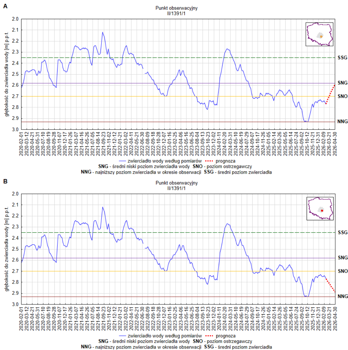
Rys. 8. Prognoza dotycząca stanu wód o zwierciadle swobodnym (gruntowych) na okres 01.04.2026 – 30.04.2026 r. – stacja hydrogeologiczna nr II/1391/1 w miejscowości Sulejów (woj. łódzkie). A – prognoza przy założeniu scenariusza A; B – prognoza przy założeniu scenariusza B
