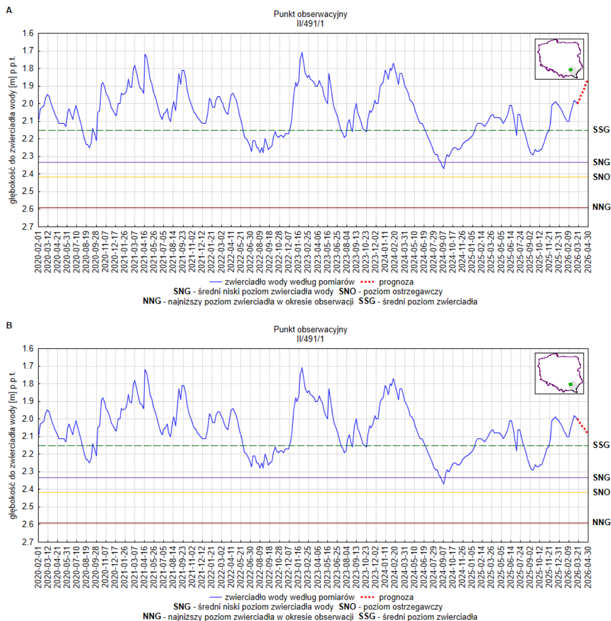
Rys. 14. Prognoza dotycząca stanu wód o zwierciadle swobodnym (gruntowych) na okres 01.04.2026 – 30.04.2026 r. – stacja hydrogeologiczna nr II/491/1 w miejscowości Mielec (woj. podkarpackie). A – prognoza przy założeniu scenariusza A; B – prognoza przy założeniu scenariusza B
