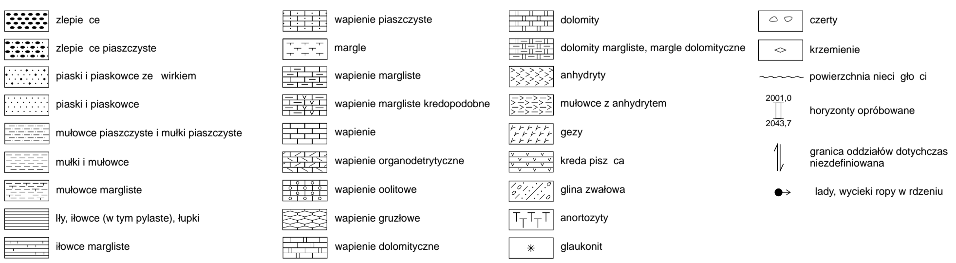
Fig. 3. Profil litologiczno-stratigraficzny otworu wiertniczego K trzyn IG 1
