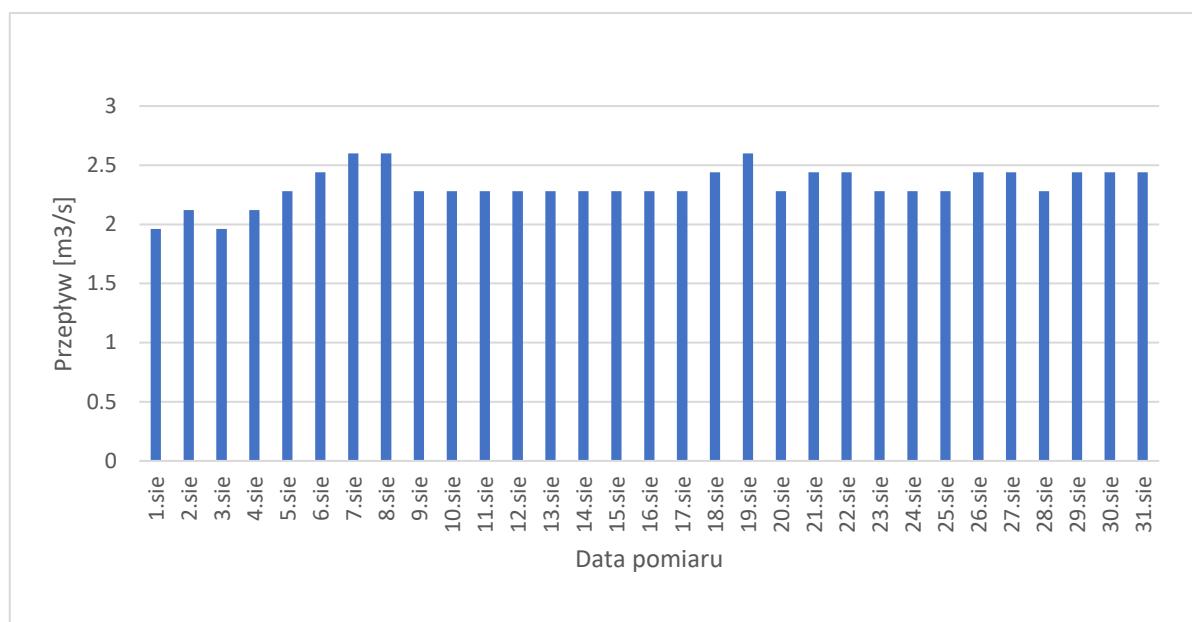
Ryc. 1. Wyniki pomiarów przepływów w sierpniu 2026 r. na rzece Biała Przemsza na stacji hydrologicznej w Sławkowie (źródło: IMGW).
