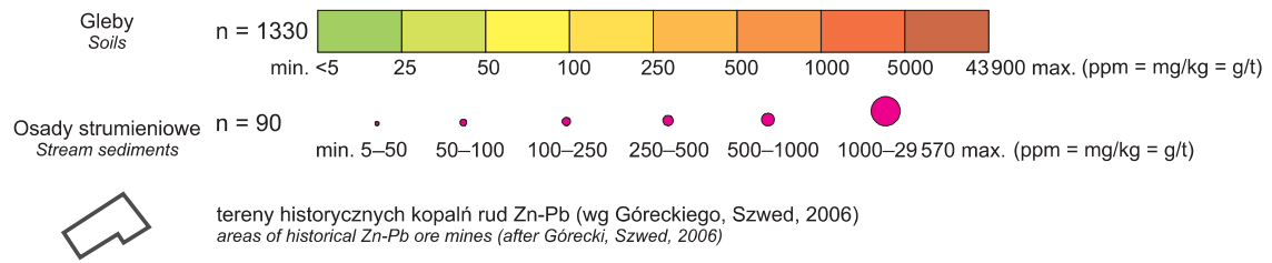
Fig. 3. Zawartość ołowiu w glebach i osadach strumieniowych
