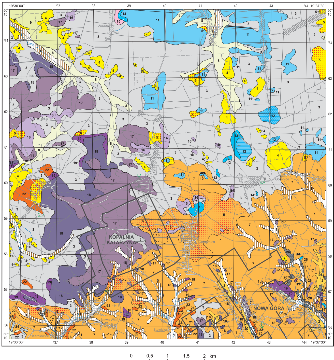
Fig. 1. Mapa geologiczna wg Kurek, Preidl (1992) (objaśnienia na następnej stronie)
