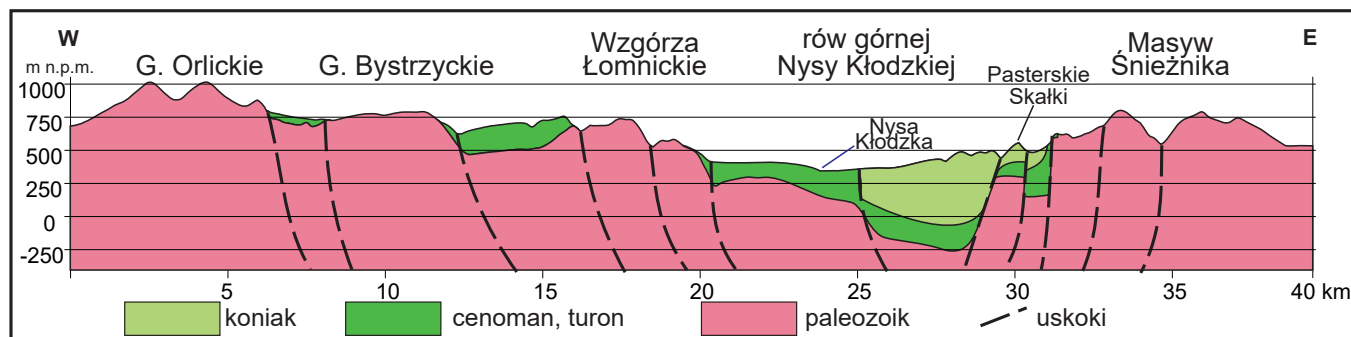
FIG. 4. Przewyższony schematyczny przekrój poprzeczny rowu górnej Nysy Kłodzkiej, ukazujący różnice hipsometryczne położenia utworów górnokredowych będące skutkiem kenozoicznych przemieszczeń blokowych w obrębie rowu oraz w Górach Orlickich i Bystrzyckich
