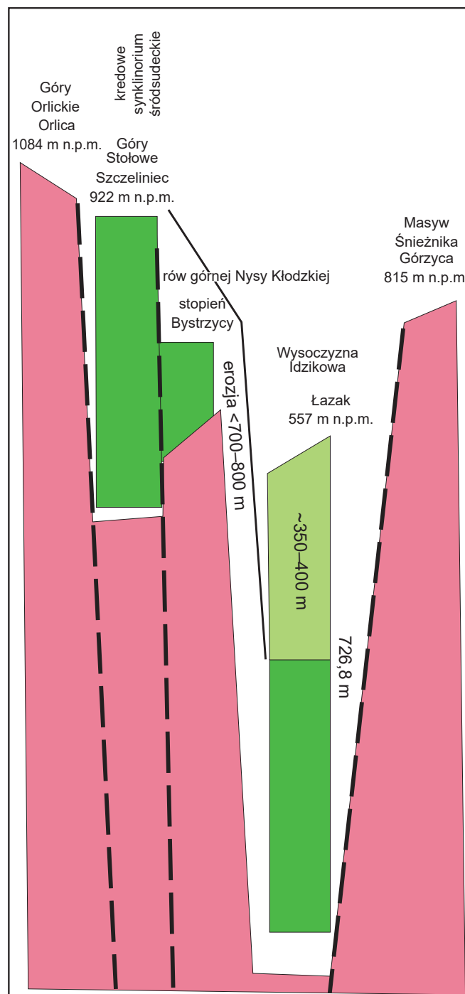
FIG. 5. Tektonicznie uwarunkowane efekty erozji sukcesji skał górnokredowych w zależności od ich pozycji hipsometrycznej w związku z kenozoicznymi przemieszczeniami blokowymi w rejonie rowu górnej Nysy Kłodzkiej. Osady koniak i santonu zachowały się jedynie w pozycji obniżonej w rowie Nysy, zaś zostały zerodowane na wypiętrzonych obrzeżach rowu. Barwy – jak na fig. 4. Miąższości osadów kredowych w Górach Stołowych i na Wysoczyźnie Ildzikowskiej wg Wojewody (1997)
