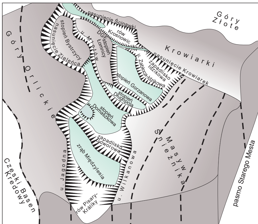
FIG. 3. Blokowa budowa dna rowu górnej Nysy Kłodzkiej i jego ram strukturalnych (wg Badury, Rauch, 2014, na podstawie kompilacji niepublikowanych danych wiertniczych i elektrooporowych). Na figurze trójkątnymi zębami na białym tle oznaczono skarpy w dnie rowu i na jego brzegach, oddzielające od siebie poszczególne stopnie ukształtowania dna – w zależności od położenia względem elementów sąsiednich – określane też jako zręby i rowy. Pola białe (bez zębów) opisują najgłębiej pograżone segmenty dna rowu, pola zielone – segmenty występujące płycej, pola szare – najwyższe wyniesione fragmenty spągu górnej kredy (w NW części rowu) oraz krystaliczne podłoże odsłonięte na ramionach rowu w Masywie Śnieżnika, Krowiarkach oraz na większości obszaru Gór Orlickich (i Bystrzyckich – zlokalizowanych we wschodniej części obszaru opisanego tu zbiorczo pod nazwą Gór Orlickich).
