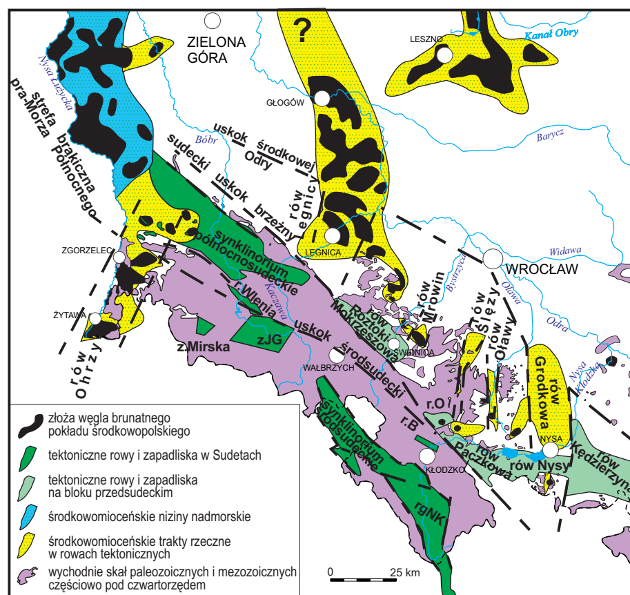
FIG. 1. Kenozoiczne rowy i zapadliska tektoniczne w Sudetach i na bloku przedsudeckim oraz tektonicznie kontrolowane śródkowomiocenijskie traktów rzecznych i obszary bagien w strefie brakicznej pra-Morza Północnego. Skróty: r. – rów tektoniczny, z. – zapadlisko tektoniczne, rgNK – rów górnej Nysy Kłodzkiej, r.B – rów Bierkowic, r.O – rów Ostroszowic, z.JG – zapadlisko Jeleniej Góry
