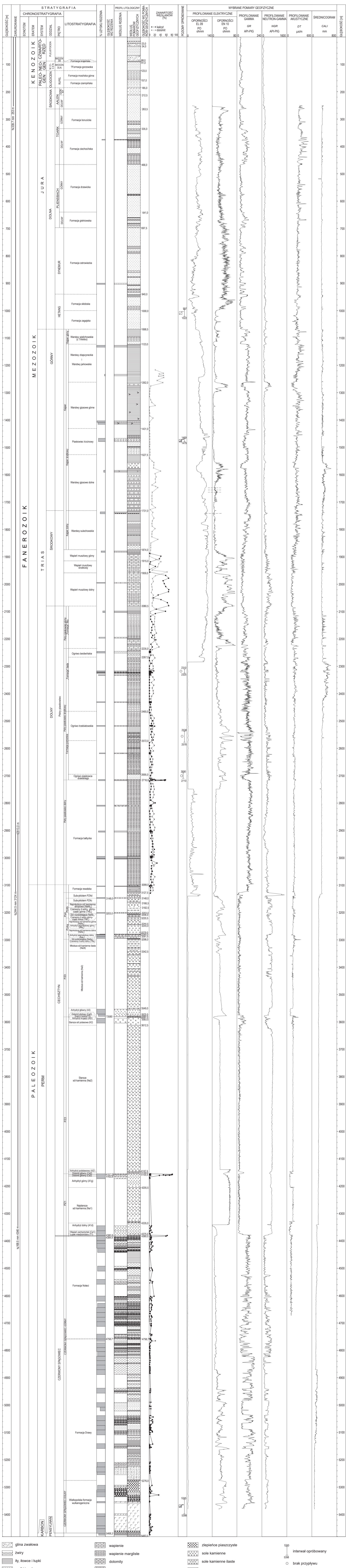
Fig. 2. Profil litologiczno-stratygraficzny otworu Piła 1/IG 1
