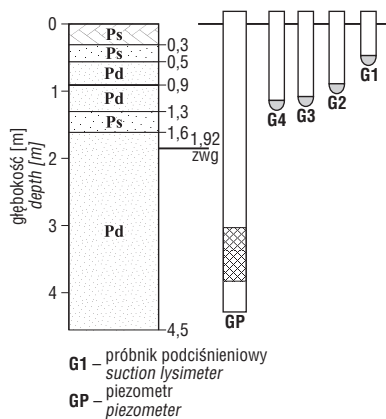
Ryc. 4. Profil geologiczny oraz schemat rozmieszczenia otworów do opróbowań hydrochemicznych. Stacja Granica
