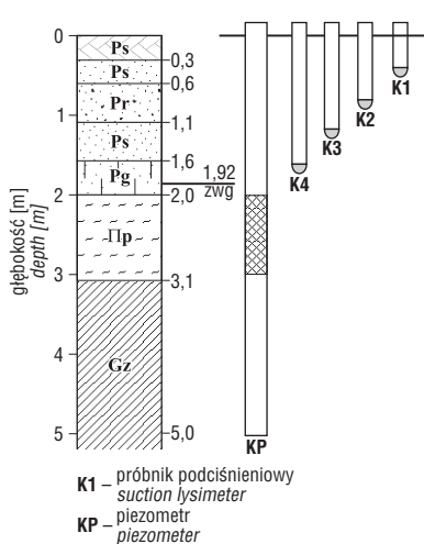
Ryc. 3. Profil geologiczny oraz schemat rozmieszczenia otworów do opróbowań hydrochemicznych. Stacja Kampinos
