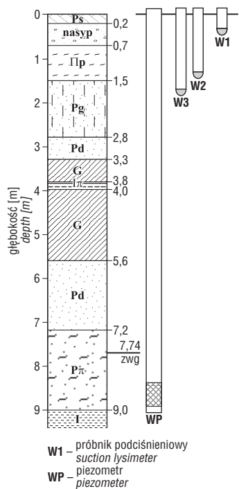
Ryc. 2. Profil geologiczny oraz schemat rozmieszczenia otworów do opróbowań hydrochemicznych. Stacja Warszawa (symbole wg PN-86/B-02480)
