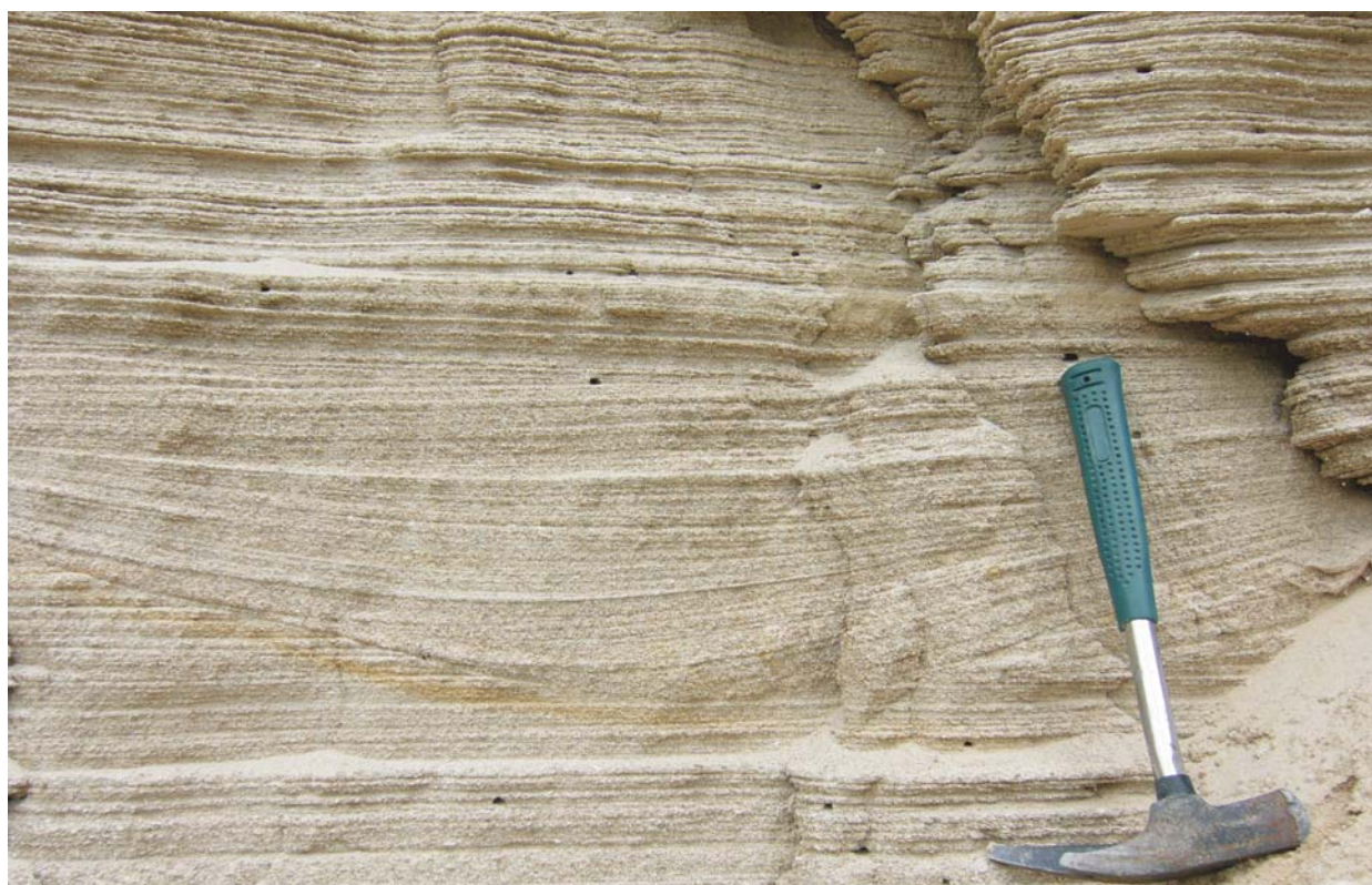
Ryc. 5. Wapienie organodetrytyczno-kwarcowe formacji z Chmielnika, warstwowane horyzontalnie i rynnowo (miocen, północna marginalna strefa zapadliska przedkarpackiego). Obie fot. U. Czarniecka Fig. 5. Quartz-organodetrittic limestones of the Chmielnik Formation with horizontal- and trough cross-bedding (Miocene, northern marginal zone of the Carpathian Foredeep). Both photos by U. Czarniecka
