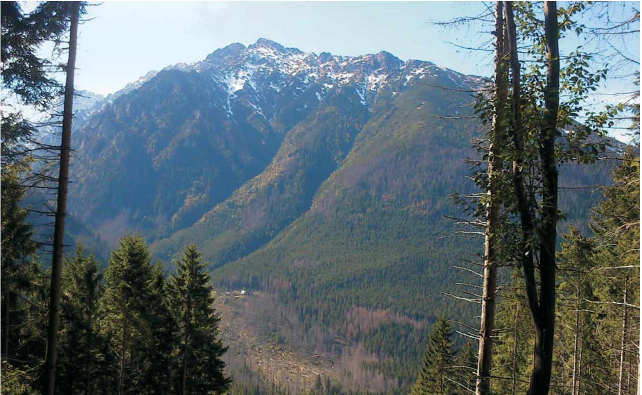
Ryc. 1. Masyw Wołoszyna w Tatarach Wysokich oddzielający Dolinę Waksmundzką od Doliny Roztoki, zbudowany z granodiorytów i tonalitytów równoziarnistych (karbon) – widok od wschodu z rejonu Rozpadliny (Słowacja)
