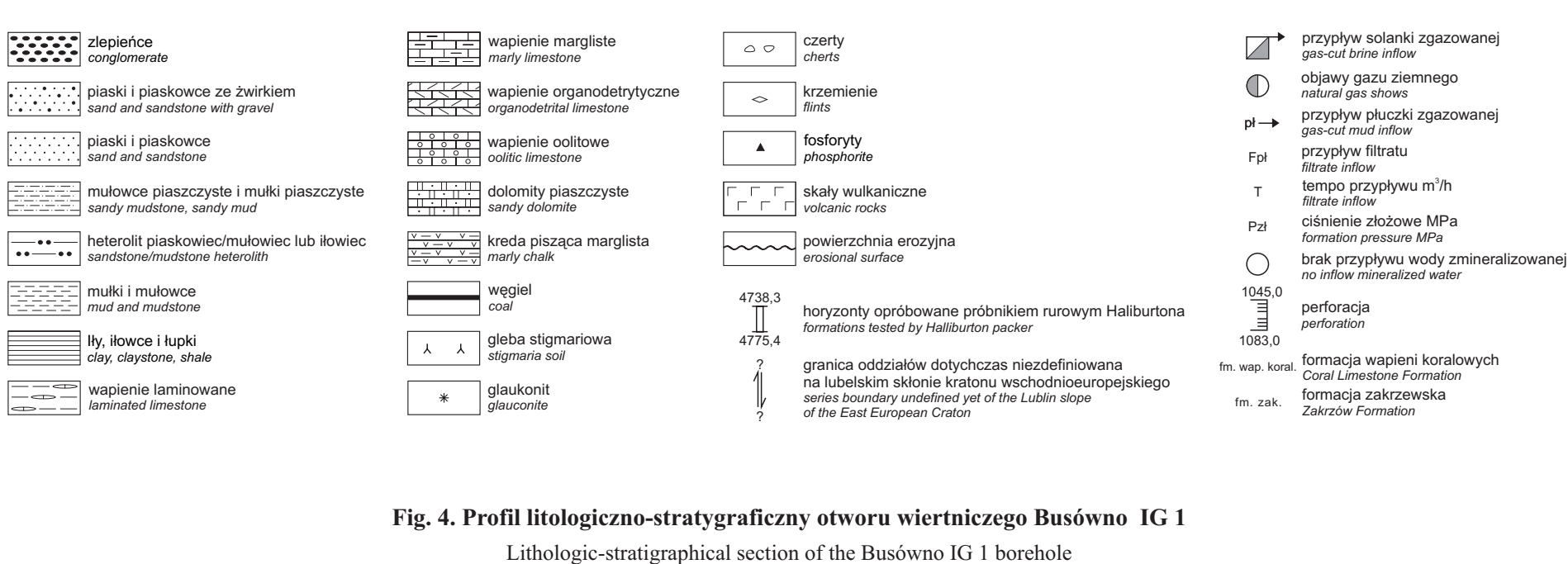
Fig. 4. Profil litologiczno-stratygraficzny otworu wiertniczego Busówno IG 1 Lithologic-stratigraphical section of the Busówno IG 1 borehole
