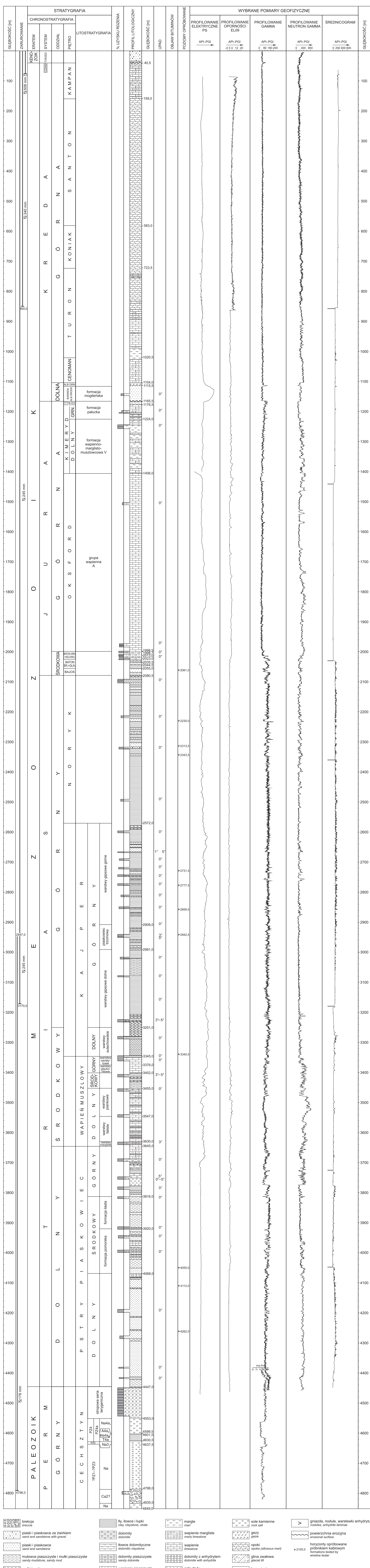
Fig. 4. Profil litologiczno-stratigraficzny otworu wiertniczego Piotrków Trybunalski IG 1 Lithological-stratigraphical section of the Piotrków Trybunalski IG 1 borehole
