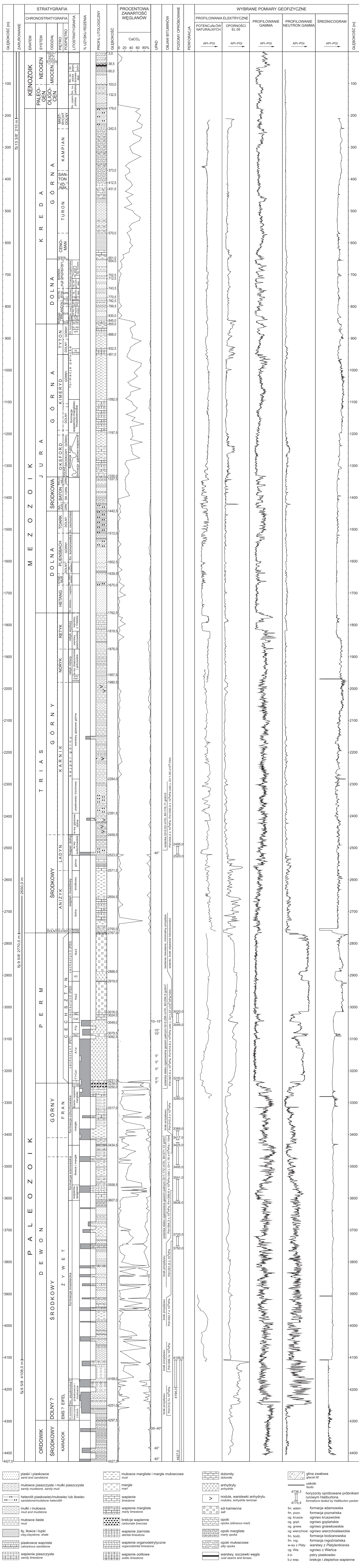
Fig. 3. Profil litologiczno-stratigraficzny otworu wiertniczego Polskie Łąki PIG 1 Lithologic-stratigraphical profile of the Polskie Łąki PIG 1 borehole
