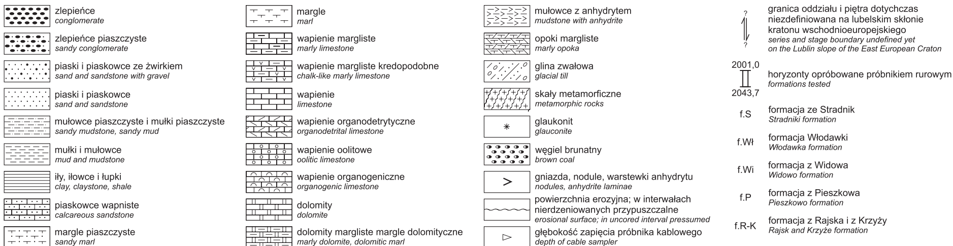
Fig. 3. Profil litologiczno-stratygraficzny otworu wiertniczego Wrotnów IG 1
