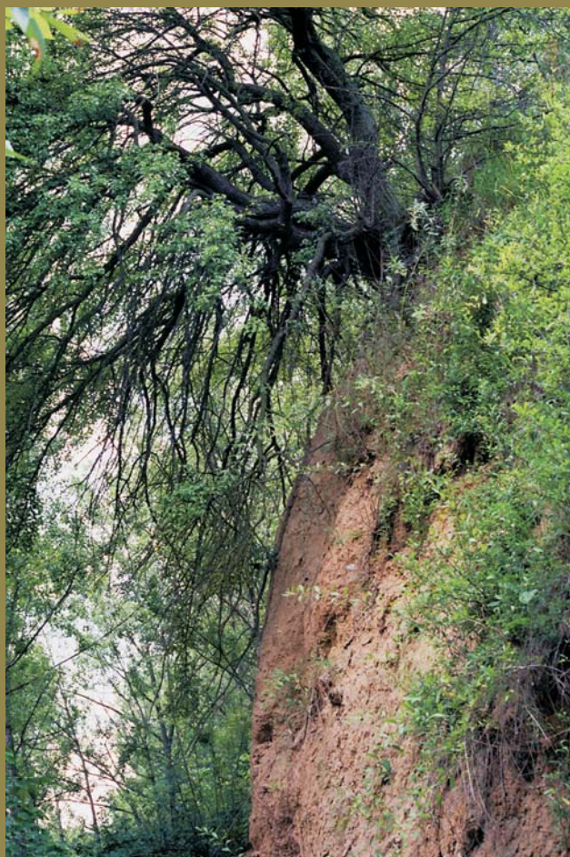
Ryc. 1. Skarpa w Wyszogrodzie — przejawy aktywności procesów zboczowych: obrywy i „pijany las”
