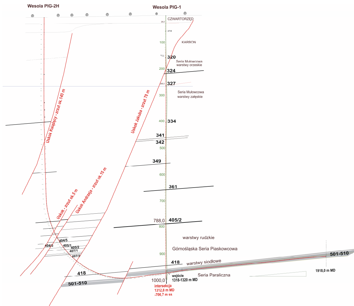
Fig. 3. Trajektoria osi wiercenia Wesola PIG-2H z uwzględnieniem otworu Wesola PIG-1 i miejsca intersekcji
