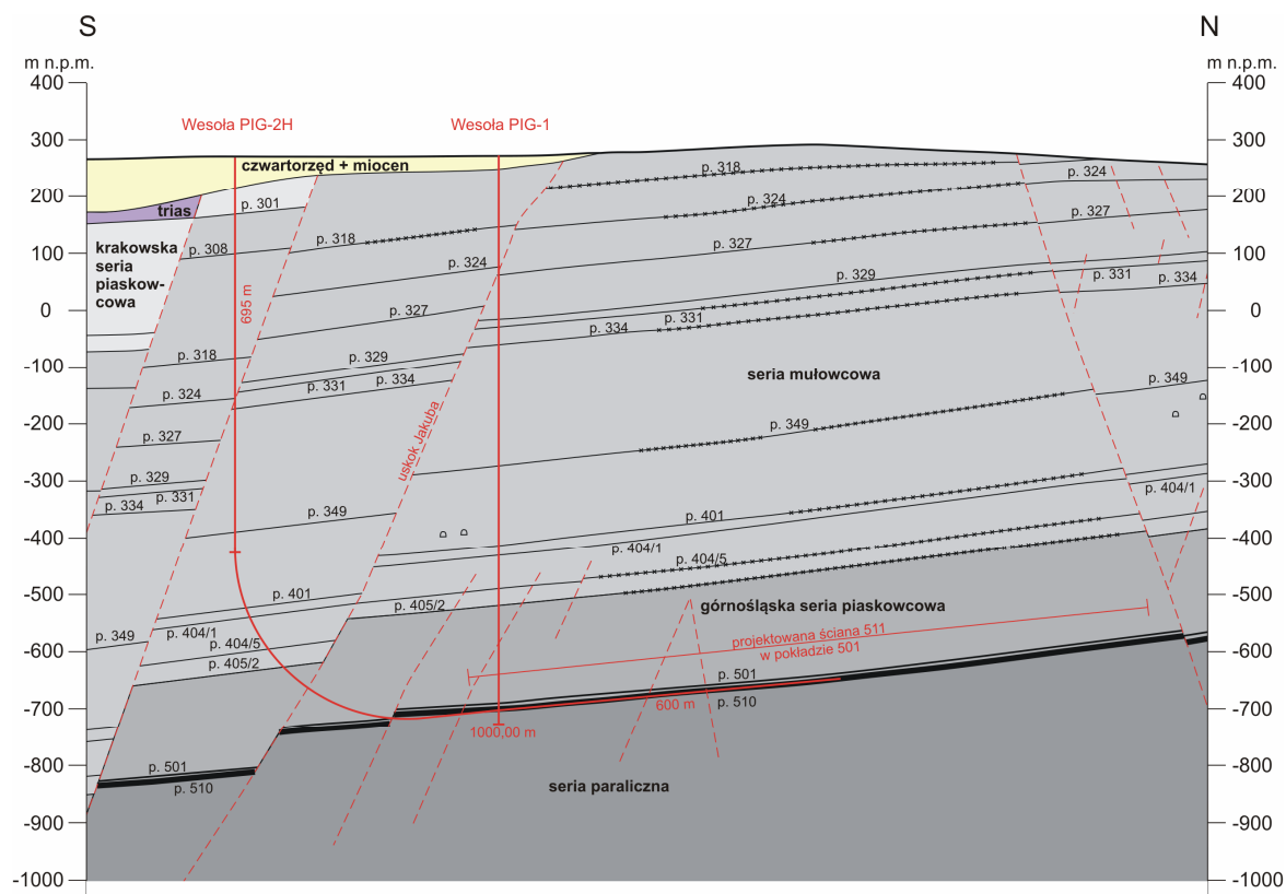
Fig. 2. Położenie wiercni Wesola PIG-1 i Wesola PIG-2H na przekroju geologicznym
