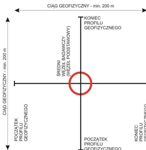
Rysunek 2. Schemat rozmieszczenia badań w lokalizacji 5 i 7
