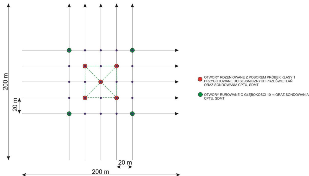
Rysunek 3. Schemat rozmieszczenia badań w lokalizacji 6
