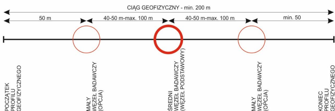
Rysunek 1. Schemat rozmieszczenia badań w lokalizacjach 1-4
