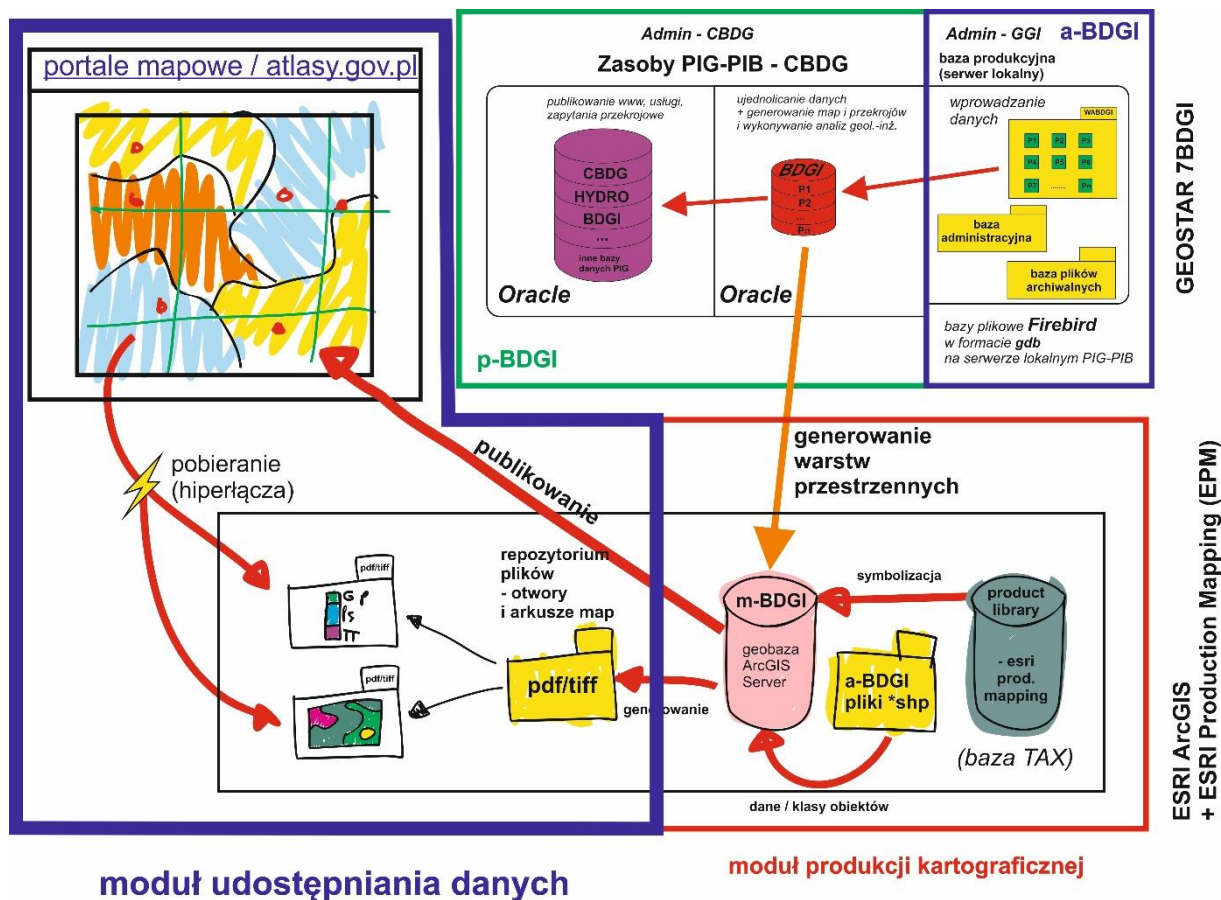
Fig. 2. Schemat koncepcyjny Systemu Przetwarzania Danych Geologiczno-Inżynierskich (SPDGI). Na schemacie uwypuklono moduł udostępniania danych oraz moduł produkcji kartograficznej.
