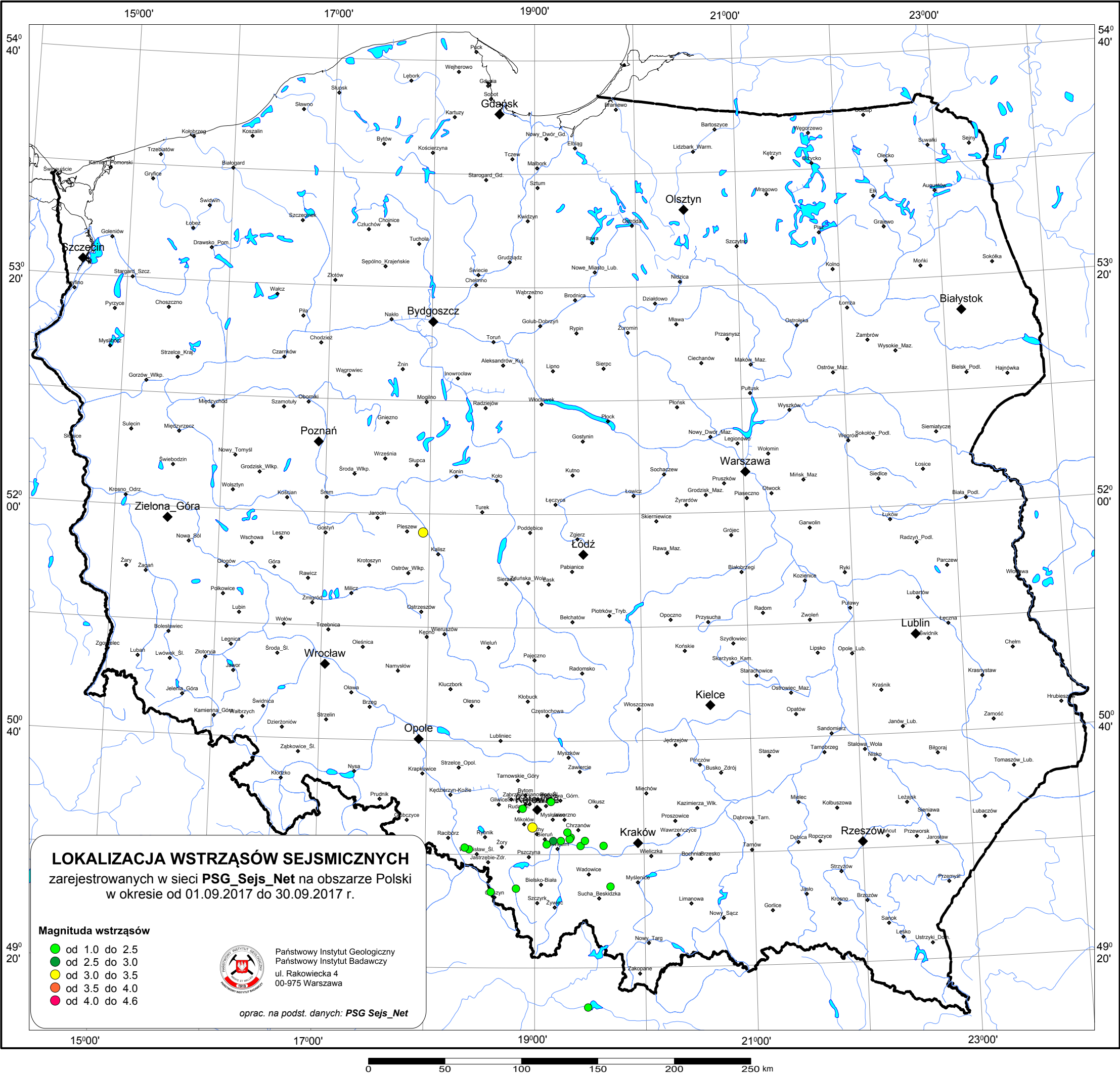
Statystyka wstrząsów w m-cu wrześniu 2017 r.
