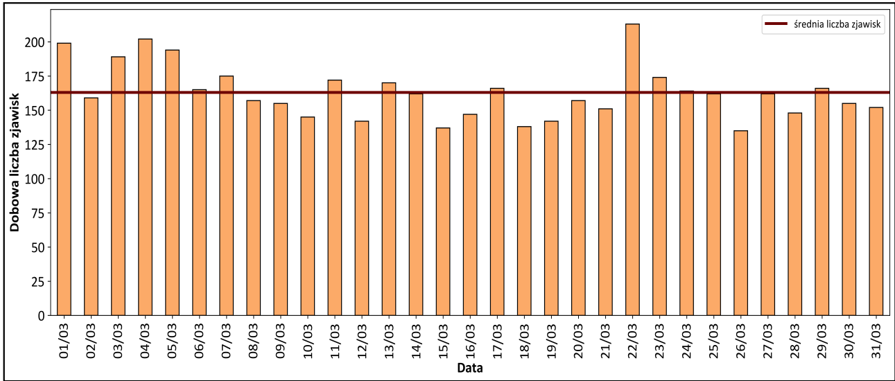
Aktywność sejsmiczna na świecie w okresie 01/03/2024 - 31/03/2024 r. (dobowa liczba zjawisk o magnitudzie M>2.5)
