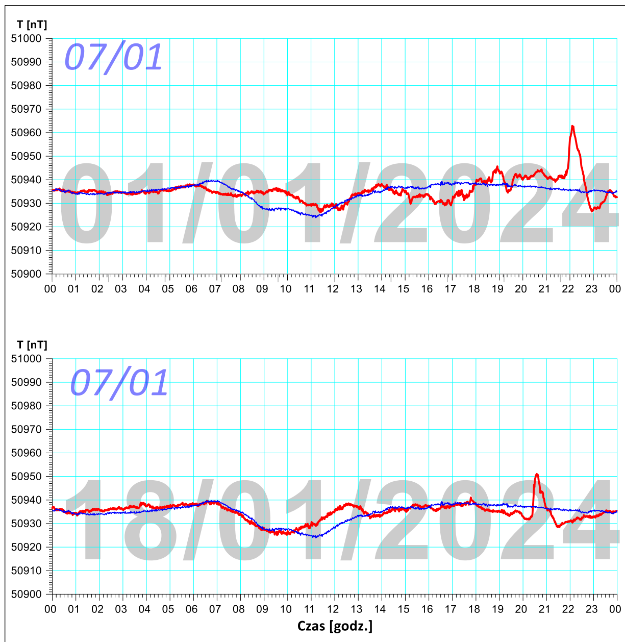
Rys. 4. Wykresy dobowe zmian modułu całkowitego wektora pola geomagnetycznego w dniach 01/01; 18/01/2024 (UTC) zarejestrowane na stacji monitoringu geodynamicznego PSG w Hołownie, gm. Podedwórze, pow. parczewski. Kolorem niebieskim wykreślono zmiany dobowe indukcji pola magnetycznego zarejestrowane w dniu 07/01/2024 (najniższy poziom zakłóceń nieperiodycznych zarejestrowanych dobowo w styczniu br. – „dobowa krzywa referencyjna”).
