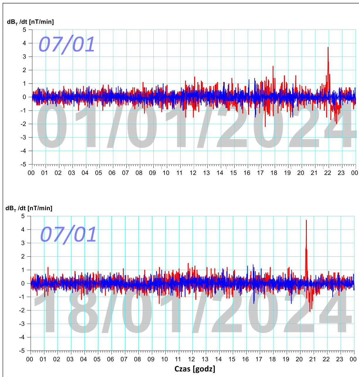
Rys. 5. Wykresy dobowe tempa zmian modułu całkowitego wektora pola geomagnetycznego dB_T/dt w dniach 01/01; 18/01/2024 r. (UTC) zaobserwowane na stacji monitoringu geodynamicznego PSG w Hołownie, gm. Podedwórze, pow. parczewski. Kolorem niebieskim wykreślono dobowy przebieg tempa zmian indukcji pola magnetycznego zarejestrowane w dniu 07/01/2024 (najniższy poziom zakłóceń nieperiodycznych zarejestrowanych dobowo w styczniu br. – „dobowa krzywa referencyjna”).
