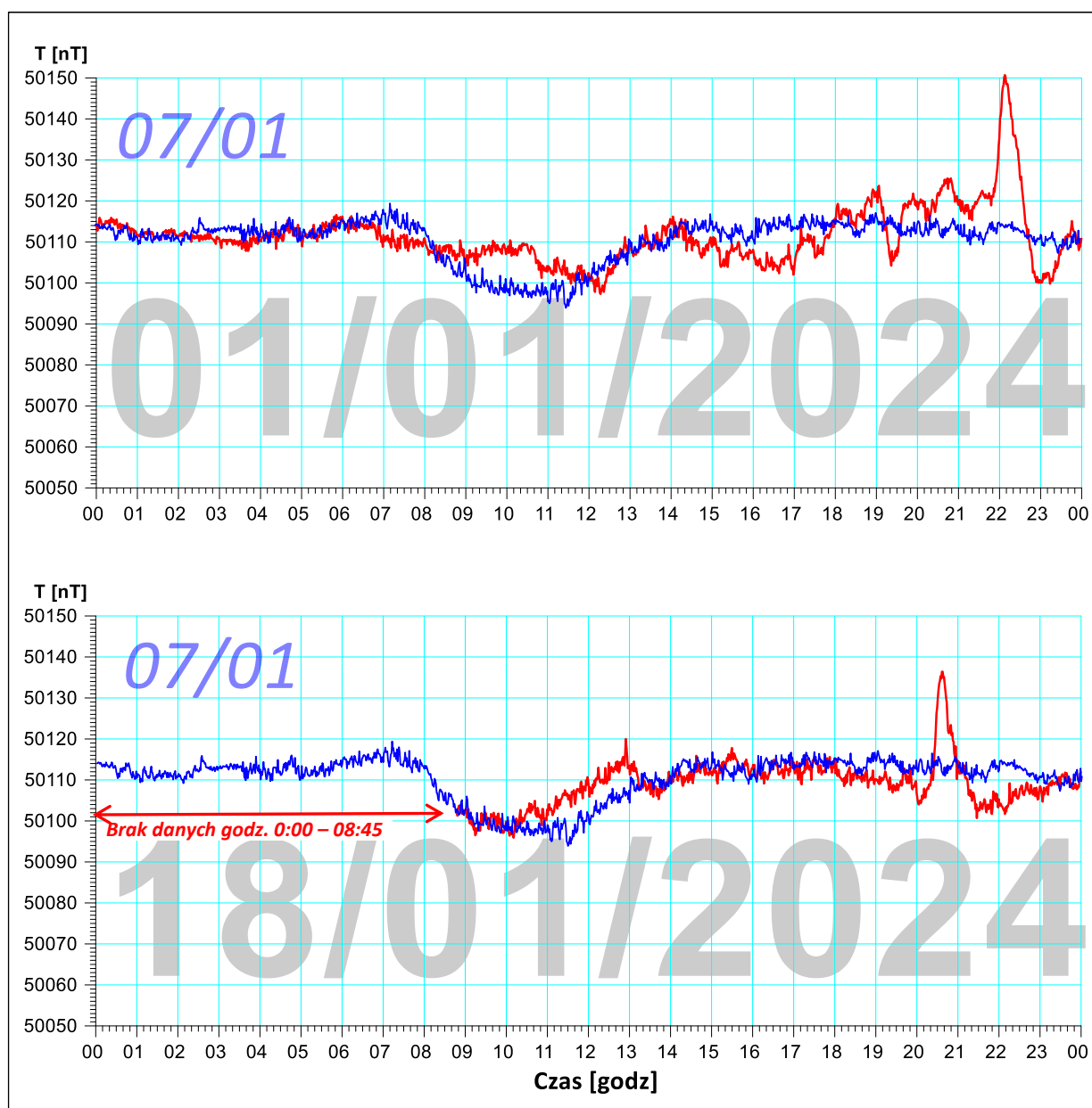
Rys. 2. Wykresy dobowe zmian modułu całkowitego wektora pola geomagnetycznego w dniu 01/01/2024 oraz 18/01/2024 (UTC) zarejestrowane na stacji monitoringu geodynamicznego PSG w Dziwiu, gm. Przedeck, pow. kolski. Kolorem niebieskim wykreślono zmiany dobowe indukcji pola magnetycznego zarejestrowane w dniu 07/01/2024 (najniższy poziom zakłóceń nieperiodycznych zarejestrowanych w czasie jednej doby w styczniu br. – „dobowa krzywa referencyjna”).
