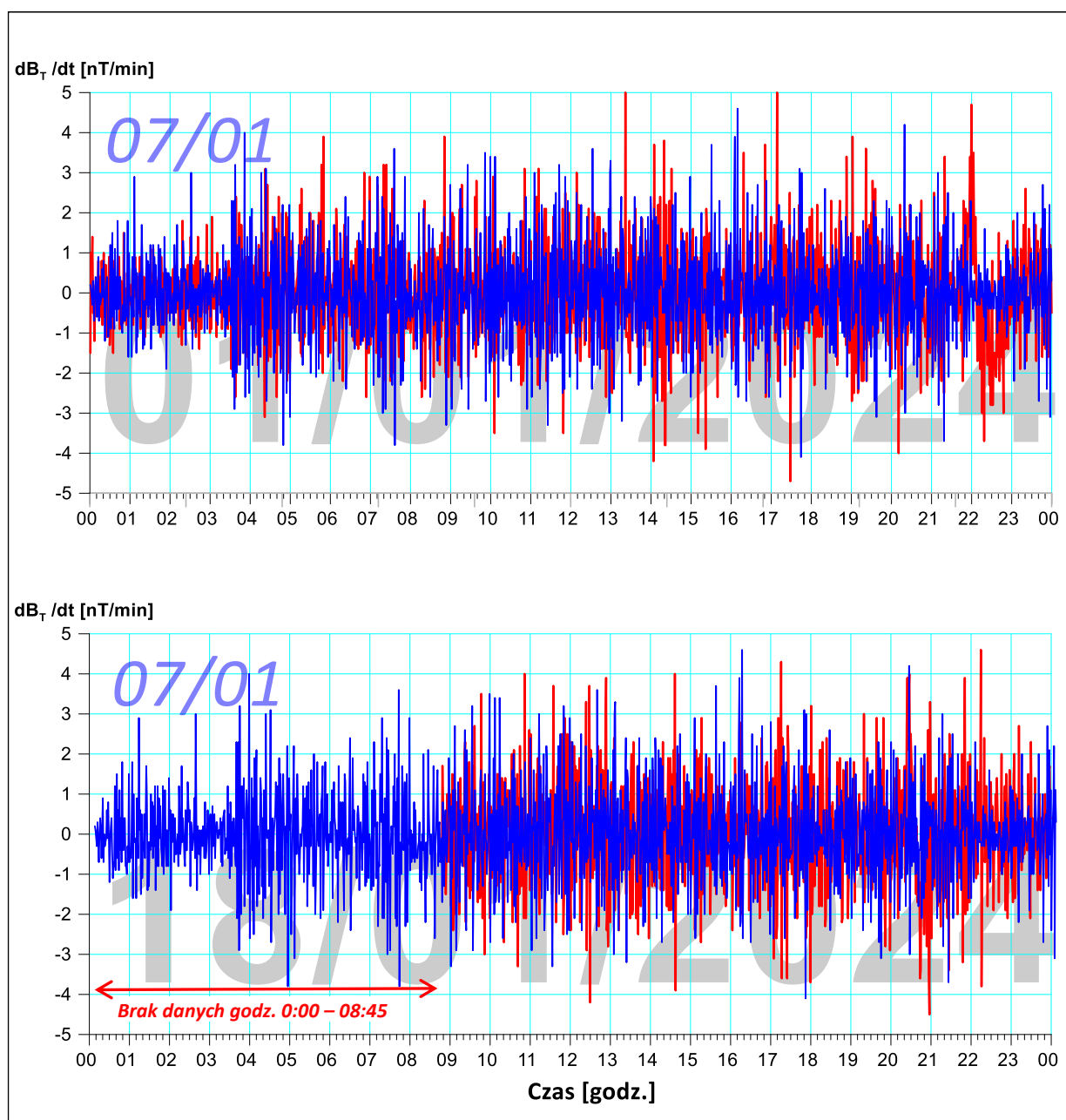
Rys. 3. Wykresy dobowe tempa zmian modułu indukcji całkowitego wektora pola geomagnetycznego dB_T/dt w dniu 01/01/2024 oraz 18/01/2024 r. (UTC) zaobserwowane na stacji monitoringu geodynamicznego PSG w Dziwiu, gm. Przedecz, pow. kolski. Kolorem niebieskim wykreślono dobowy przebieg tempa zmian indukcji pola magnetycznego zarejestrowane w dniu 07/01/2024 (najniższy poziom zakłóceń nieperiodycznych zarejestrowanych w czasie jednej doby w styczniu br. – „dobowa krzywa referencyjna”).
