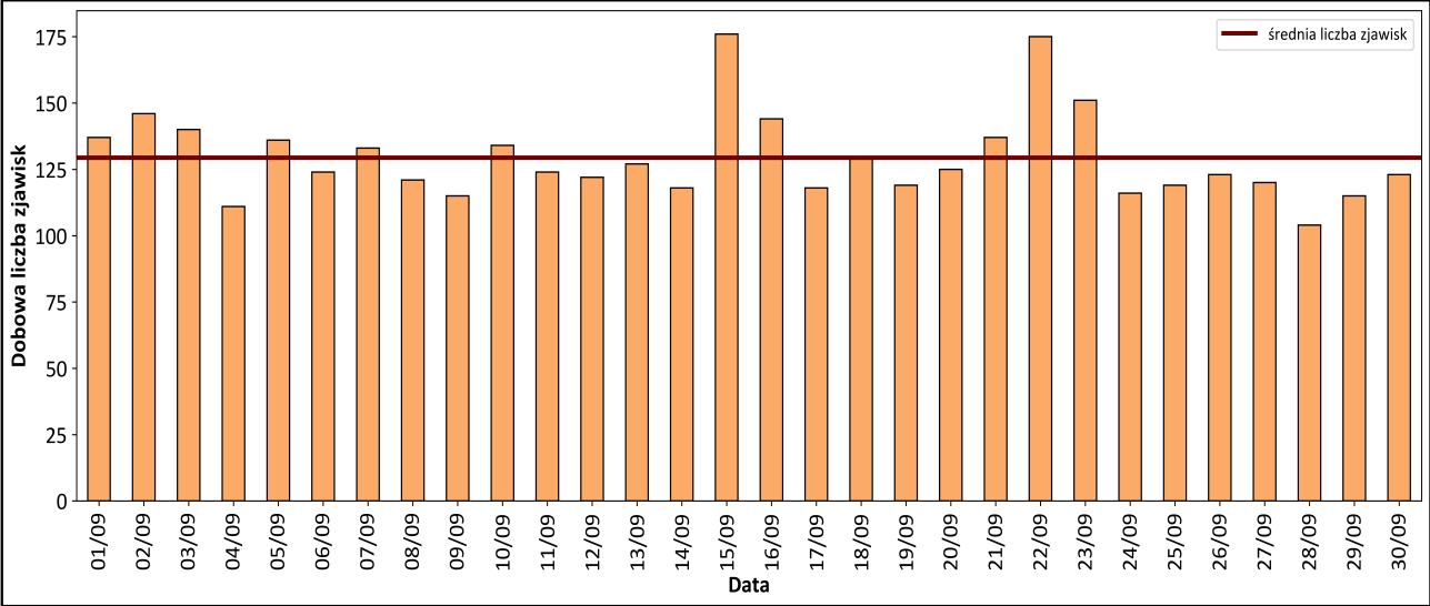
Aktywność seismiczna na świecie w okresie 01/09/2024 - 30/09/2024 r. (dobowa liczba zjawisk o magnitudzie M>2.5)
