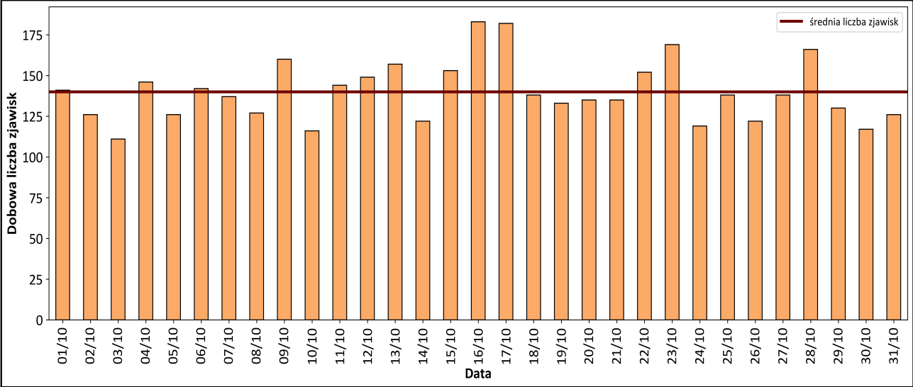
Aktywność sejsmiczna na świecie w okresie 01/10/2024 - 31/10/2024 r. (dobowa liczba zjawisk o magnitudzie M>2.5)
