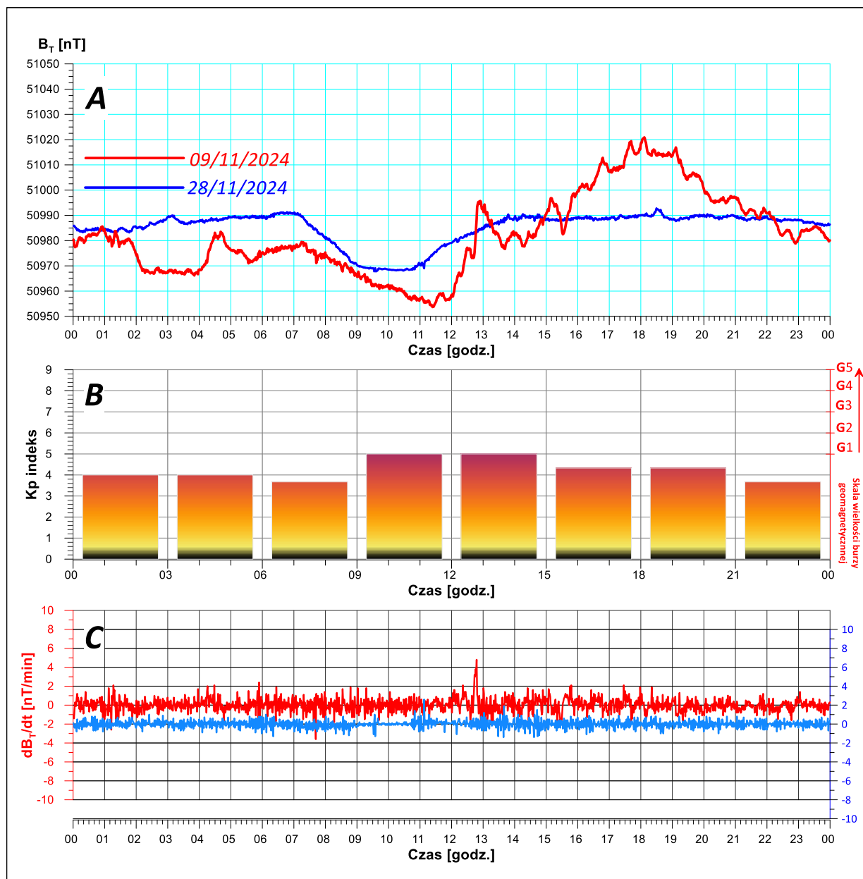
Rys. 3. Magnetogram z monitoringu modułu całkowitego wektora indukcji pola geomagnetycznego zarejestrowany w dniu 09/11/2024 r. na stacji geodynamicznej PSG zlokalizowanej w Hołownie (gm. Podedworze, pow. parczewski).
