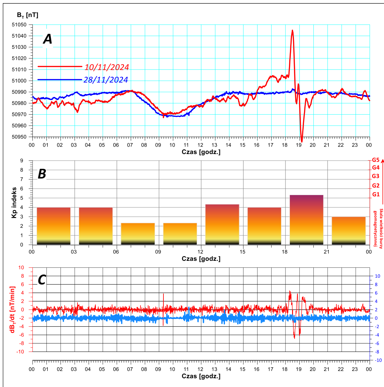
Rys. 4. Magnetogram z monitoringu modułu całkowitego wektora indukcji pola geomagnetycznego zarejestrowany w dniu 10/11/2024 r. na stacji geodynamicznej PSG zlokalizowanej w Hołownie (gm. Podedworze, pow. parczewski).
