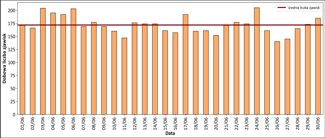
Aktywność sejsmiczna na świecie w okresie 01/06/2025 - 30/06/2025 r. (dobowa liczba zjawisk o magnitudzie M>2.5)
