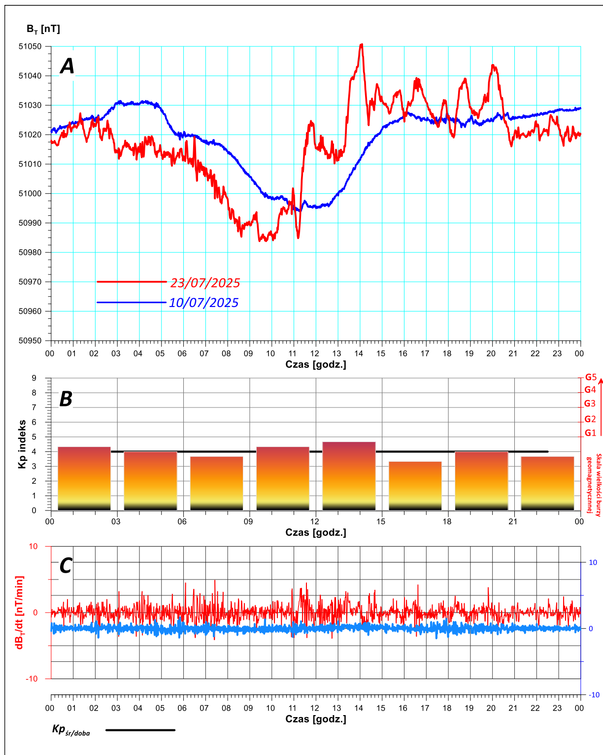
Rys. 4. Magnetogram z monitoringu modułu całkowitego wektora indukcji pola geomagnetycznego zarejestrowany w dniu 23/07/2025 r. na stacji geodynamicznej PSG zlokalizowanej w Hołownie (gm. Podedwórze, pow. parczewski).
