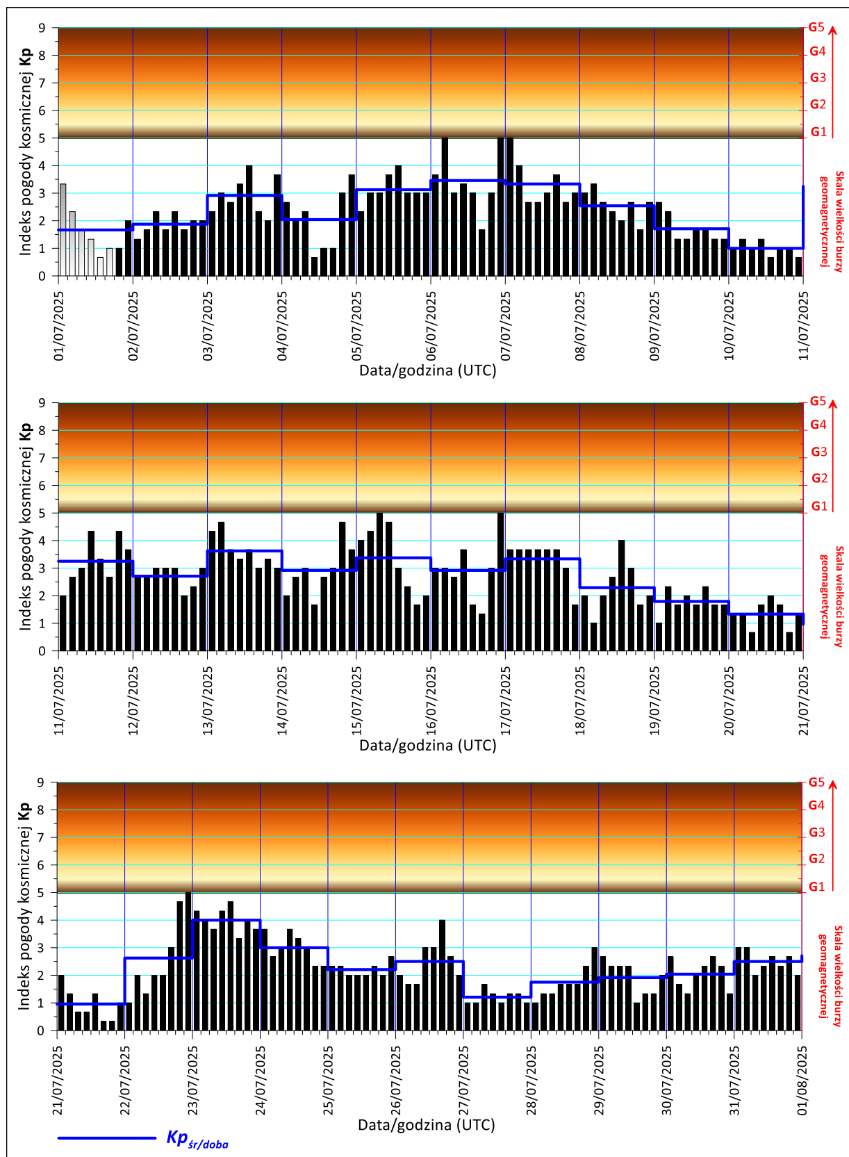
Rys. 2. Zmiany indeksu Kp pogody kosmicznej w miesiącu lipcu 2025 r. (dane wg. NOAA).
