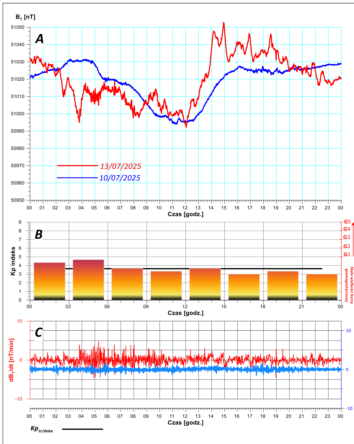
Rys. 3. Magnetogram z monitoringu modułu całkowitego wektora indukcji pola geomagnetycznego zarejestrowany w dniu 13/07/2025 r. na stacji geodynamicznej PSG zlokalizowanej w Hołownie (gm. Podedworze, pow. parczewski).
