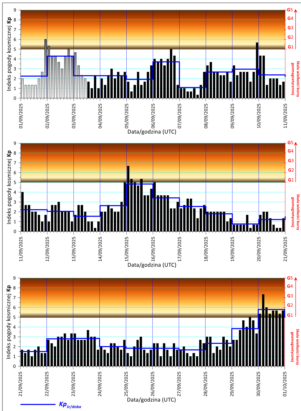
Rys. 2. Zmiany indeksu Kp pogody kosmicznej w miesiącu wrześniu 2025 r. (dane wg. NOAA).
