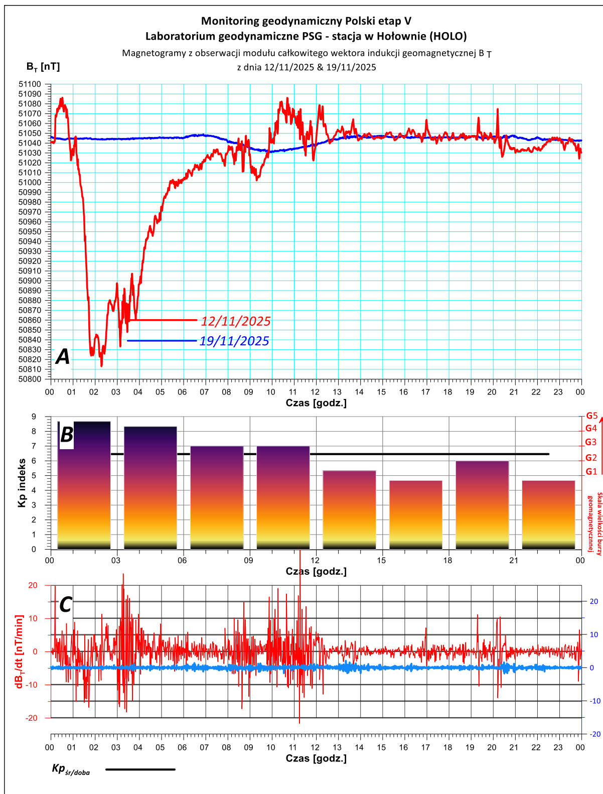
Rys. 4. Magnetogram z monitoringu modułu całkowitego wektora indukcji pola geomagnetycznego zarejestrowany w dniu 12/11/2025 r. na stacji geodynamicznej PSG zlokalizowanej w Hołownie (gm. Podedworze, pow. parczewski).
