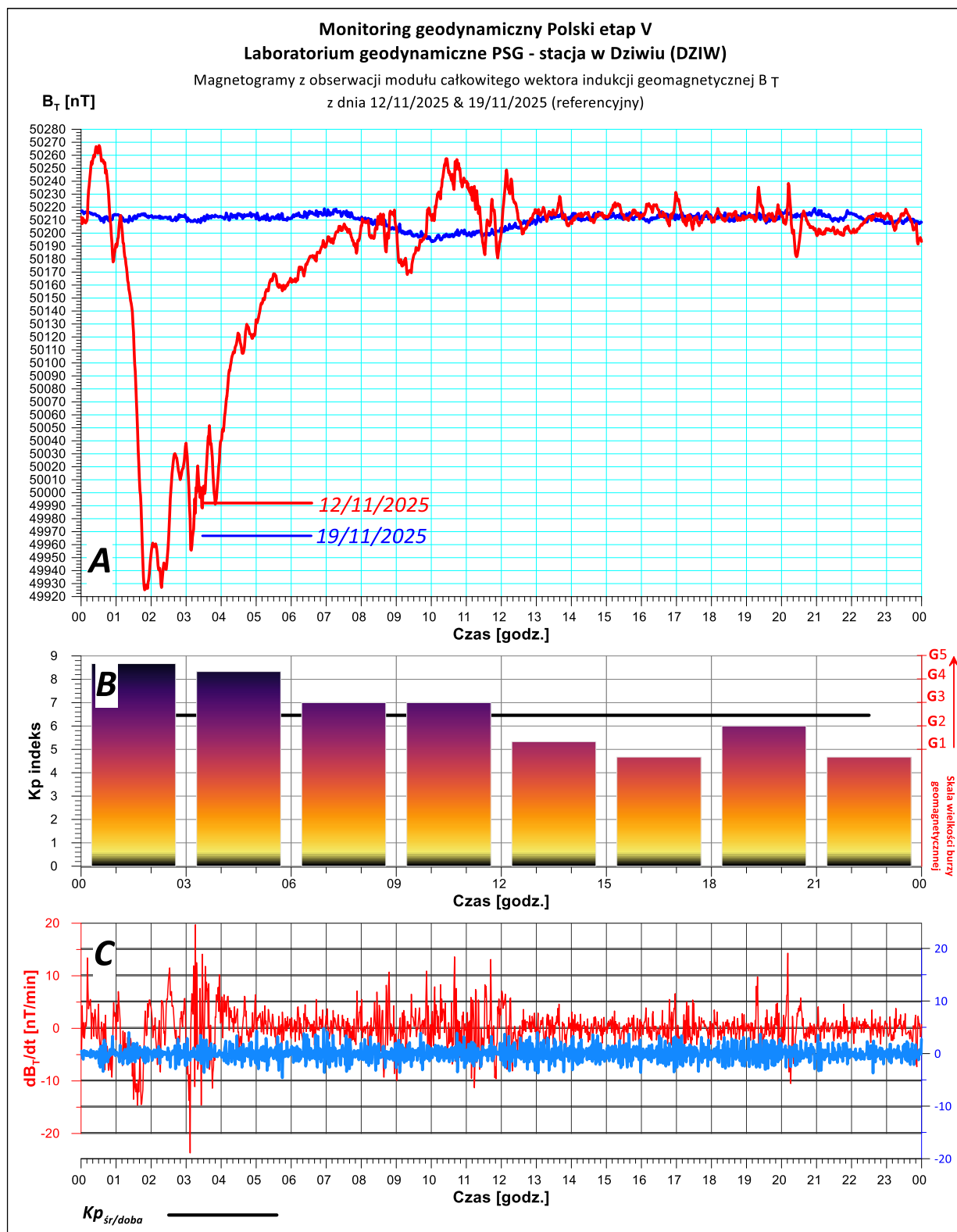
Rys. 5. Magnetogram z monitoringu modułu całkowitego wektora indukcji pola geomagnetycznego zarejestrowany w dniu 12/11/2025 r. na stacji geodynamicznej PSG zlokalizowanej w Dziwiu (gm. Przedecz, pow. kolski).
