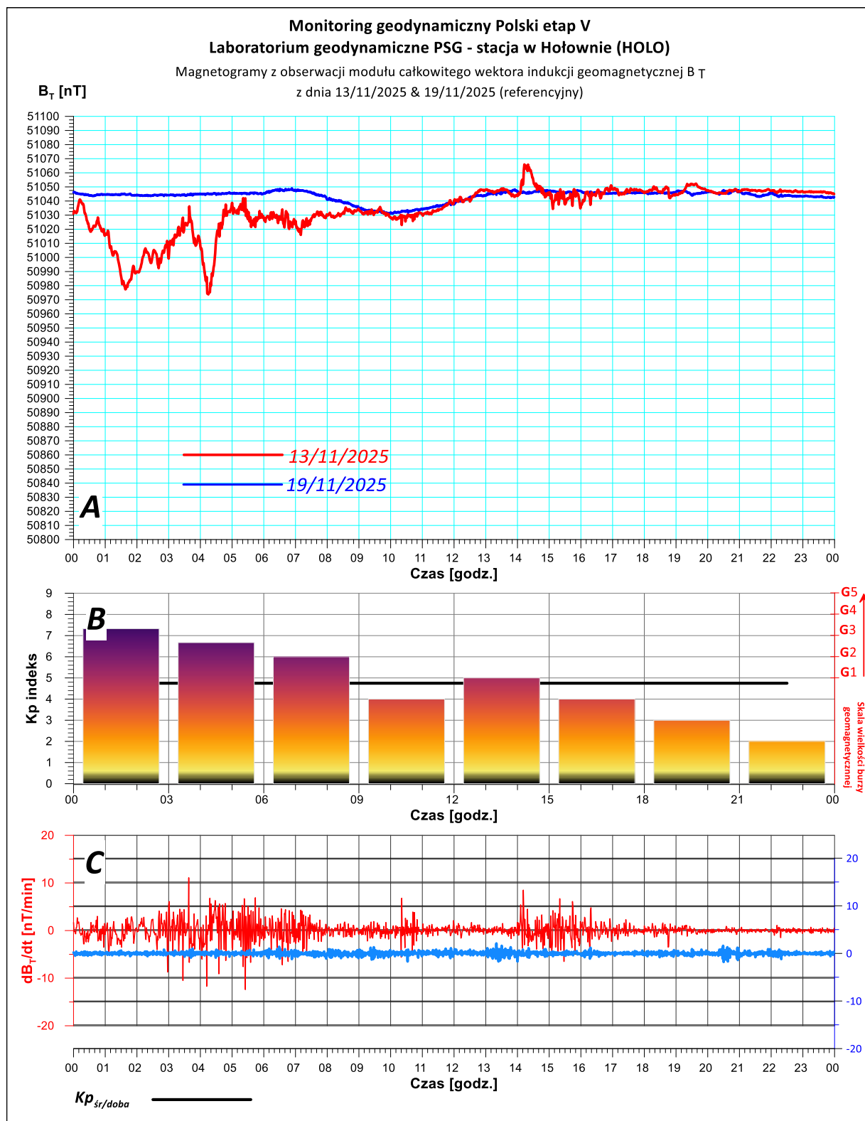
Rys. 4. Magnetogram z monitoringu modułu całkowitego wektora indukcji pola geomagnetycznego zarejestrowany w dniu 13/11/2025 r. na stacji geodynamicznej PSG zlokalizowanej w Hołownie (gm. Podedwórze, pow. parczewski).
