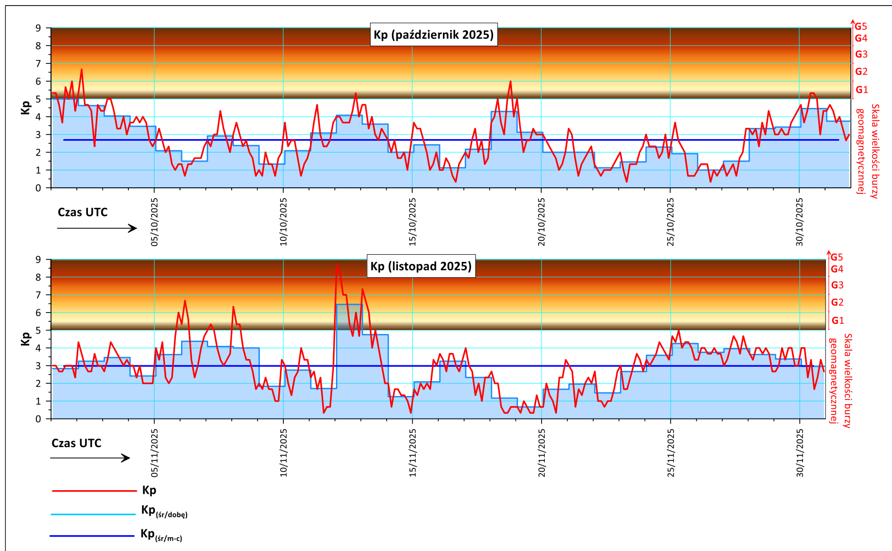
Rys. 3. Zmiany wartości indeksu pogody kosmicznej pod wpływem wiatru słonecznego Kp w październiku i listopadzie 2025 (wg. NOAA-SWPC – Centrum Prognoz Pogody Kosmicznej www.swpc.noaa.gov.us ).
