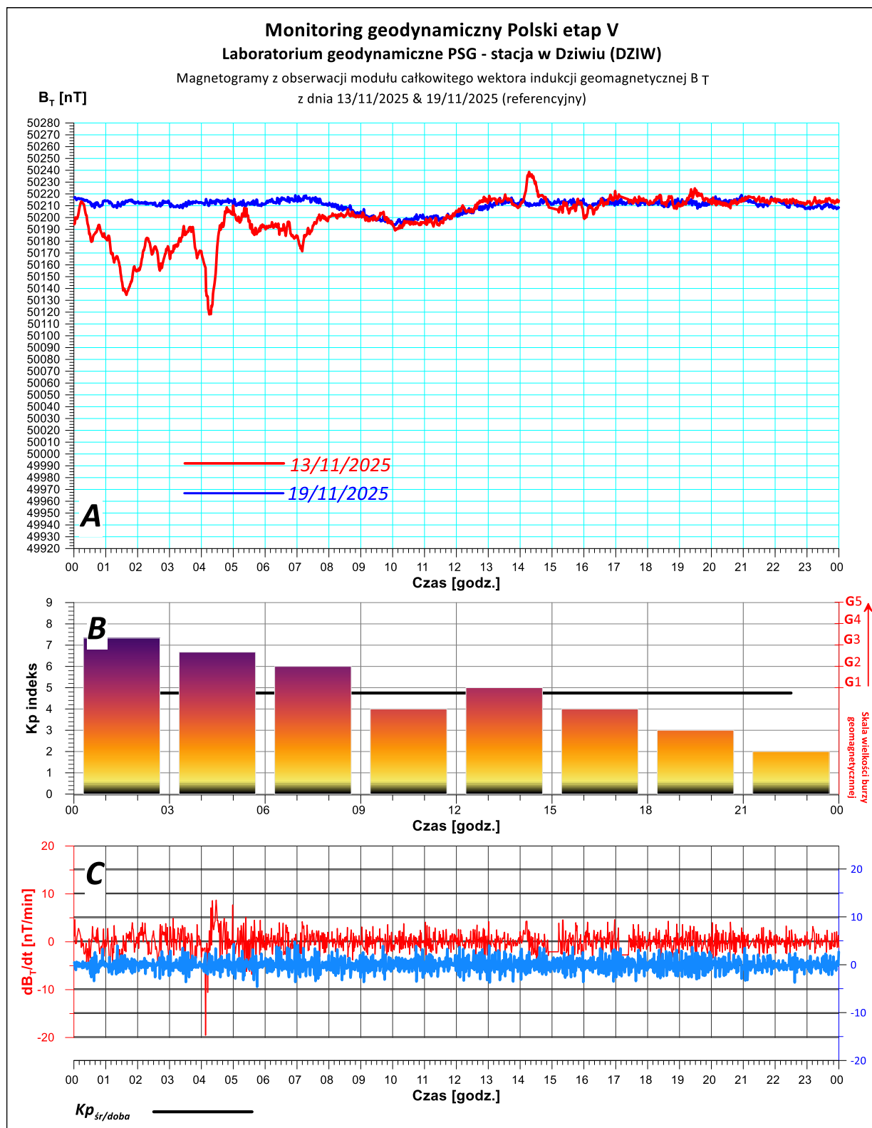
Rys. 6. Magnetogram z monitoringu modułu całkowitego wektora indukcji pola geomagnetycznego zarejestrowany w dniu 13/11/2025 r. na stacji geodynamicznej PSG zlokalizowanej w Dziwiu (gm. Przedecz, pow. kolski).
