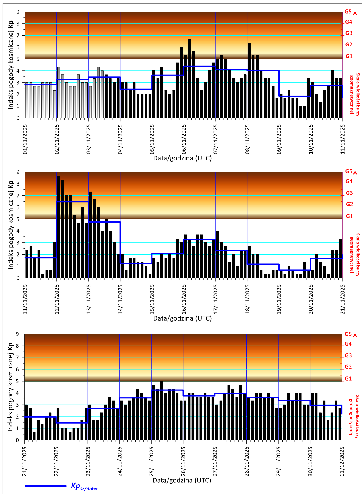
Rys. 2. Zmiany indeksu Kp pogody kosmicznej w miesiącu listopadzie 2025 r. (dane wg. NOAA).
