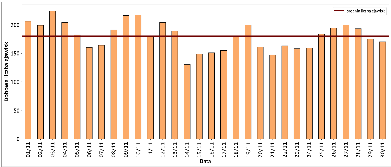
Aktywność sejsmiczna na świecie w okresie 01/11/2025 - 30/11/2025 r. (dobowa liczba zjawisk o magnitudzie M>2.5)
