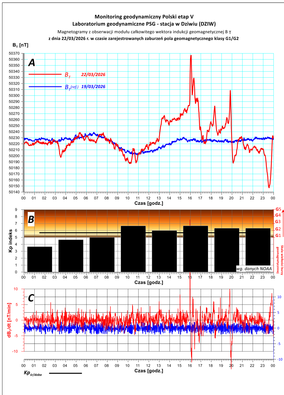
Rys. 7. Magnetogram z monitoringu modułu całkowitego wektora indukcji pola geomagnetycznego zarejestrowany w dniu 22/03/2026 r. na stacji geodynamicznej PSG zlokalizowanej w Dziwiu (gm. Przedecz, pow. kolski).
