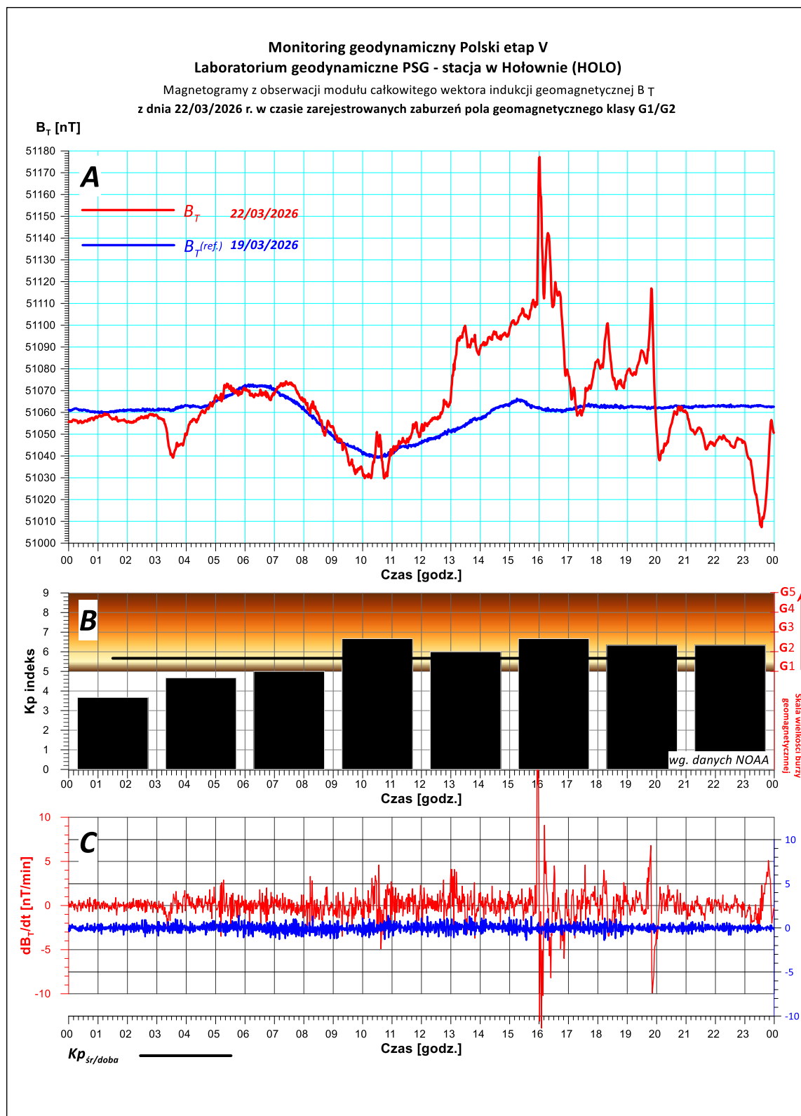
Rys. 5. Magnetogram z monitoringu modułu całkowitego wektora indukcji pola geomagnetycznego zarejestrowany w dniu 22/03/2026 r. na stacji geodynamicznej PSG zlokalizowanej w Hołownie (gm. Podewórze, pow. parczewski).
