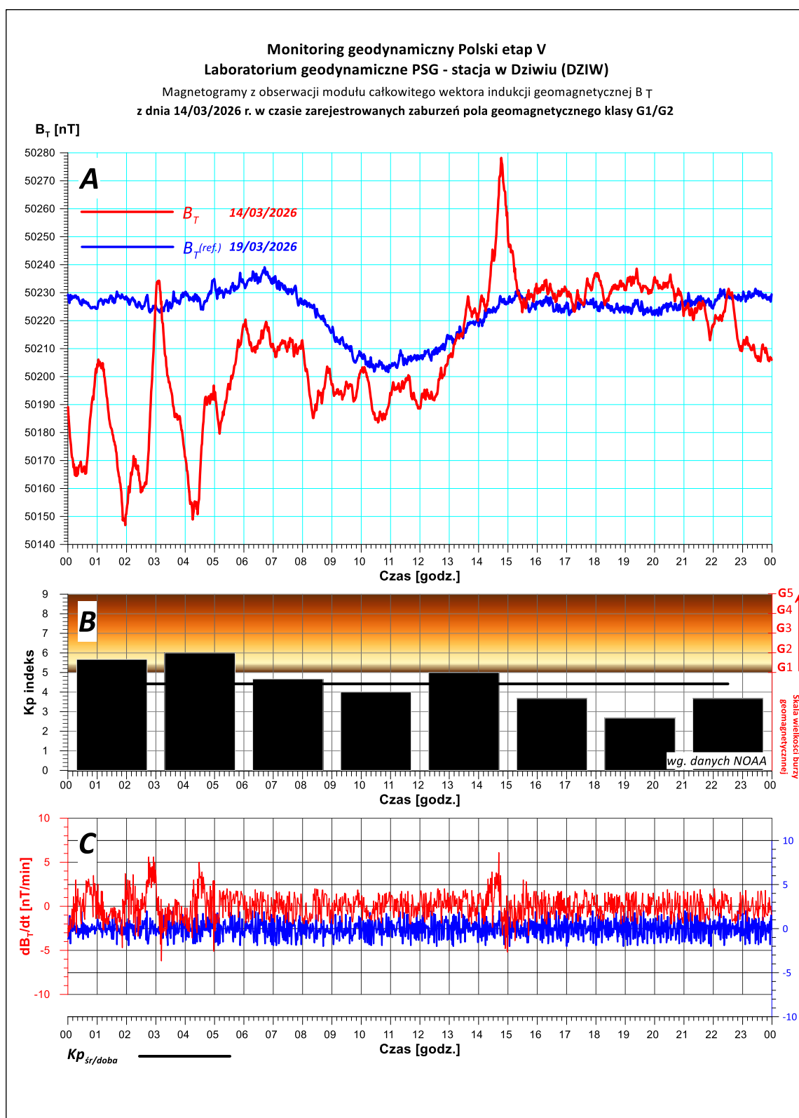
Rys. 6. Magnetogram z monitoringu modułu całkowitego wektora indukcji pola geomagnetycznego zarejestrowany w dniu 14/03/2026 r. na stacji geodynamicznej PSG zlokalizowanej w Dziwiu (gm. Przedecz, pow. kolski).
