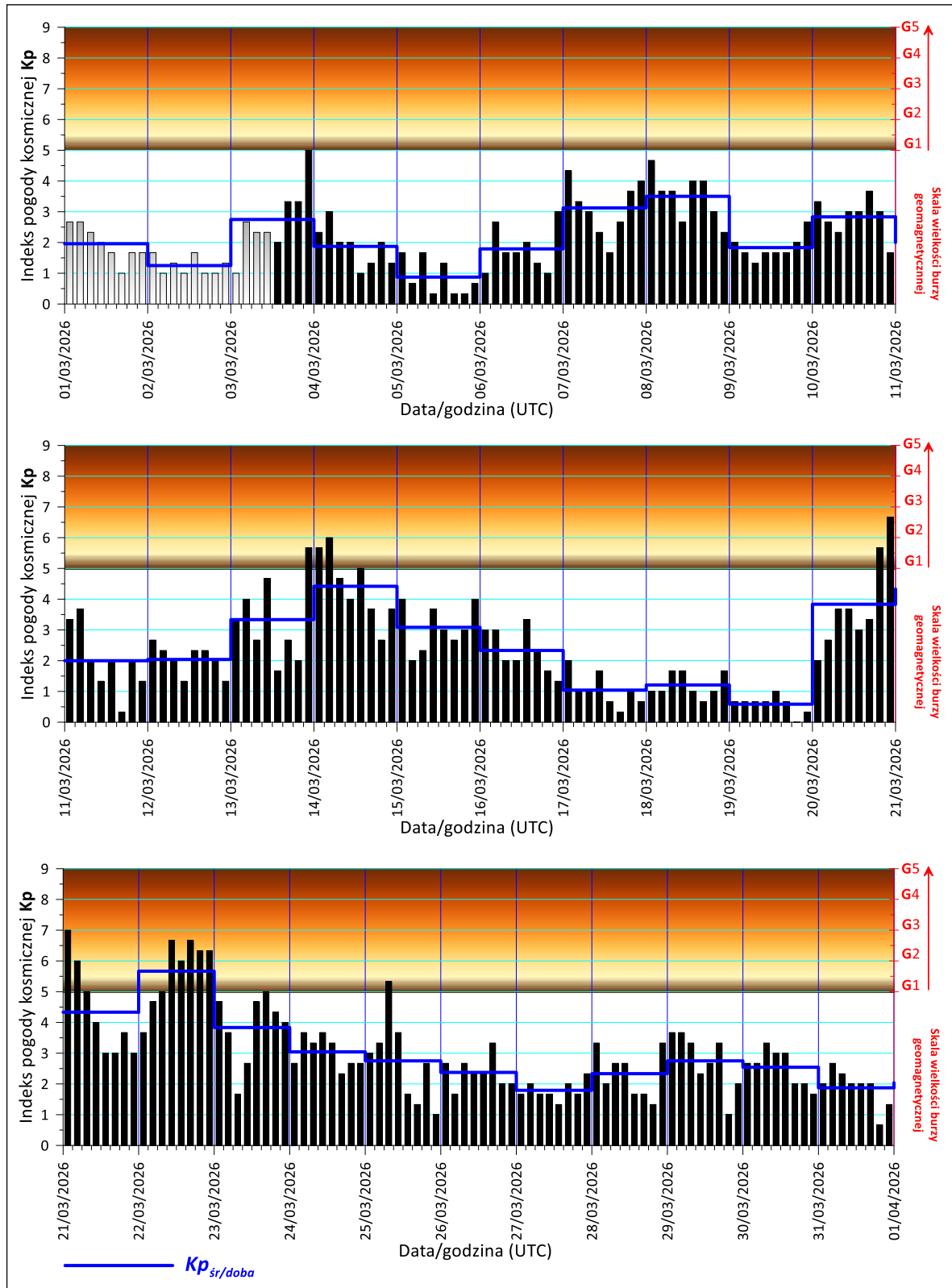
Rys. 2. Zmiany indeksu Kp pogody kosmicznej w miesiącu marcu 2026 r. (oprac. PSG, dane wg. NOAA).
