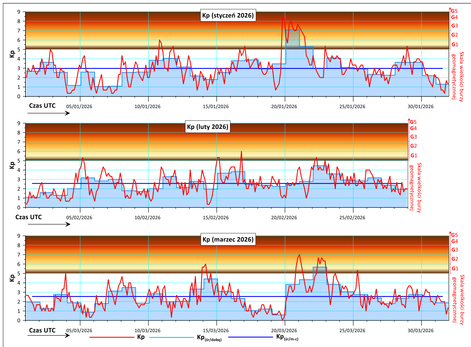
Rys. 3. Zmiany wartości indeksu pogody kosmicznej pod wpływem wiatru słonecznego Kp w styczniu 2026, lutym 2026 oraz w marcu 2026 r. (oprac. PSG, wg. danych NOAA-SWPC – Centrum Prognoz Pogody Kosmicznej www.swpc.noaa.gov.us ).
