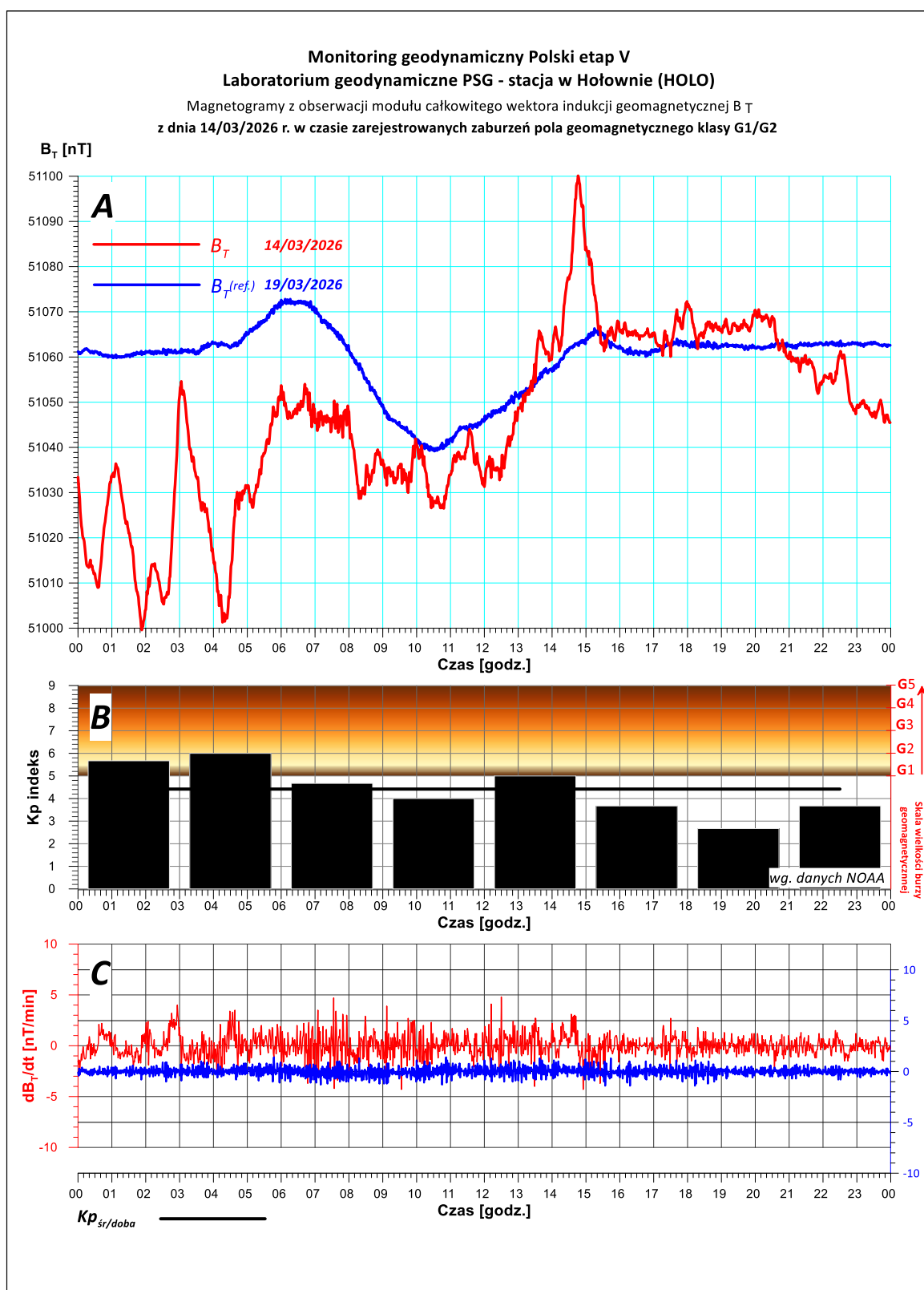
Rys. 4. Magnetogram z monitoringu modułu całkowitego wektora indukcji pola geomagnetycznego zarejestrowany w dniu 14/03/2026 r. na stacji geodynamicznej PSG zlokalizowanej w Hołownie (gm. Podedworze, pow. parczewski).
