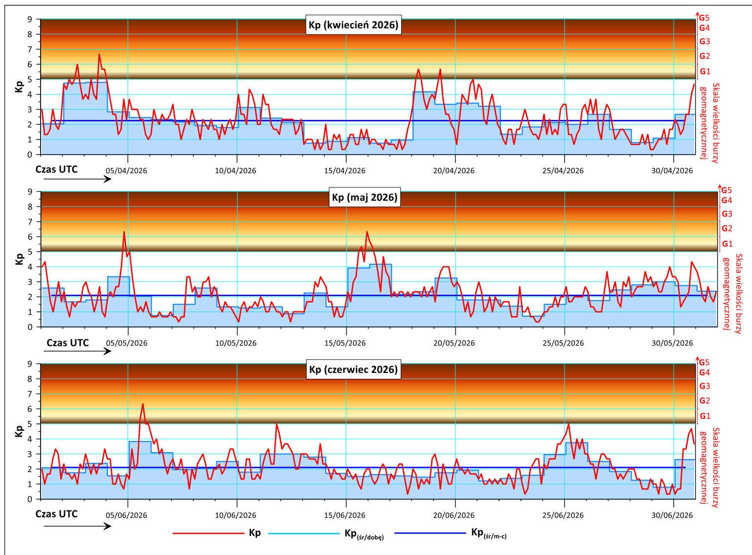
Rys. 3. Zmiany wartości indeksu pogody kosmicznej pod wpływem wiatru słonecznego Kp w kwietniu, maju oraz w czerwcu 2026 r. (oprac. PSG, wg. danych NOAA-SWPC – Centrum Prognoz Pogody Kosmicznej www.swpc.noaa.gov.us ).
