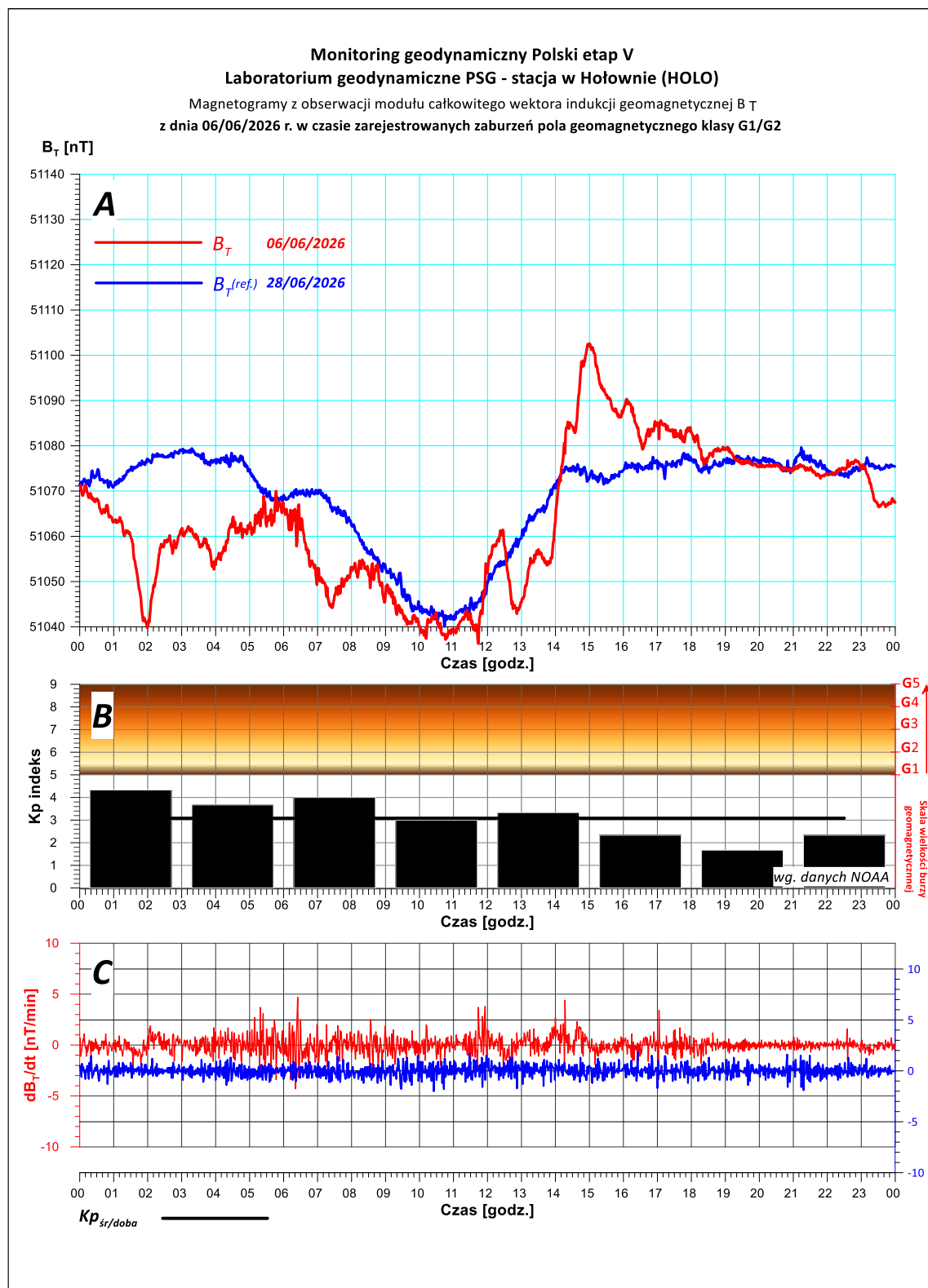
Rys. 5. Magnetogram z monitoringu modułu całkowitego wektora indukcji pola geomagnetycznego zarejestrowany w dniu 06/06/2026 r. na stacji geodynamicznej PSG zlokalizowanej w Hołownie (gm. Podedwórze, pow. parczewski).
