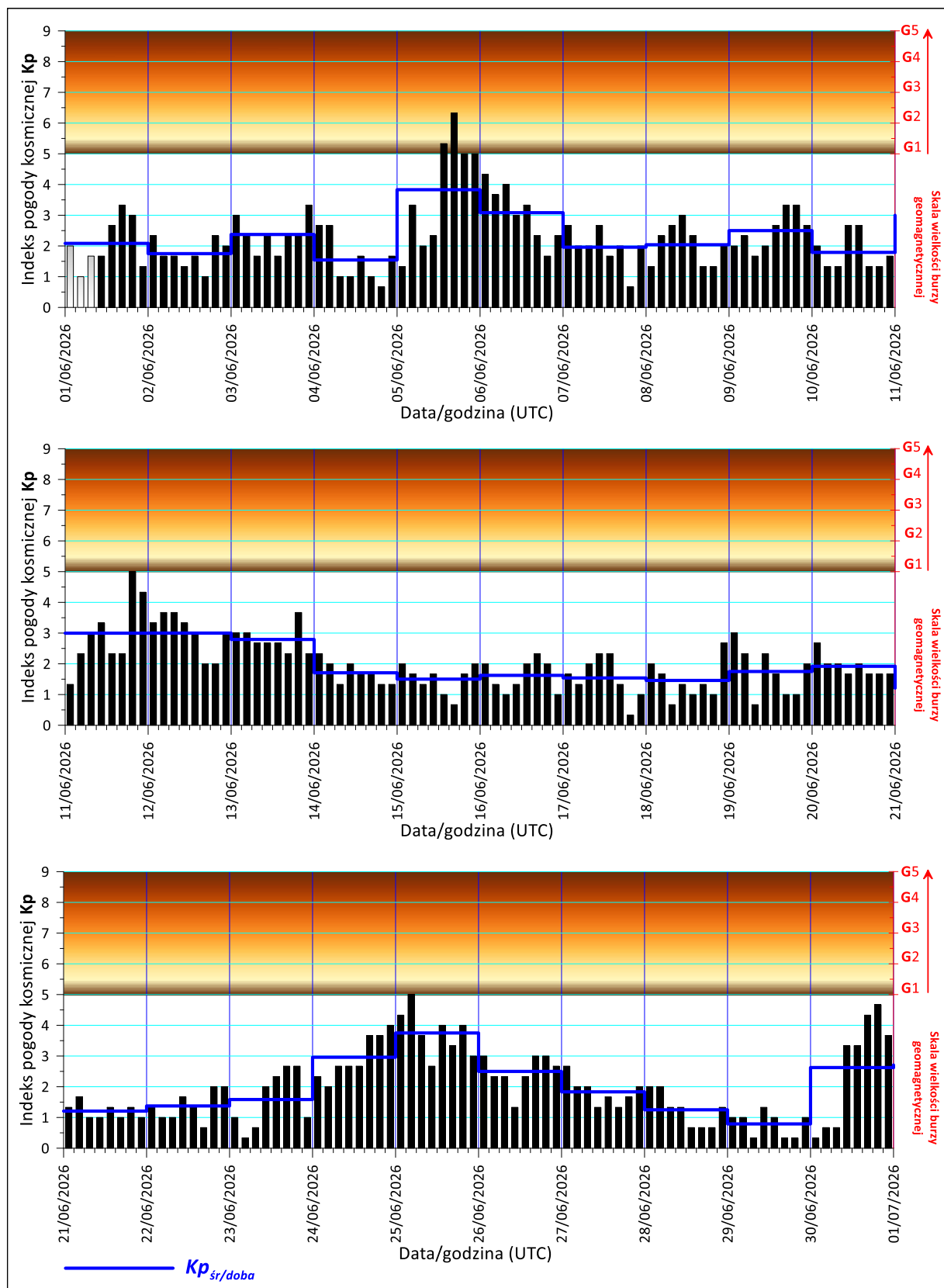
Rys. 2. Zmiany indeksu Kp pogody kosmicznej w miesiącu czerwcu 2026 r. (oprac. PSG, dane wg. NOAA).
