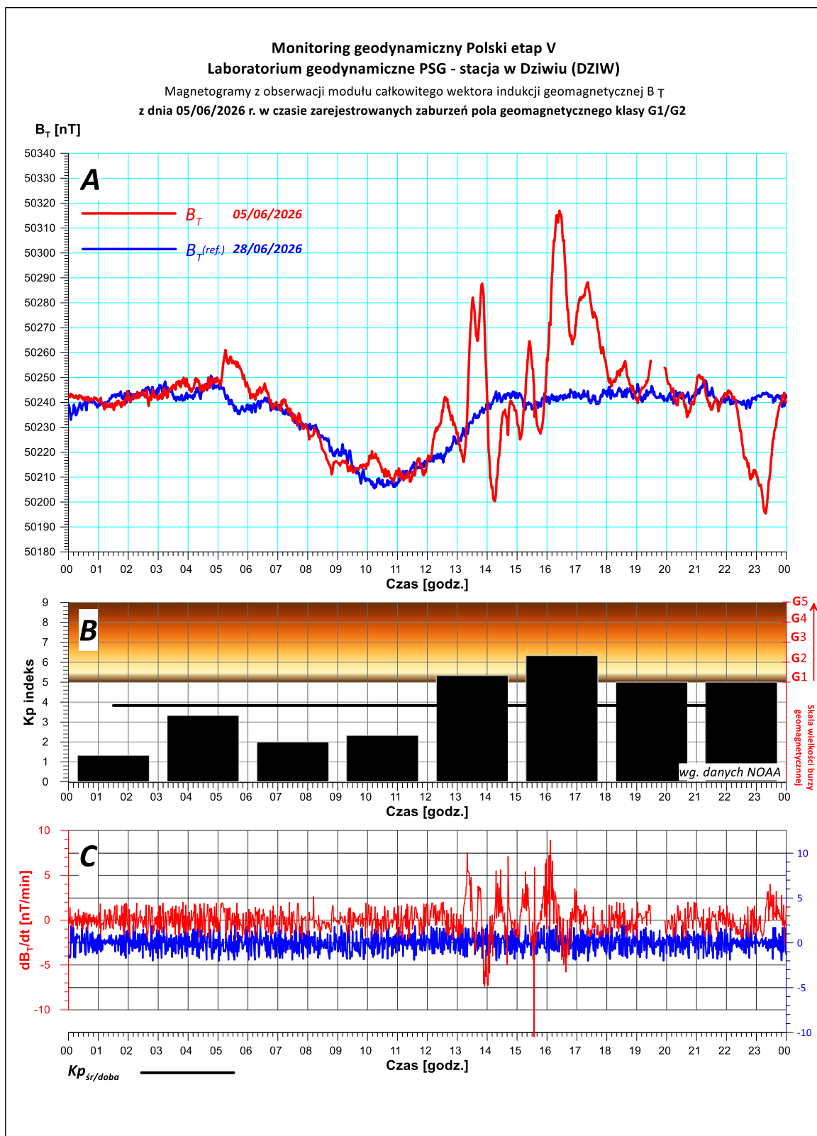
Rys. 6. Magnetogram z monitoringu modułu całkowitego wektora indukcji pola geomagnetycznego zarejestrowany w dniu 05/06/2026 r. na stacji geodynamicznej PSG zlokalizowanej w Dziwiu (gm. Przedecz, pow. kolski).
