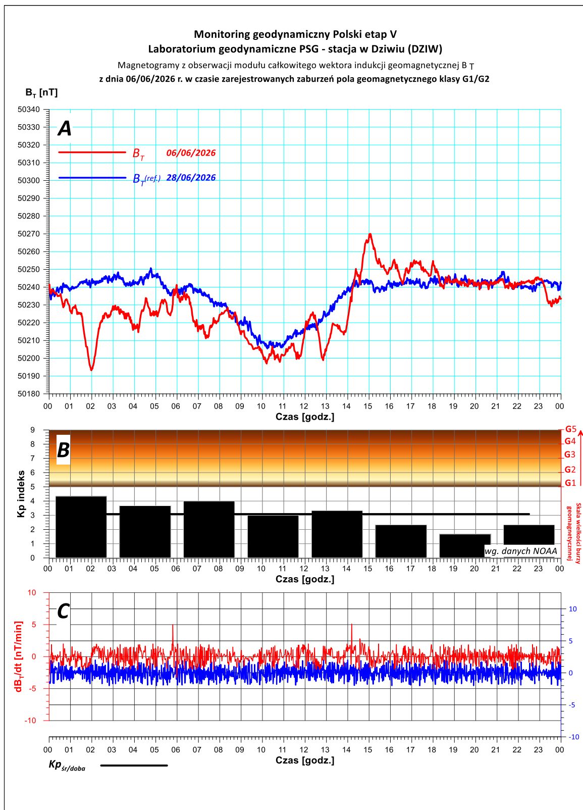
Rys. 7. Magnetogram z monitoringu modułu całkowitego wektora indukcji pola geomagnetycznego zarejestrowany w dniu 06/06/2026 r. na stacji geodynamicznej PSG zlokalizowanej w Dziwiu (gm. Przedecz, pow. kolski).
