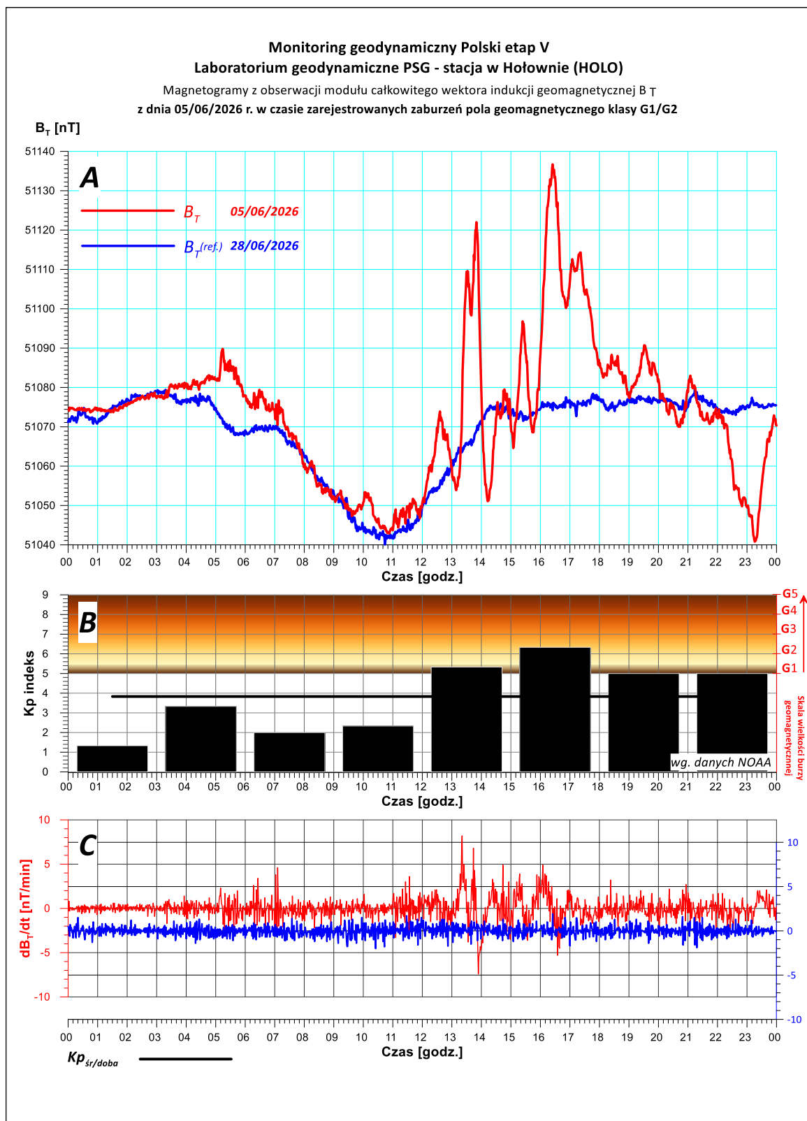
Rys. 4. Magnetogram z monitoringu modułu całkowitego wektora indukcji pola geomagnetycznego zarejestrowany w dniu 05/06/2026 r. na stacji geodynamicznej PSG zlokalizowanej w Hołownie (gm. Podedwórze, pow. parczewski).
