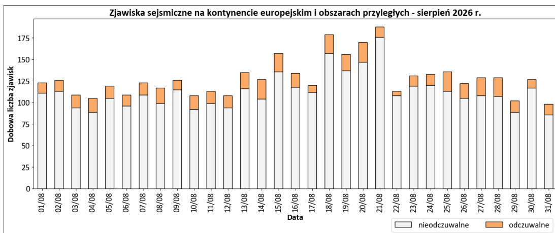
Rys. 5. Sekwencja zjawisk sejsmicznych na kontynencie europejskim w sierpniu 2026 r. – dobową liczebność zjawisk (odczuwalnych i nieodczuwalnych) – oprac. PSG, dane EMSC.
