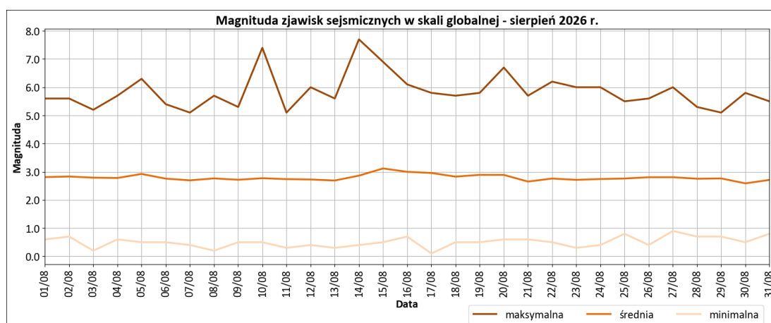
Rys. 8. Sekwencja zjawisk sejsmicznych w skali globalnej w sierpniu 2026 r. – dobową magnitudą: minimalną, średnią i maksymalną – oprac. PSG, dane EMSC.
