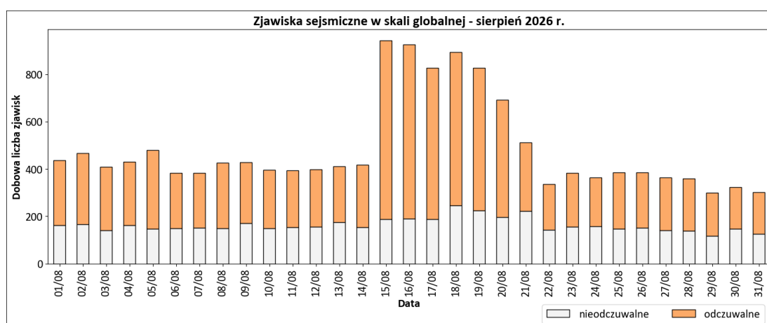
Rys. 7. Sekwencja zjawisk sejsmicznych w skali globalnej w sierpniu 2026 r. – dobową liczebność zjawisk (odczuwalnych i nieodczuwalnych) – oprac. PSG, dane EMSC.
