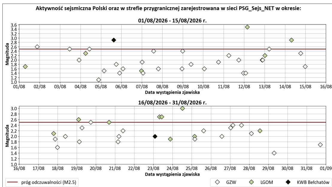
Rys. 2. Sekwencja czasowa zjawisk sejsmicznych zarejestrowanych w sierpniu 2026 r. w sieci PSG_Sejs_NET na terenie Polski oraz w strefie przygranicznej w podziale na regiony, w których zjawiska wystąpiły.
