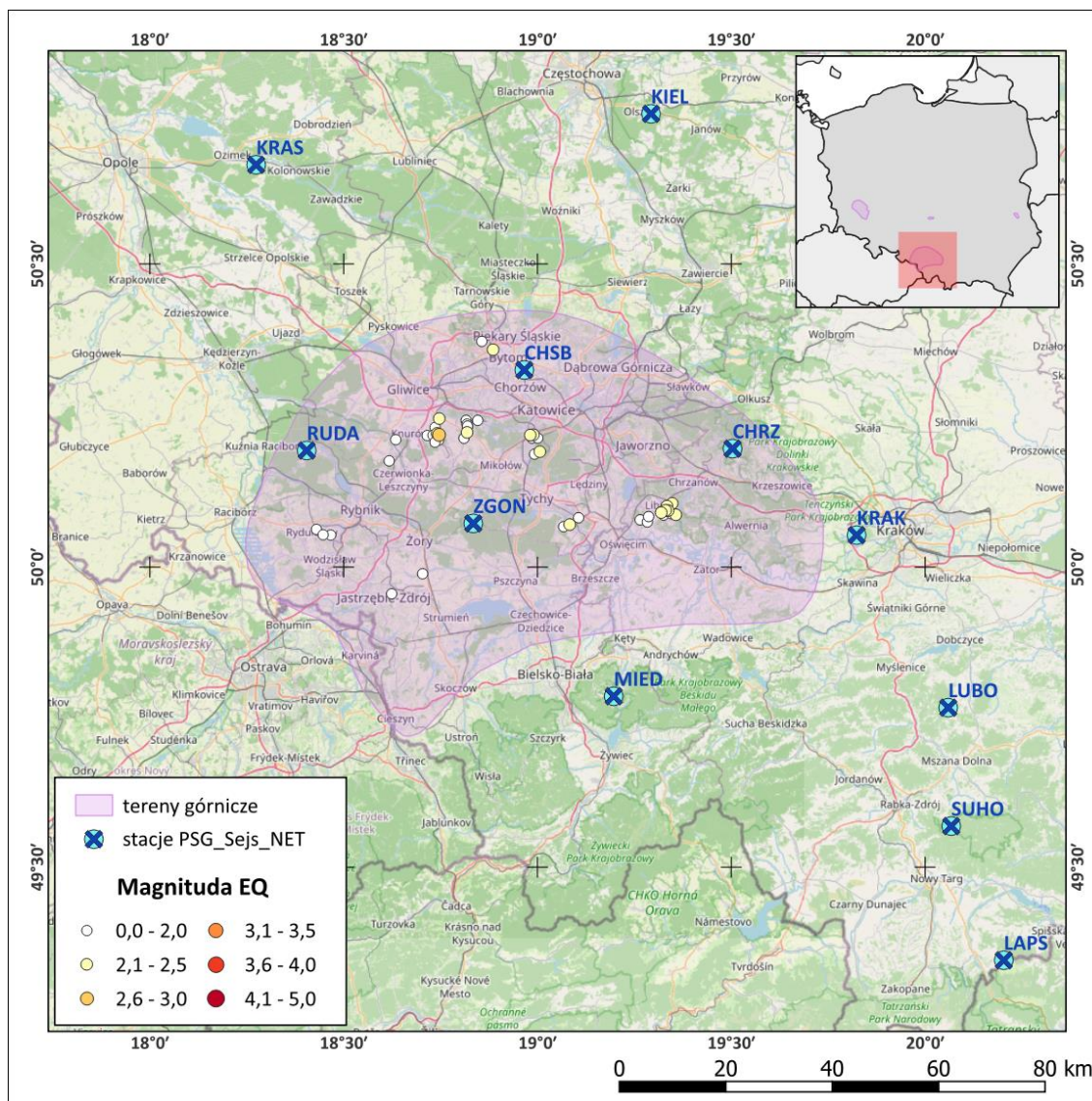
Rys. 3. Lokalizacja epicentrów zjawisk sejsmicznych zarejestrowanych w sieci PSG_Sejs_NET państwowej służby geologicznej na obszarze GZW w sierpniu 2026 r. (dane i oprac. PSG, podkład mapowy: OSM).
