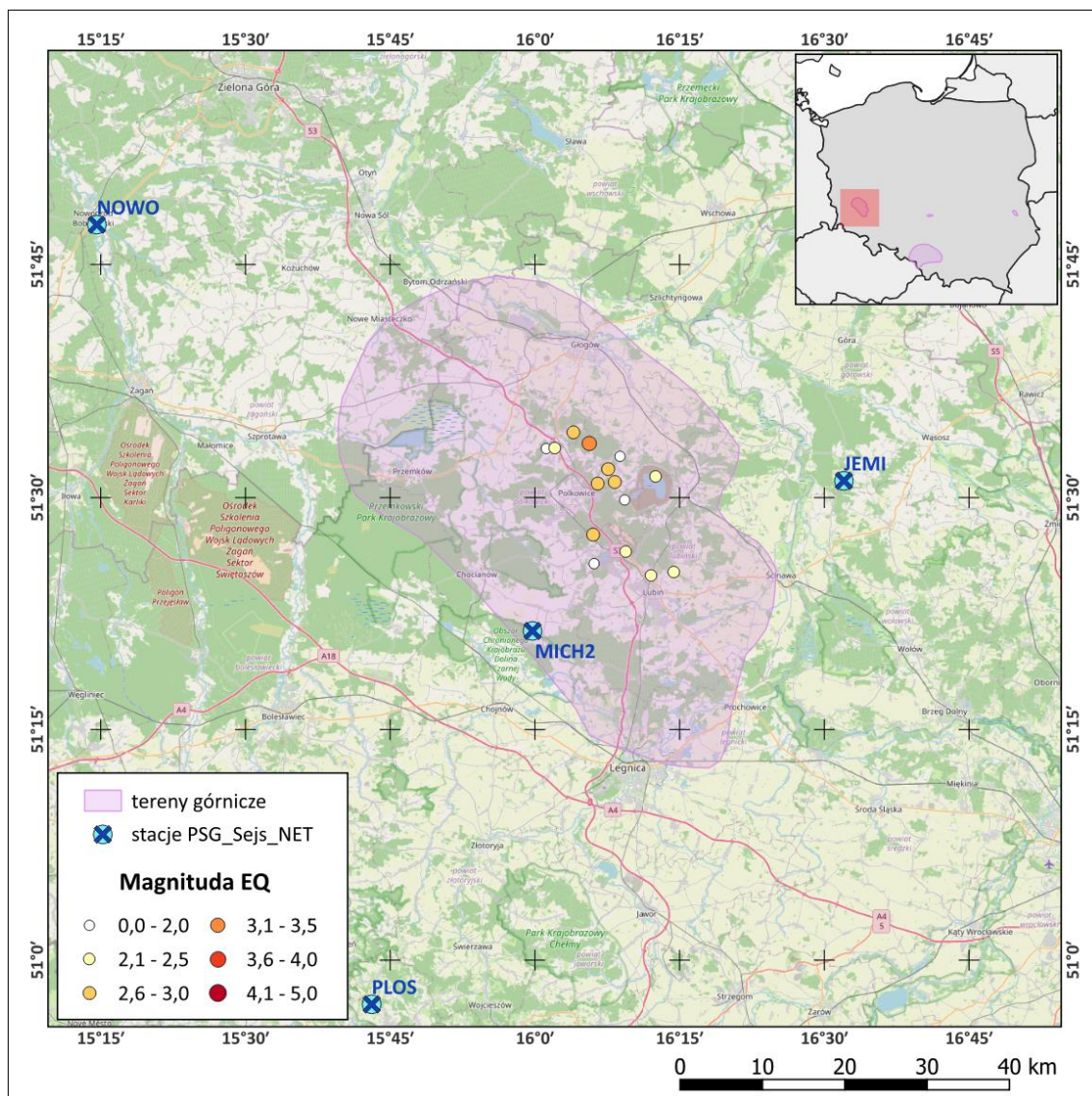
Rys. 4. Lokalizacja epicentrów zjawisk sejsmicznych zarejestrowanych w sieci PSG_Sejs_NET państwowej służby geologicznej na obszarze LGOM w sierpniu 2026 r. (dane i oprac. PSG, podkład mapowy: OSM).
