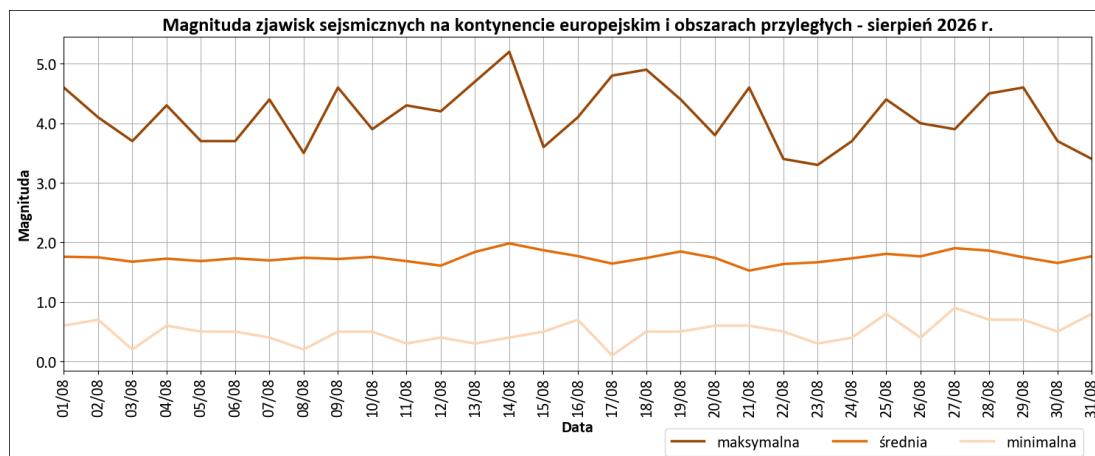
Rys. 6. Sekwencja zjawisk sejsmicznych na kontynencie europejskim w sierpniu 2026 r. – dobowa magnituda: minimalna, średnia i maksymalna – oprac. PSG, dane EMSC.
