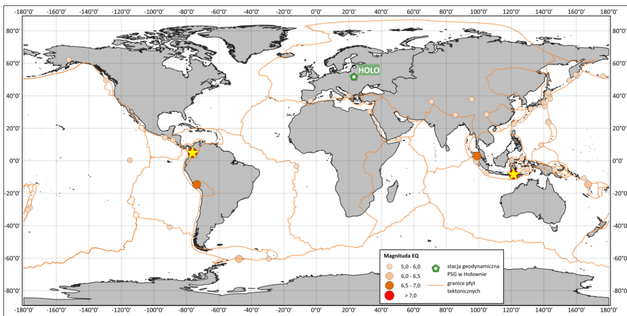
Rys. 12. Lokalizacja epicentrów wybranych zjawisk sejsmicznych widocznych w zapisie parametrów monitoringu grawimetrycznego w sierpniu 2026 r. na stacji geodynamicznej PSG w Hołownie (HOLO).
