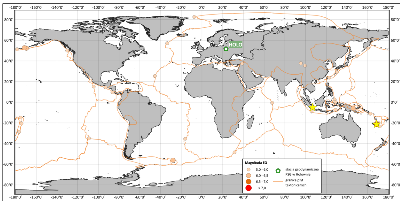
Rys. 12. Lokalizacja epicentrów wybranych zjawisk sejsmicznych widocznych w zapisie parametrów monitoringu grawimetrycznego we wrześniu 2026 r. na stacji geodynamicznej PSG w Hołownie (HOLO).
