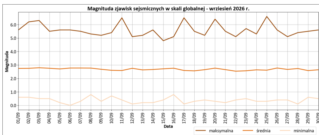
Rys. 8. Sekwencja zjawisk sejsmicznych w skali globalnej we wrześniu 2026 r. – dobowa magnituda: minimalna, średnia i maksymalna – oprac. PSG, dane EMSC.
