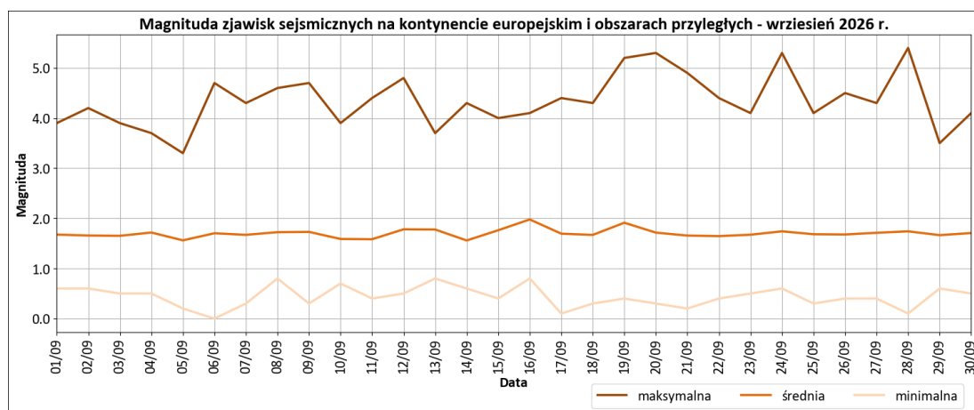
Rys. 6. Sekwencja zjawisk sejsmicznych na kontynencie europejskim we wrześniu 2026 r. – dobowa magnituda: minimalna, średnia i maksymalna – oprac. PSG, dane EMSC.
