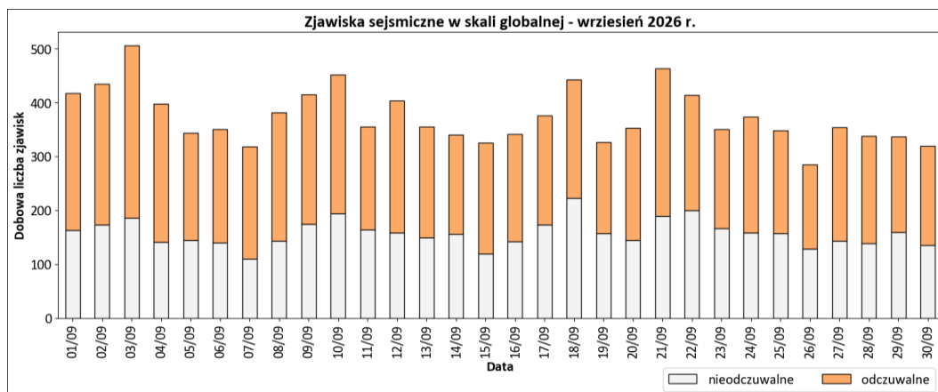
Rys. 7. Sekwencja zjawisk sejsmicznych w skali globalnej we wrześniu 2026 r. – dobowa liczebność zjawisk (odczuwalnych i nieodczuwalnych) – oprac. PSG, dane EMSC.
