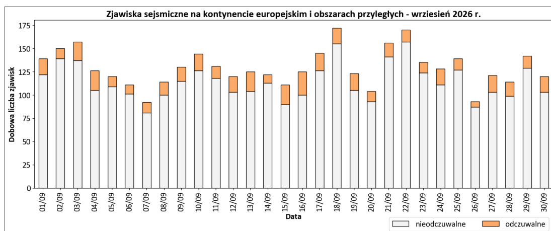
Rys. 5. Sekwencja zjawisk sejsmicznych na kontynencie europejskim we wrześniu 2026 r. – dobowa liczebność zjawisk (odczuwalnych i nieodczuwalnych) – oprac. PSG, dane EMSC.
