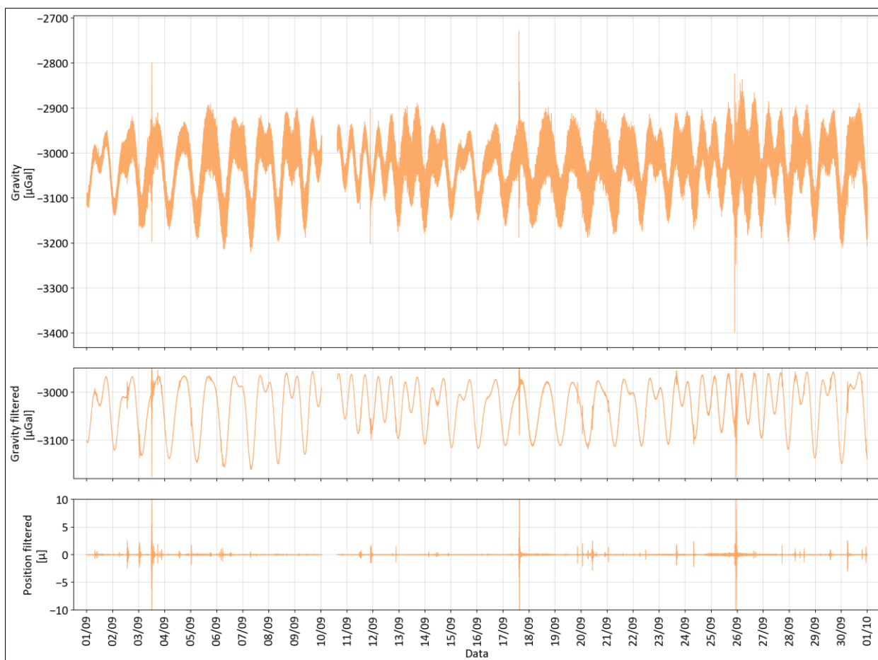
Rys. 9. Zmiany pionowej składowej siły ciężkości g zarejestrowane w okresie od 01/09/2026 do 30/09/2026 r. w laboratorium geodynamicznym PSG w Hołownie; zmiany składowej pionowej przyspieszenia siły ciężkości (górny wykres), zmiany składowej pionowej przyspieszenia siły ciężkości po filtracji dolnoprzepustowej (środkowy wykres), podwójne przecałowane, zredukowane zmiany składowej pionowej przyspieszenia siły ciężkości po filtracji dolnoprzepustowej (dolny wykres).
