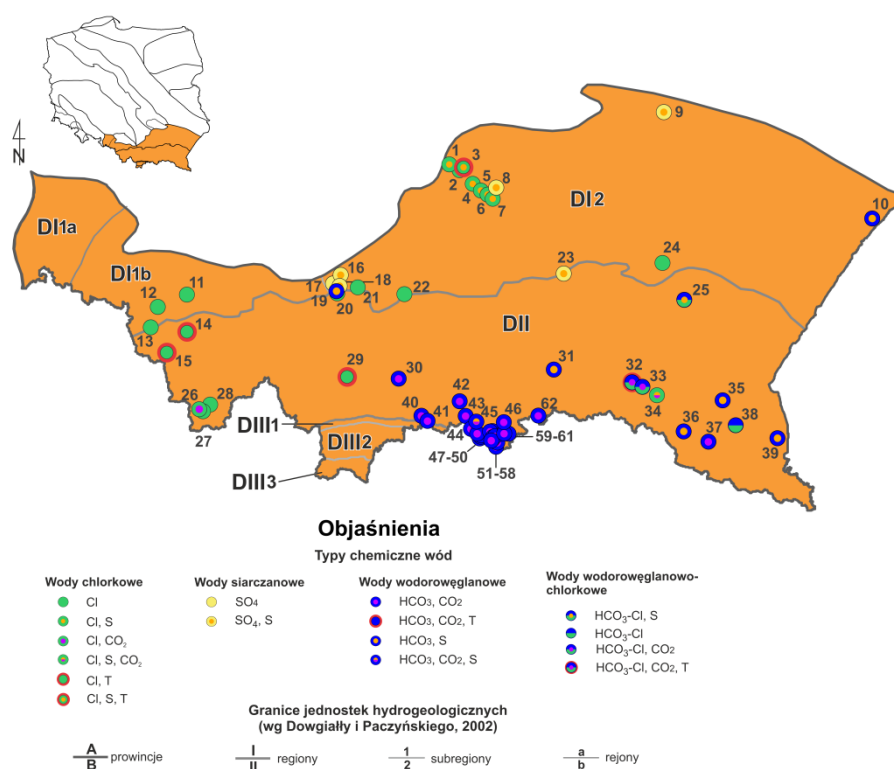
Fig. 3.4. Lokalizacja złóż wód leczniczych i solanek w obrębie prowincji karpackiej – nazwy złóż w tabeli 3.2 (regionalizacja wg Dowgiałły, Paczyńskiego, 2002)
