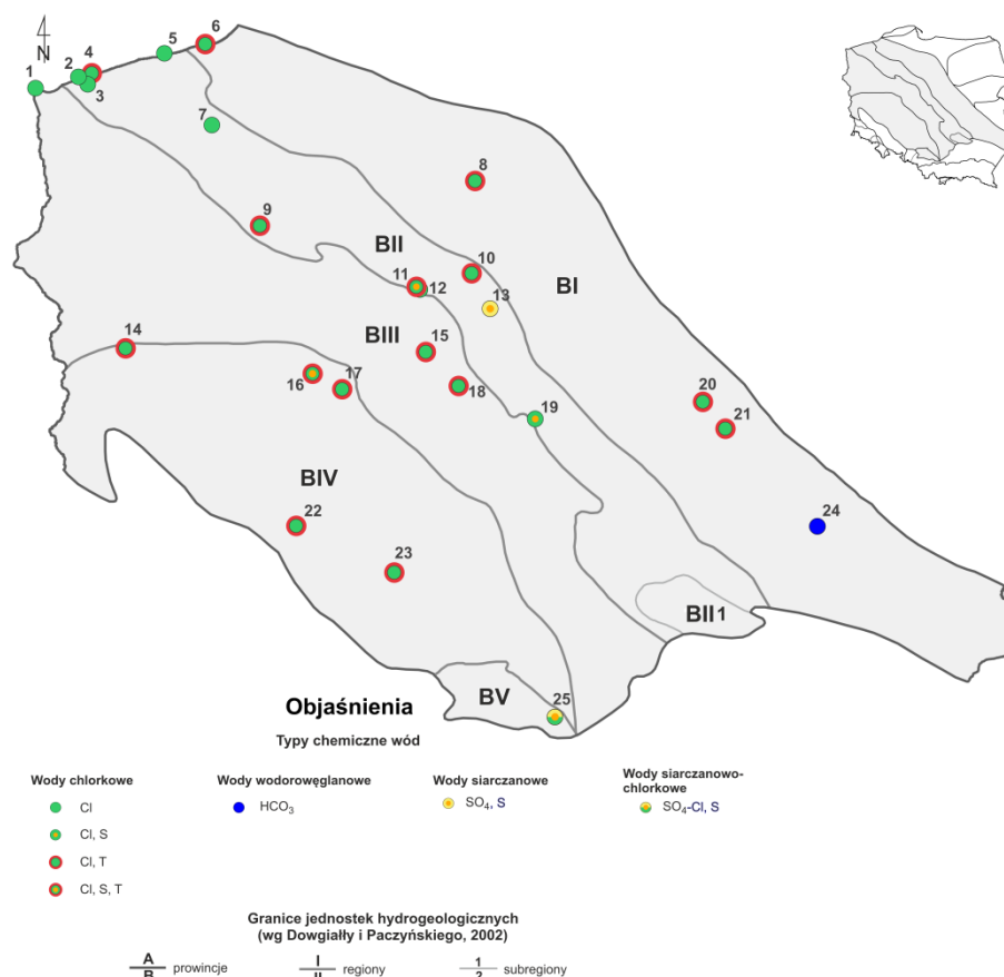
Fig. 3.2. Lokalizacja źródeł wód leczniczych w obrębie platformy paleozoicznej – nazwy źródeł w tabeli 3.2 (regionalizacja wg Dowgiałły, Paczyńskiego, 2002)
