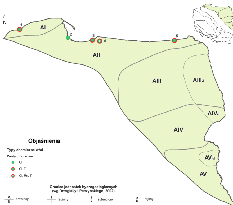
Fig. 3.1. Lokalizacja złóż wód leczniczych w obrębie platformy prekambryjskiej – nazwy złóż w tabeli 3.2 (regionalizacja wg Dowgiałły, Paczyńskiego, 2002)
