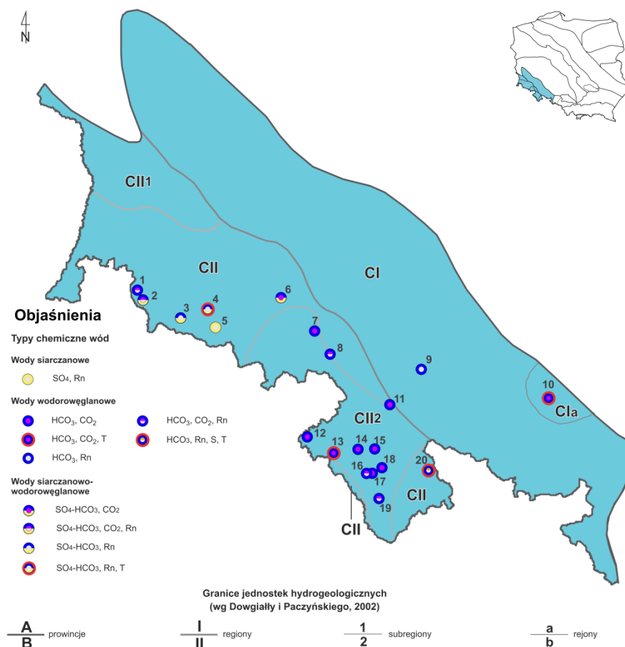
Fig. 3.3. Lokalizacja źródeł wód leczniczych w obrębie prowincji sudeckiej – nazwy źródeł w tabeli 3.2 (regionalizacja wg Dowgiałły, Paczyńskiego, 2002)
