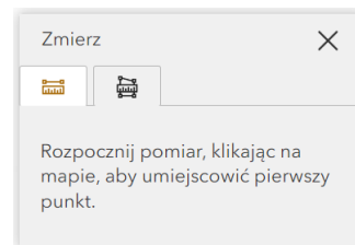
Rys. 6. Widżet Zmierz
