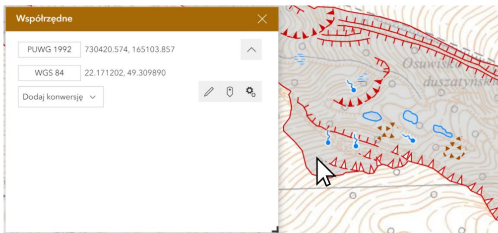
Rys. 39. Widżet współrzędne
