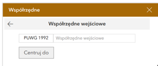
Rys. 40. Współrzędne wejściowe
