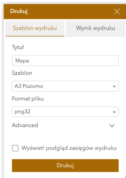
Rys. 19. Widżet Drukuj
