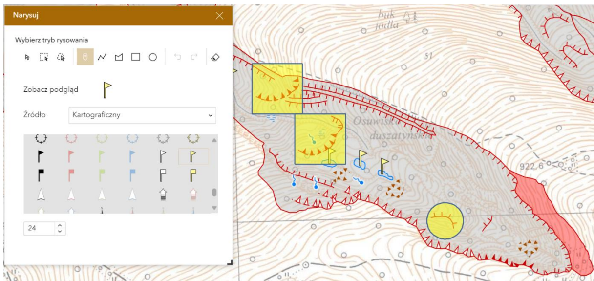
Rys. 42. Widżet Narysuj
