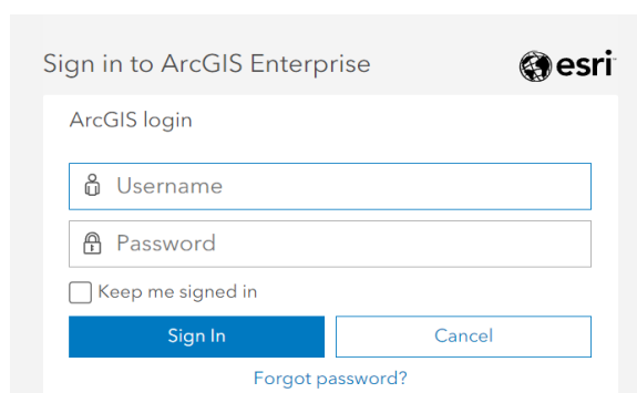
Rys. 2. Okno logowania
