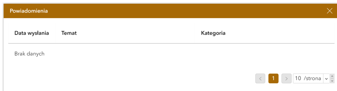
Rys. 11. Widżet powiadomienia
