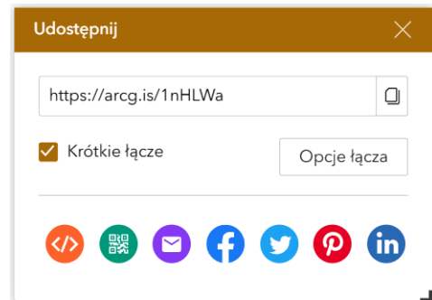
Rys. 9. Widżet Udostępnij
