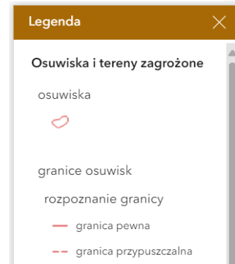
Rys. 18. Widżet Legenda
