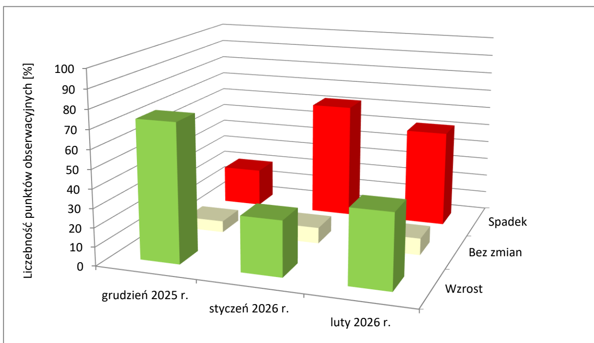
Ryc. 2. Rozkład zmian położenia swobodnego zwierciadła wód podziemnych w okresie od grudnia 2025 r. do lutego 2026 r.
