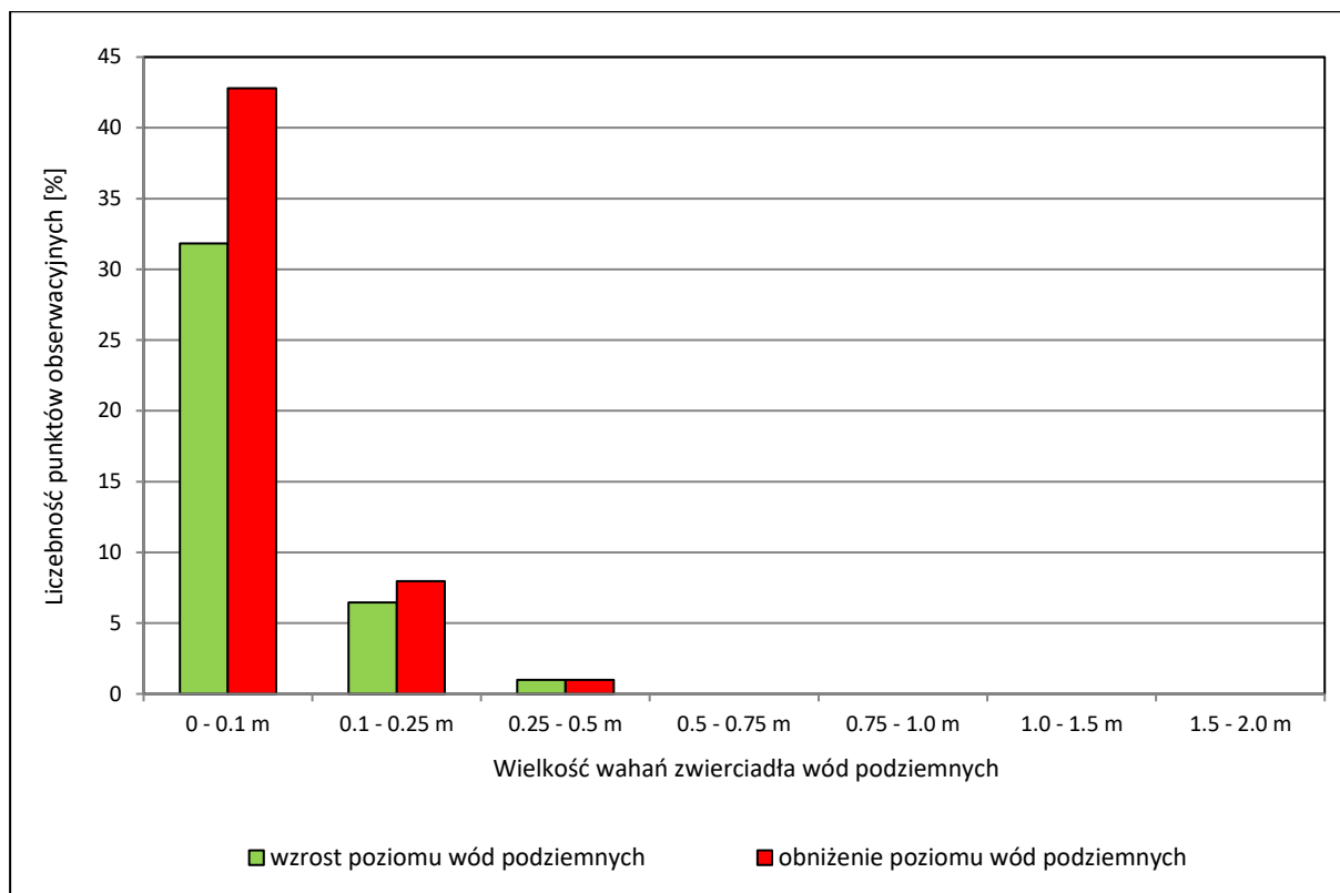
Ryc. 3. Rozkład wielkości wahań swobodnego zwierciadła wód podziemnych w lutym 2026 r.
