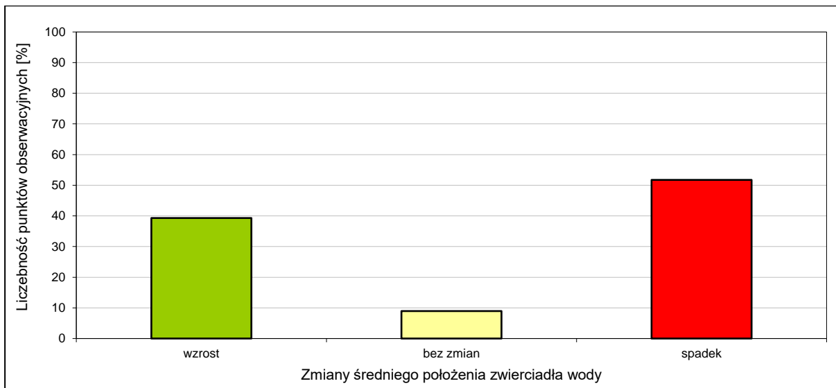
Ryc. 1. Rozkład zmian położenia swobodnego zwierciadła wód podziemnych w lutym 2026 r. w stosunku do stanu zaobserwowanego w poprzednim miesiącu (na podstawie średnich wartości miesięcznych)
