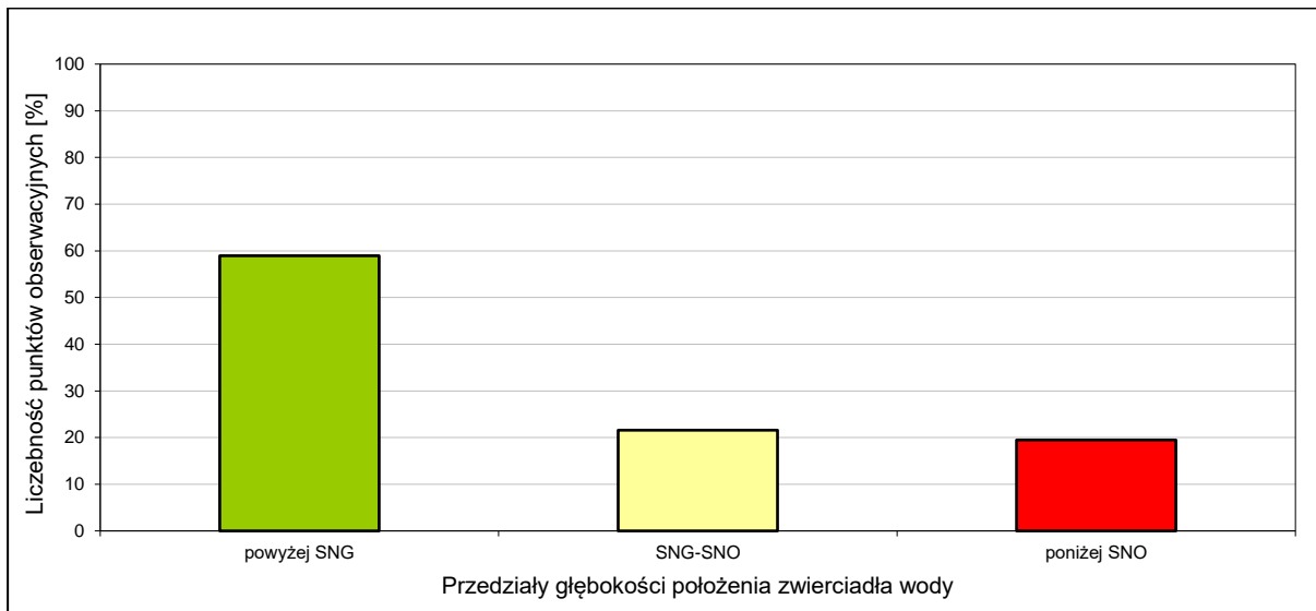
Ryc. 7 Rozkład średnich wartości położenia zwierciadła wód podziemnych w lutym 2026 r. w stosunku do wyznaczonych poziomów odniesienia (SNG, SNO)
