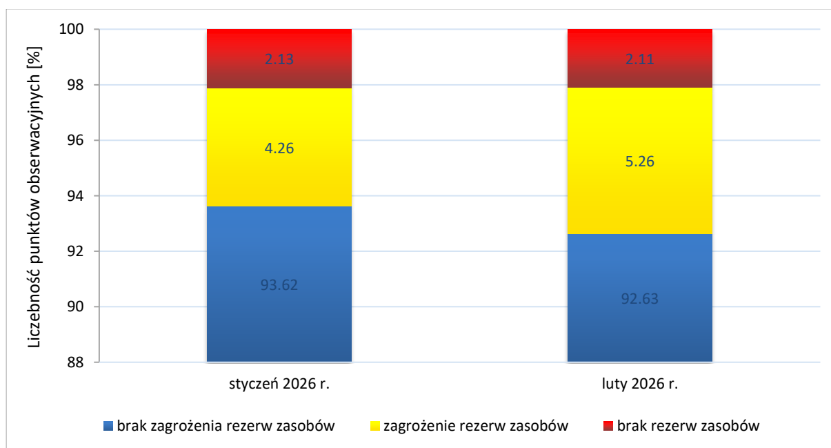
Ryc. 5. Liczebność punktów objętych analizą w przyjętych klasach stanu rezerw zmiennych zasobów wód podziemnych na terenie kraju w styczniu i lutym 2026 r.
