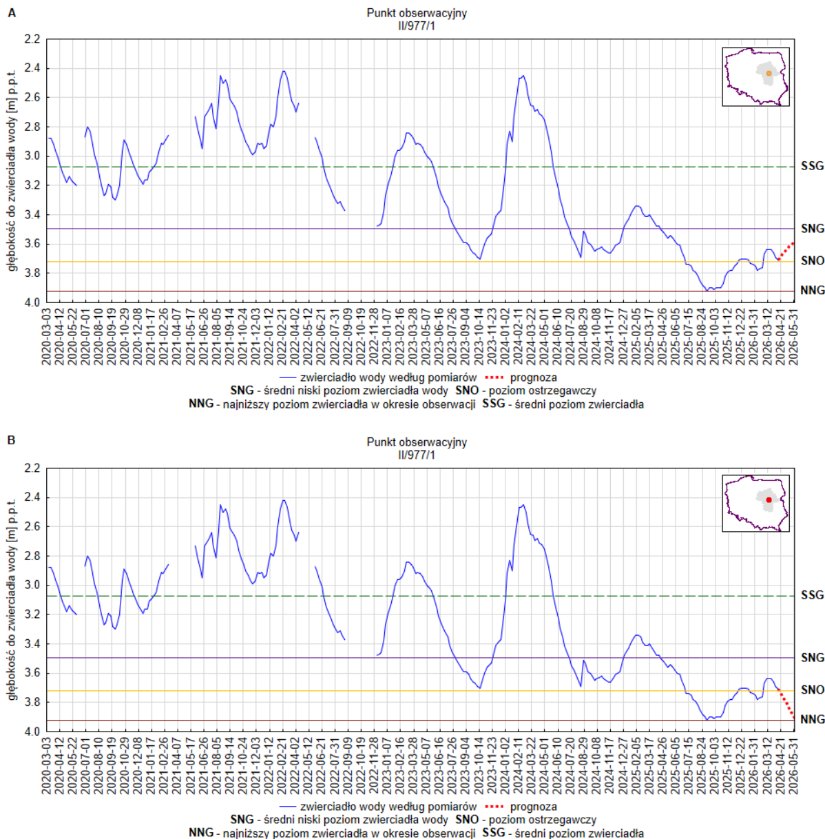
Rys. 10. Prognoza dotycząca stanu wód o zwiędziadle swobodnym (gruntowych) na okres 01.05.2026–31.05.2026 r. – stacja hydrogeologiczna nr II/977/1 w miejscowości Okuniew (woj. mazowieckie). A – prognoza przy założeniu scenariusza A; B – prognoza przy założeniu scenariusza B
