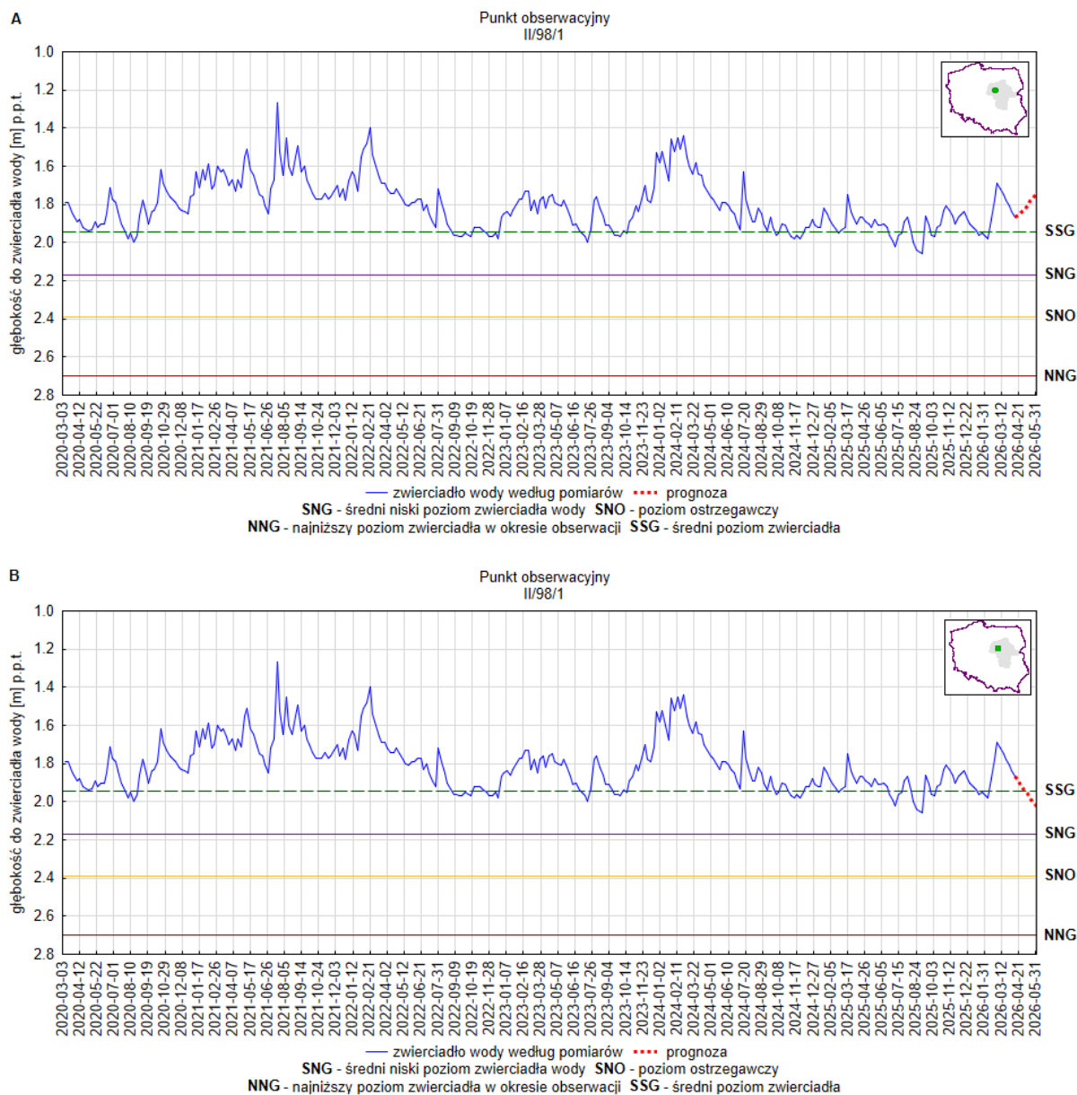
Rys. 11. Prognoza dotycząca stanu wód o zwierciadle swobodnym (gruntowych) na okres 01.05.2026–31.05.2026 r. – stacja hydrogeologiczna nr II/98/1 w miejscowości Płońsk (woj. mazowieckie). A – prognoza przy założeniu scenariusza A; B – prognoza przy założeniu scenariusza B
