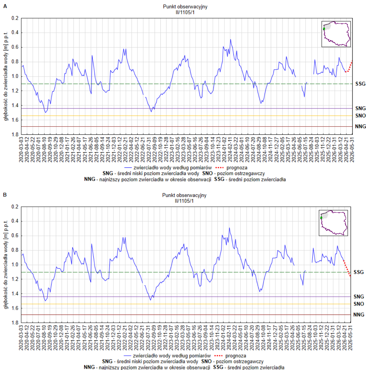
Rys. 24. Prognoza dotycząca stanu wód o zwierciadle swobodnym (gruntowych) na okres 01.05.2026–31.05.2026 r. – stacja hydrogeologiczna nr II/1105/1 w miejscowości Ognica (woj. zachodniopomorskie). A – prognoza przy założeniu scenariusza A; B – prognoza przy założeniu scenariusza B
