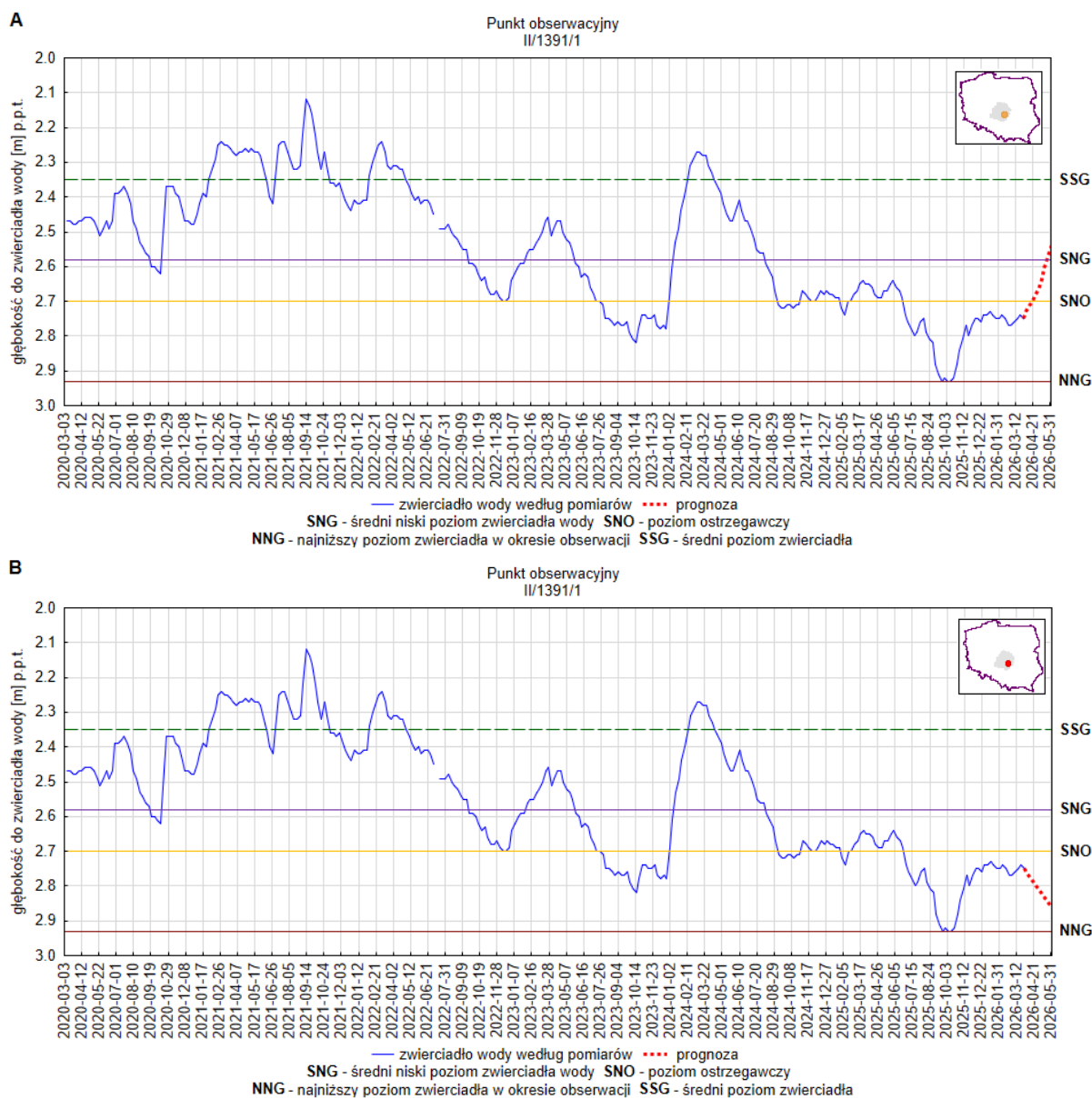
Rys. 7. Prognoza dotycząca stanu wód o zwierciadle swobodnym (gruntowych) na okres 01.05.2026–31.05.2026 r. – stacja hydrogeologiczna nr II/1391/1 w miejscowości Sulejów (woj. łódzkie). A – prognoza przy założeniu scenariusza A; B – prognoza przy założeniu scenariusza B
