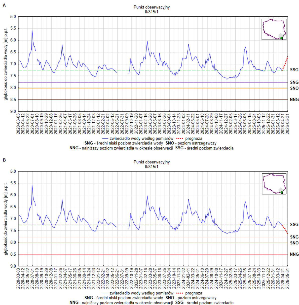
Rys. 13. Prognoza dotycząca stanu wód o zwierciadle swobodnym (gruntowych) na okres 01.05.2026–31.05.2026 r. – stacja hydrogeologiczna nr II/815/1 w miejscowości Lesko (woj. podkarpackie). A – prognoza przy założeniu scenariusza A; B – prognoza przy założeniu scenariusza B
