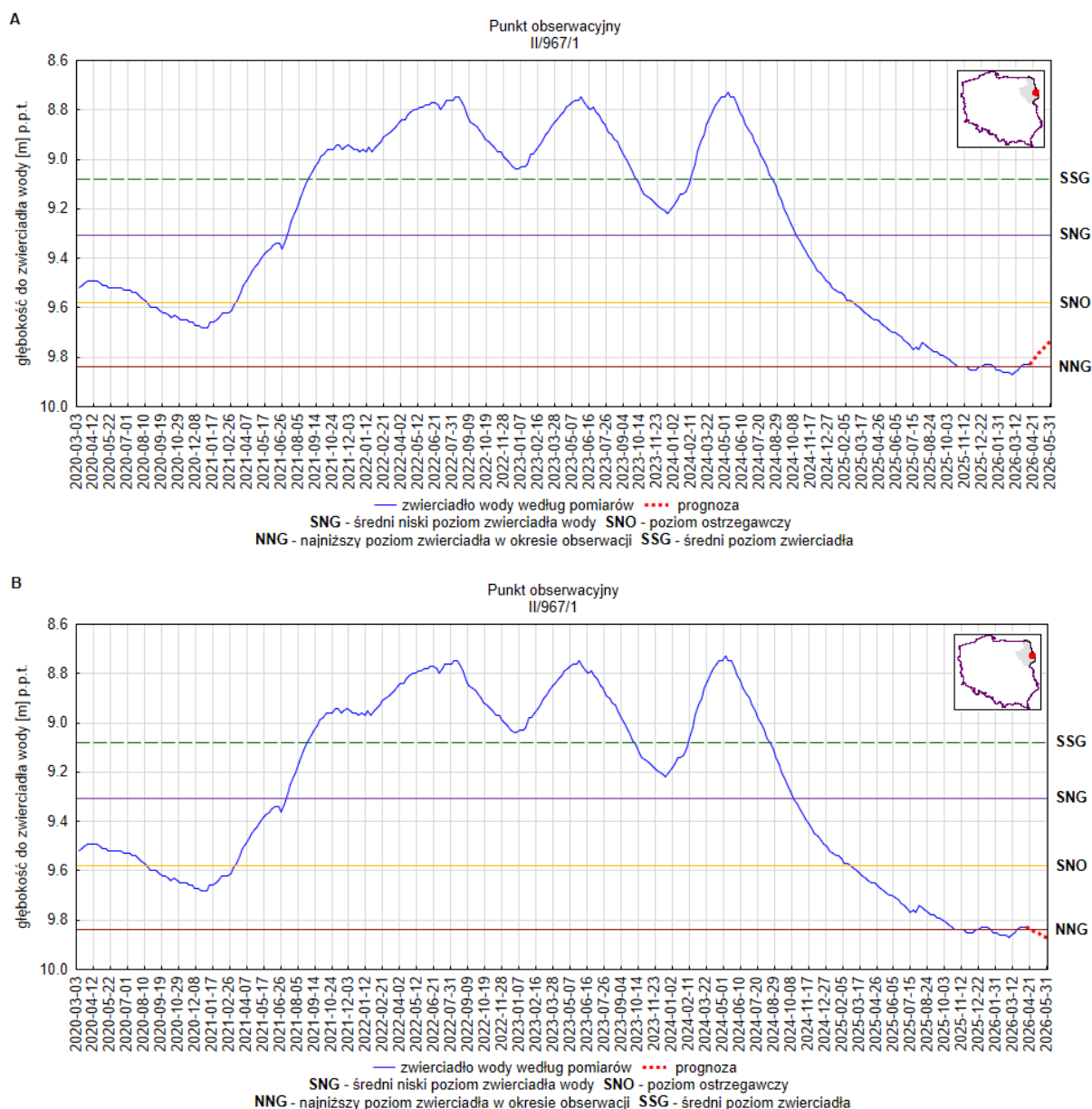
Rys. 14. Prognoza dotycząca stanu wód o zwierciadle swobodnym (gruntowych) na okres 01.05.2026–31.05.2026 r.- stacja hydrogeologiczna nr II/967/1 w miejscowości Waliły (woj. podlaskie). A – prognoza przy założeniu scenariusza A; B – prognoza przy założeniu scenariusza B
