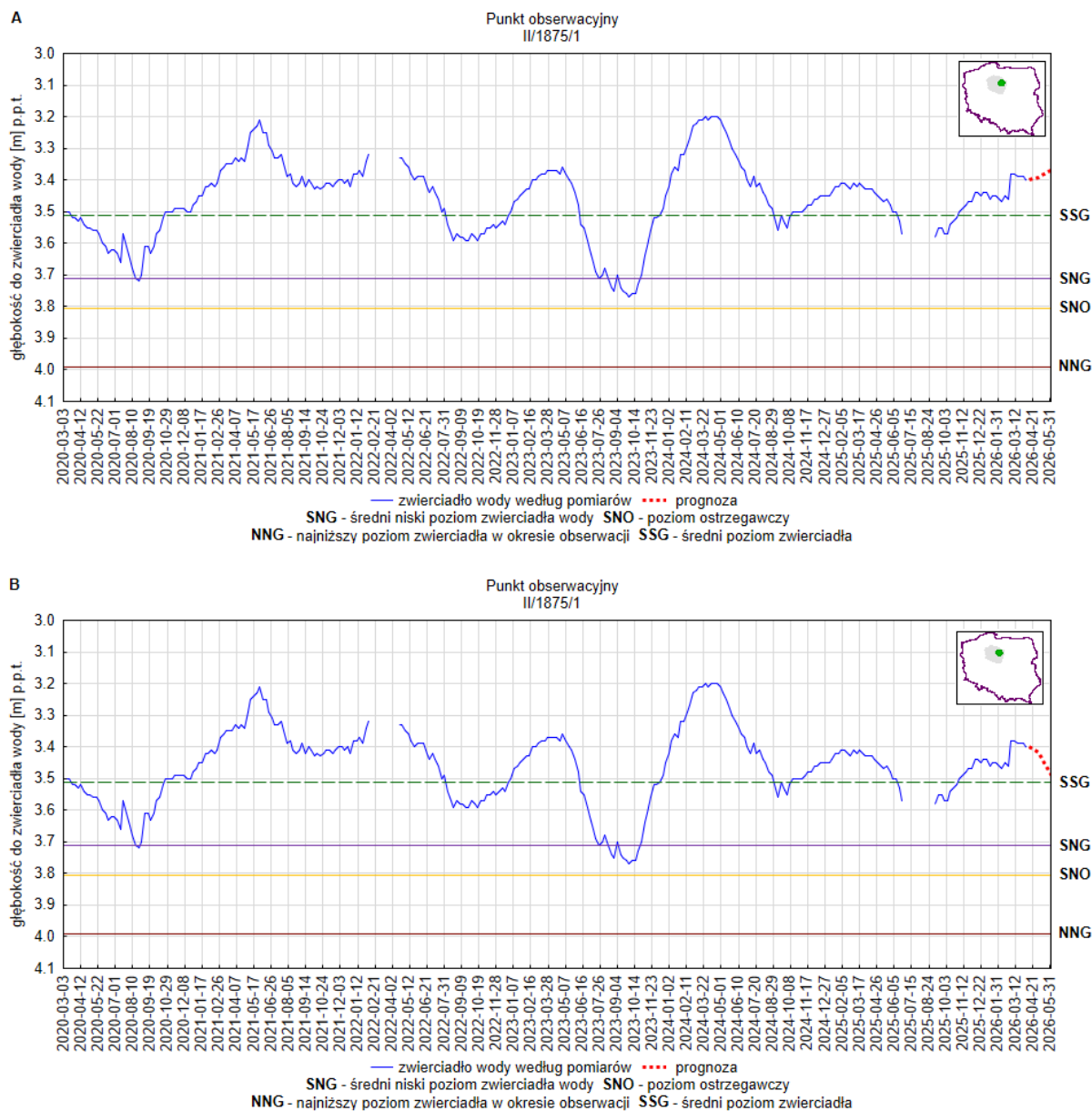
Rys. 3. Prognoza dotycząca stanu wód o zwierciadle swobodnym (gruntowych) na okres 01.05.2026–31.05.2026 r. – stacja hydrogeologiczna nr II/1875/1 w miejscowości Mokry Las (woj. kujawsko-pomorskie). A – prognoza przy założeniu scenariusza A; B – prognoza przy założeniu scenariusza B
