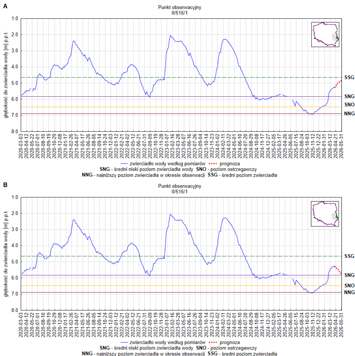
Rys. 5. Prognoza dotycząca stanu wód o zwierciadle swobodnym (gruntowych) na okres 01.05.2026–31.05.2026 r. – stacja hydrogeologiczna nr II/516/1 w miejscowości Żmudź (woj. lubelskie). A – prognoza przy założeniu scenariusza A; B – prognoza przy założeniu scenariusza B
