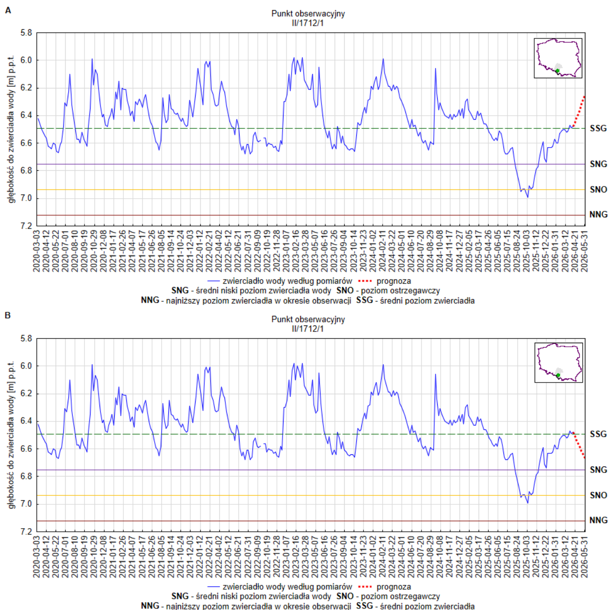
Rys. 18 Prognoza dotycząca stanu wód o zwierciadle swobodnym (gruntowych) na okres 01.05.2026–31.05.2026 r. – stacja hydrogeologiczna nr II/1712/1 w miejscowości Piasek (woj. śląskie). A – prognoza przy założeniu scenariusza A; B - prognoza przy założeniu scenariusza B
