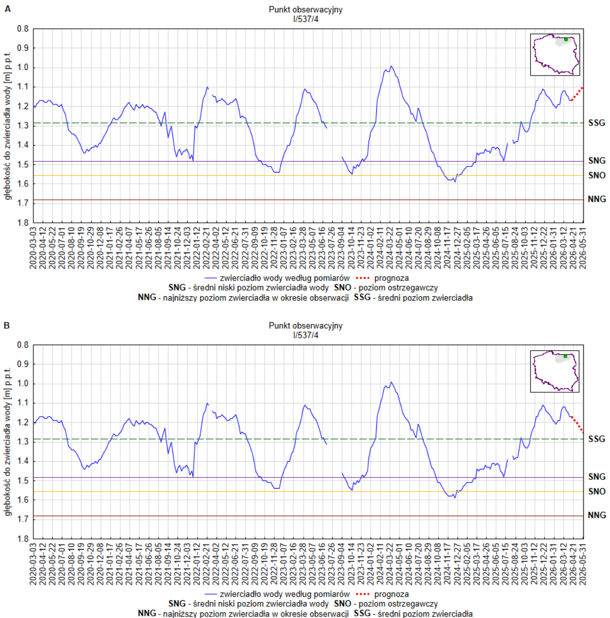
Rys. 21. Prognoza dotycząca stanu wód o zwierciadle swobodnym (gruntowych) na okres 01.05.2026–31.05.2026 r. – stacja hydrogeologiczna nr I/537/4 w miejscowości Doba (woj. warmińsko-mazurskie). A – prognoza przy założeniu scenariusza A; B – prognoza przy założeniu scenariusza B
