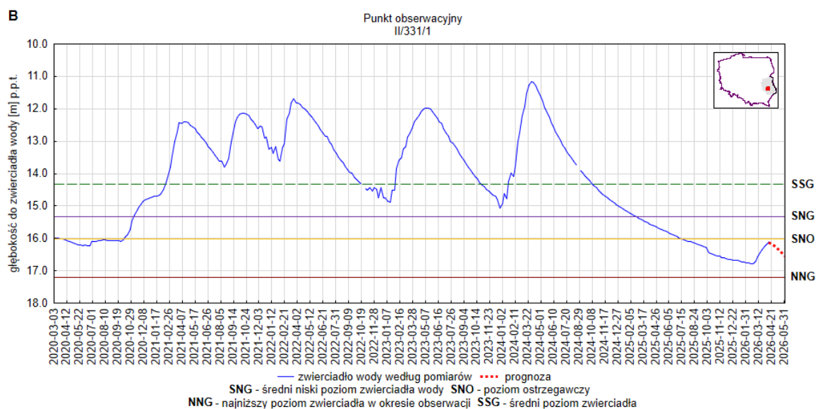
Rys. 4. Prognoza dotycząca stanu wód o zwierciadle swobodnym (gruntowych) na okres 01.05.2026–31.05.2026 r. – stacja hydrogeologiczna nr II/331/1 w miejscowości Giełczew Doły (woj. lubelskie). A – prognoza przy założeniu scenariusza A; B – prognoza przy założeniu scenariusza B
