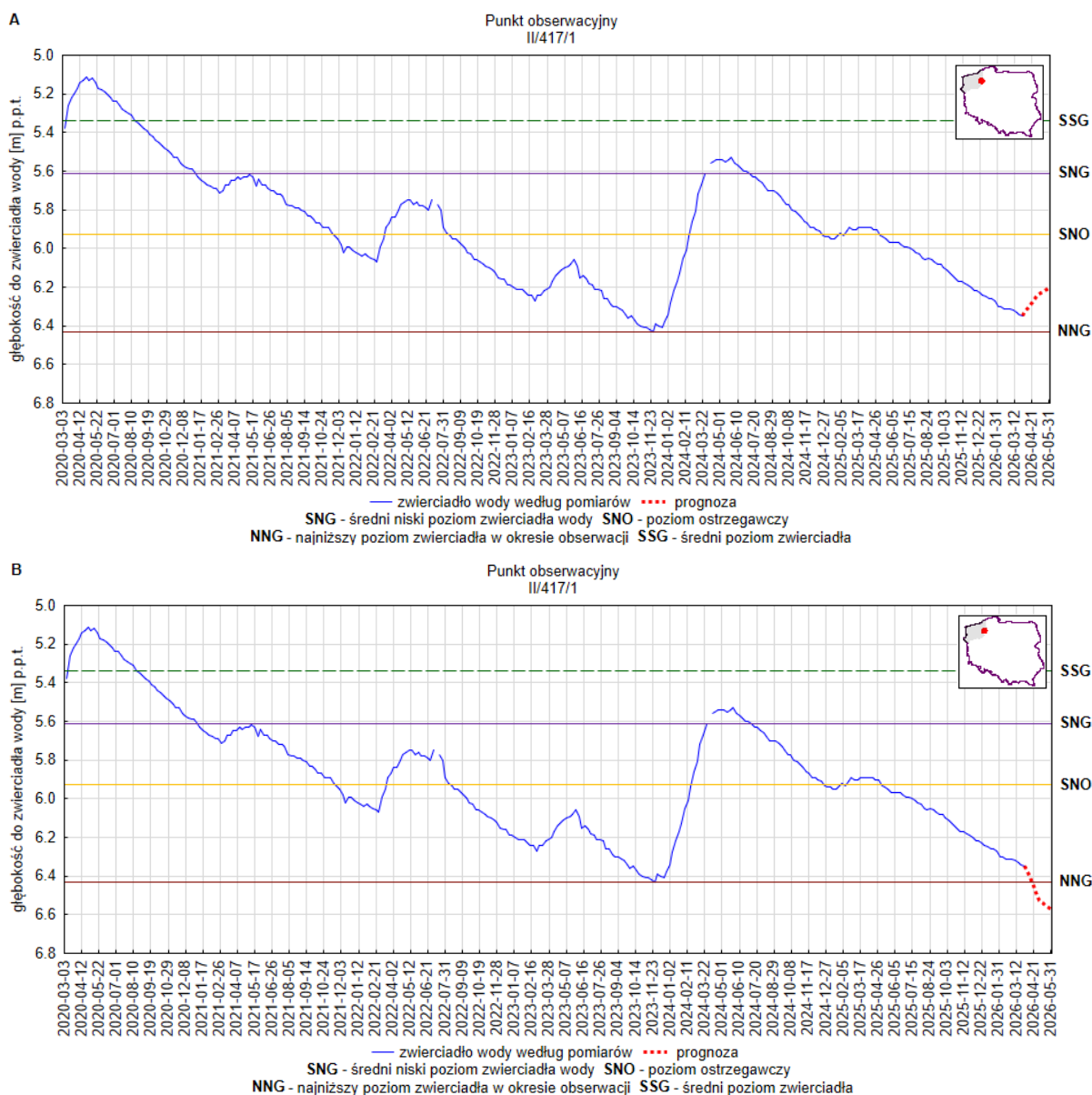
Rys. 23. Prognoza dotycząca stanu wód o zwierciadle swobodnym (gruntowych) na okres 01.05.2026–31.05.2026 r. – stacja hydrogeologiczna nr II/417/1 w miejscowości Turowo (woj. zachodniopomorskie). A – prognoza przy założeniu scenariusza A; B – prognoza przy założeniu scenariusza B
