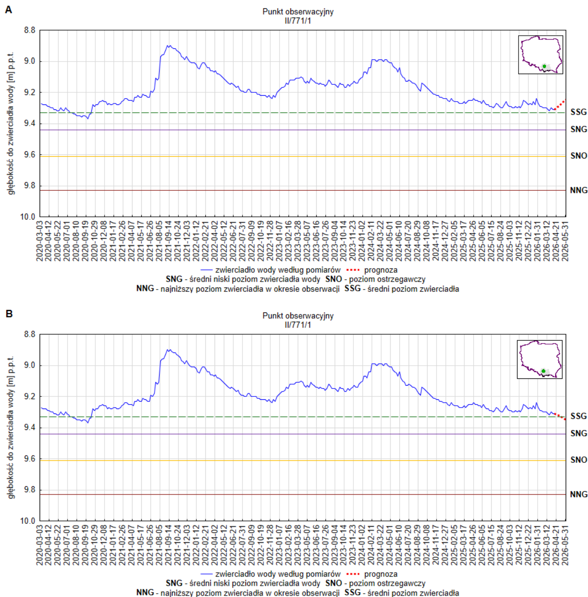
Rys. 9. Prognoza dotycząca stanu wód o zwierniadle swobodnym (gruntowych) na okres 01.05.2026–31.05.2026 r. – stacja hydrogeologiczna nr II/771/1 w miejscowości Kraków (woj. małopolskie). A – prognoza przy założeniu scenariusza A; B – prognoza przy założeniu scenariusza B
