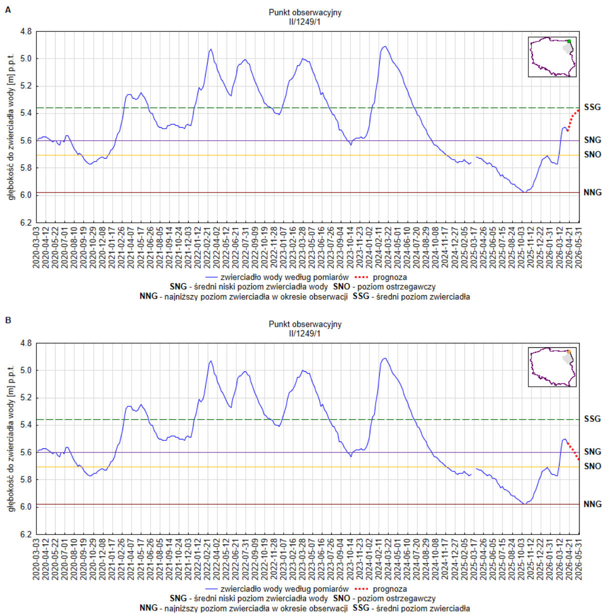
Rys. 15. Prognoza dotycząca stanu wód o zwierciadle swobodnym (gruntowych) na okres 01.05.2026–31.05.2026 r.- stacja hydrogeologiczna nr II/1249/1 w miejscowości Boksze Stare (woj. podlaskie). A – prognoza przy założeniu scenariusza A; B – prognoza przy założeniu scenariusza B
