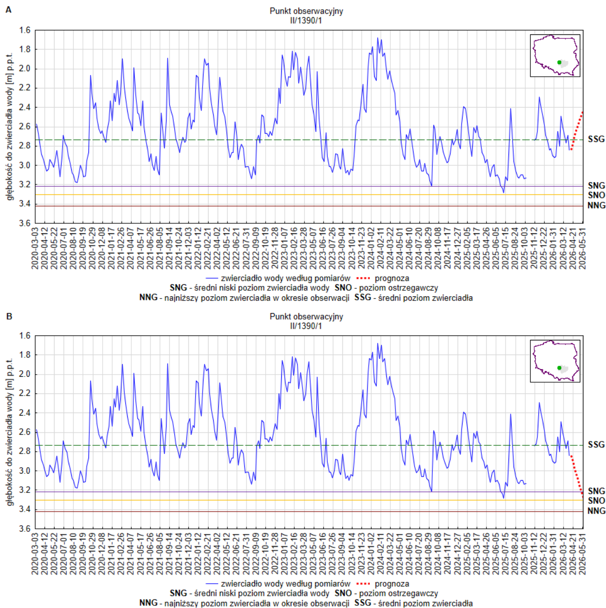
Rys. 20. Prognoza dotycząca stanu wód o zwierciadle swobodnym (gruntowych) na okres 01.05.2026–31.05.2026 r. – stacja hydrogeologiczna nr II/1390/1 w miejscowości Januszewice (woj. świętokrzyskie). A – prognoza przy założeniu scenariusza A; B – prognoza przy założeniu scenariusza B
