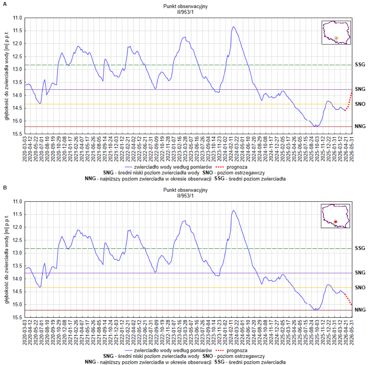
Rys. 17. Prognoza dotycząca stanu wód o zwierciadle swobodnym (gruntowych) na okres 01.05.2026–31.05.2026 r. – stacja hydrogeologiczna nr II/953/1 w miejscowości Żeliszawice/ woj. śląskie). A – prognoza przy założeniu scenariusza A; B – prognoza przy założeniu scenariusza B
