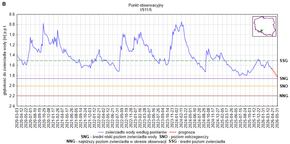
Rys. 12. Prognoza dotycząca stanu wód o zwierciadle swobodnym (gruntowych) na okres 01.05.2026–31.05.2026 r. – stacja hydrogeologiczna nr I/911/5 w miejscowości Wrzoski (woj. opolskie). A – prognoza przy założeniu scenariusza A; B – prognoza przy założeniu scenariusza B
