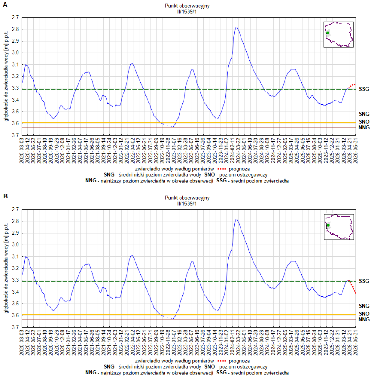
Rys. 6. Prognoza dotycząca stanu wód o zwierciadle swobodnym (gruntowych) na okres 01.05.2026–31.05.2026 r. – stacja hydrogeologiczna nr II/1539/1 w miejscowości Czartów (woj. lubuskie). A – prognoza przy założeniu scenariusza A; B – prognoza przy założeniu scenariusza B
