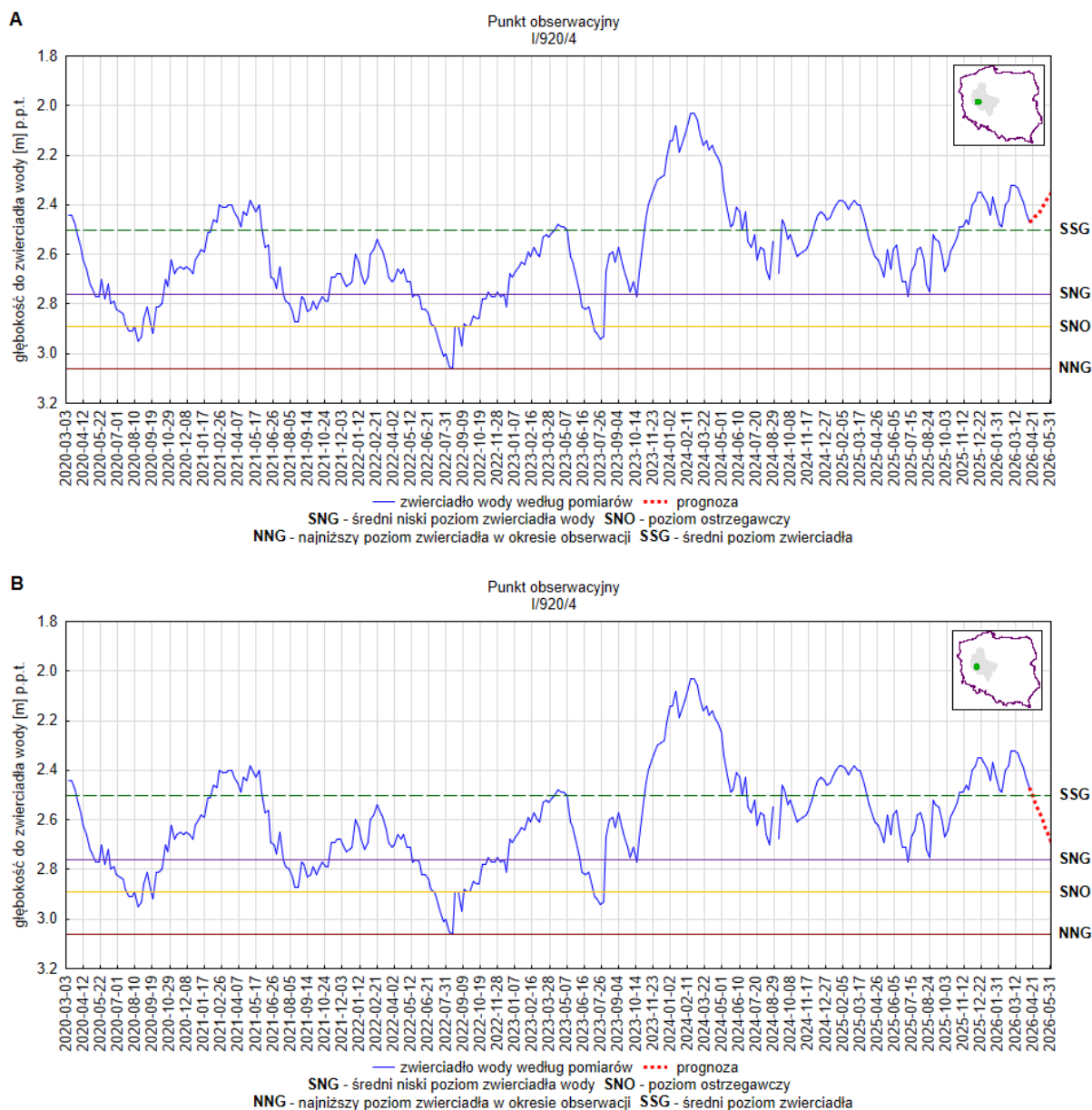
Rys. 22. Prognoza dotycząca stanu wód o zwierciadle swobodnym (gruntowych) na okres 01.05.2026–31.05.2026 r. – stacja hydrogeologiczna nr I/920/4 w miejscowości Sepno (woj. wielkopolskie). A – prognoza przy założeniu scenariusza A; B – prognoza przy założeniu scenariusza B
