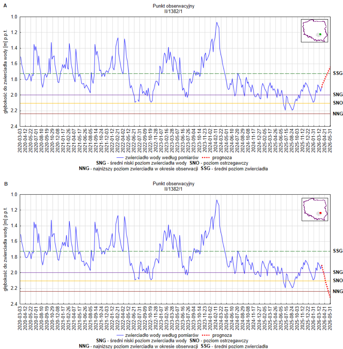
Rys. 19. Prognoza dotycząca stanu wód o zwierciadle swobodnym (gruntowych) na okres 01.05.2026–31.05.2026 r. – stacja hydrogeologiczna nr II/1382/1 w miejscowości Ostrowiec Świętokrzyski (woj. świętokrzyskie). A – prognoza przy założeniu scenariusza A; B – prognoza przy założeniu scenariusza B
