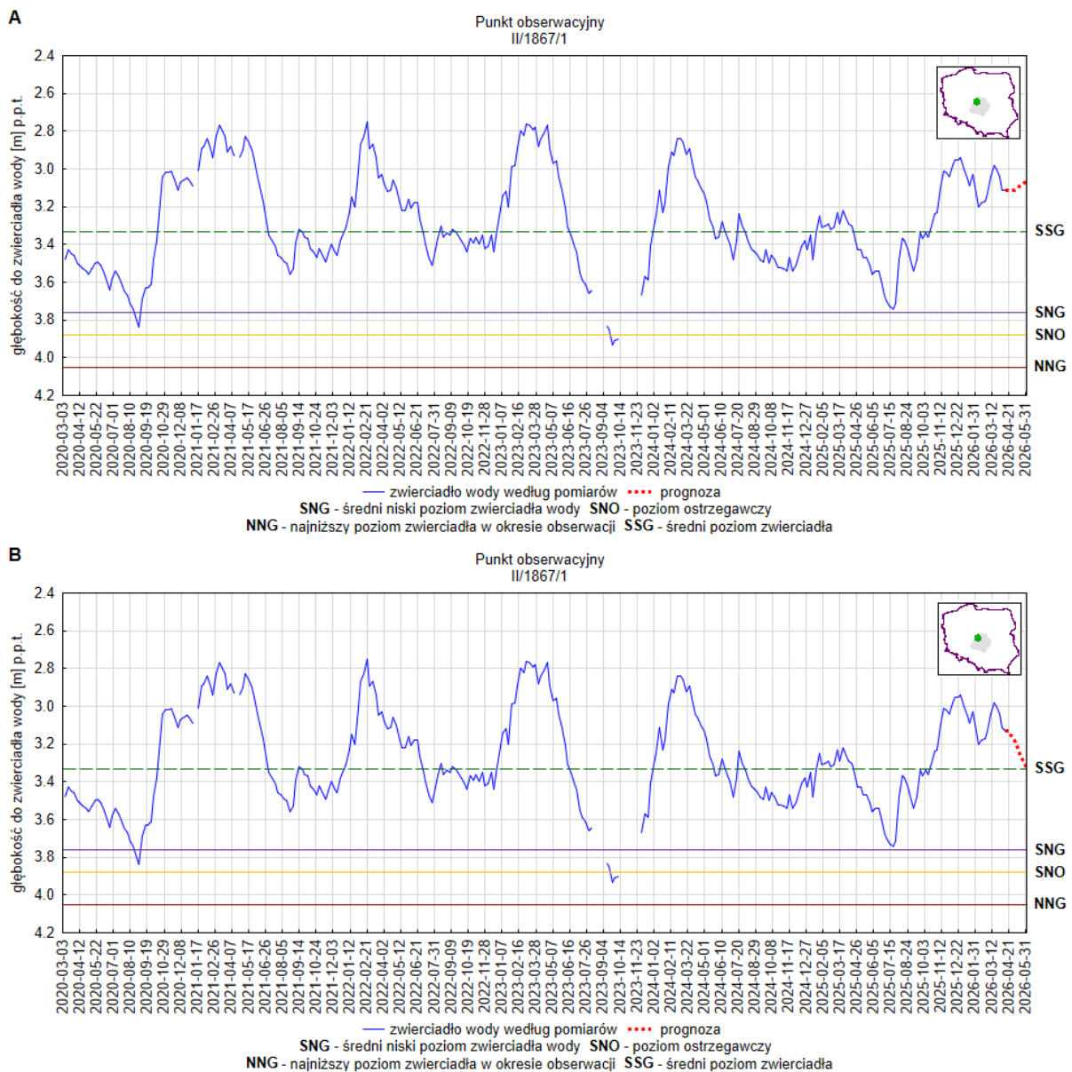
Rys. 8. Prognoza dotycząca stanu wód o zwierciadle swobodnym (gruntowych) na okres 01.05.2026–31.05.2026 r. – stacja hydrogeologiczna nr II/1867/1 w miejscowości Saków (woj. łódzkie). A – prognoza przy założeniu scenariusza A; B – prognoza przy założeniu scenariusza B
